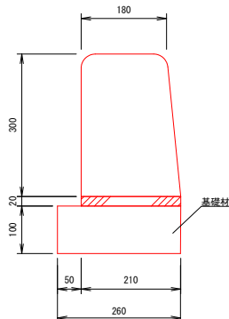
歩車道境界ブロックC S=1:10
