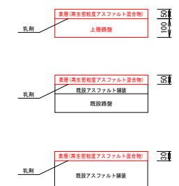
舗装標準断面図 S=1:20
