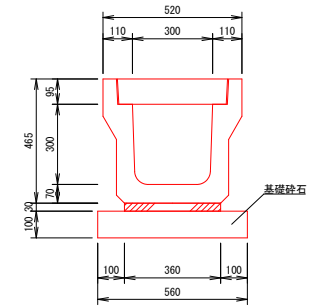
車線分離標 S=1:10
