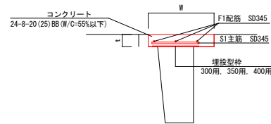
撤去しない埋設型枠
