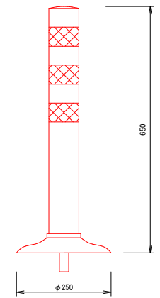
車線分離標 S=1:10
