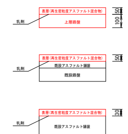
舗装標準断面図
