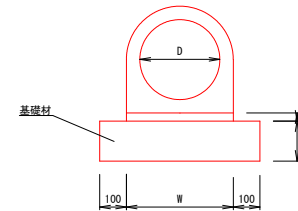
台付鉄筋コンクリート管
