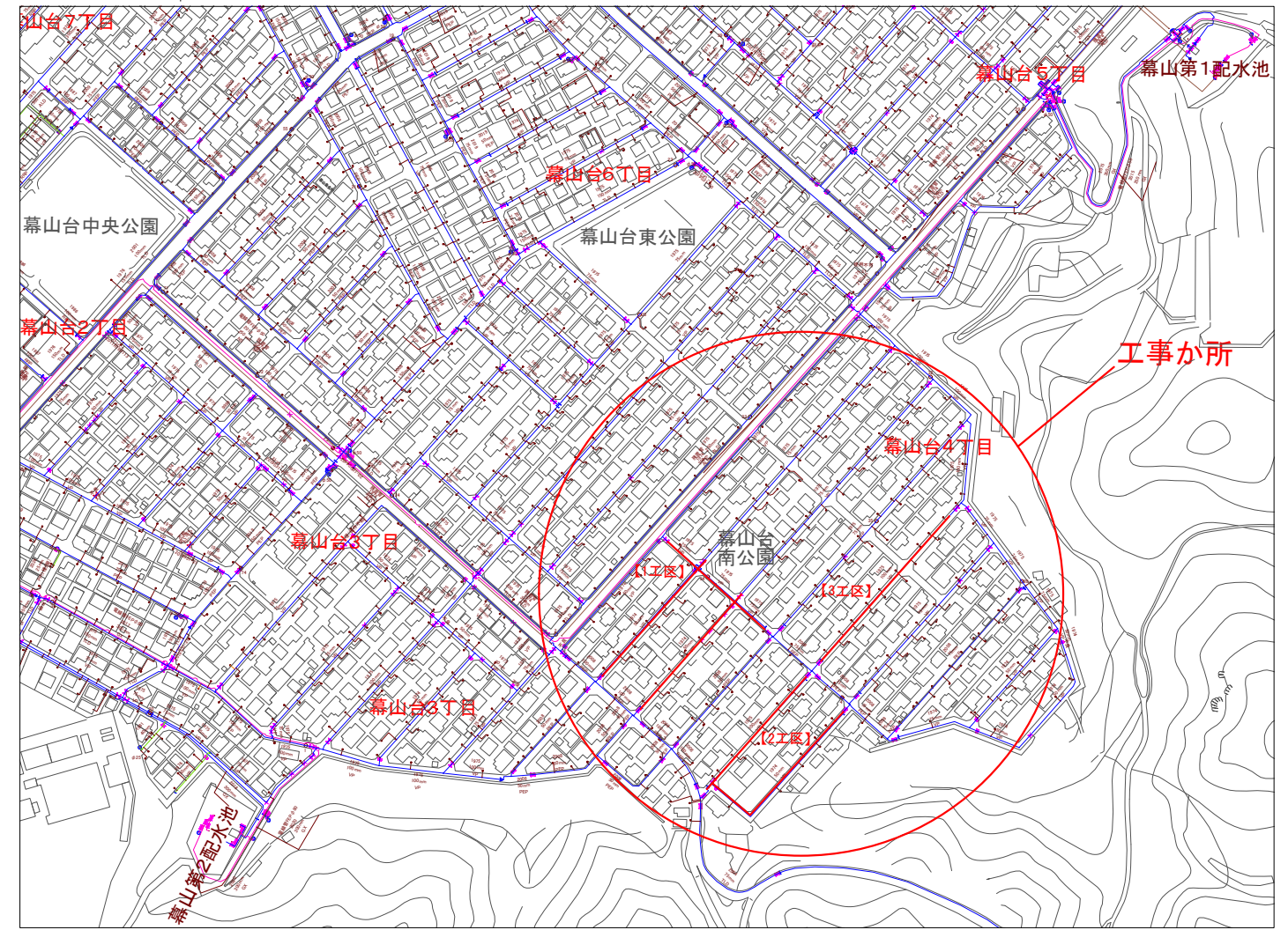
配管図 S=1/2500
