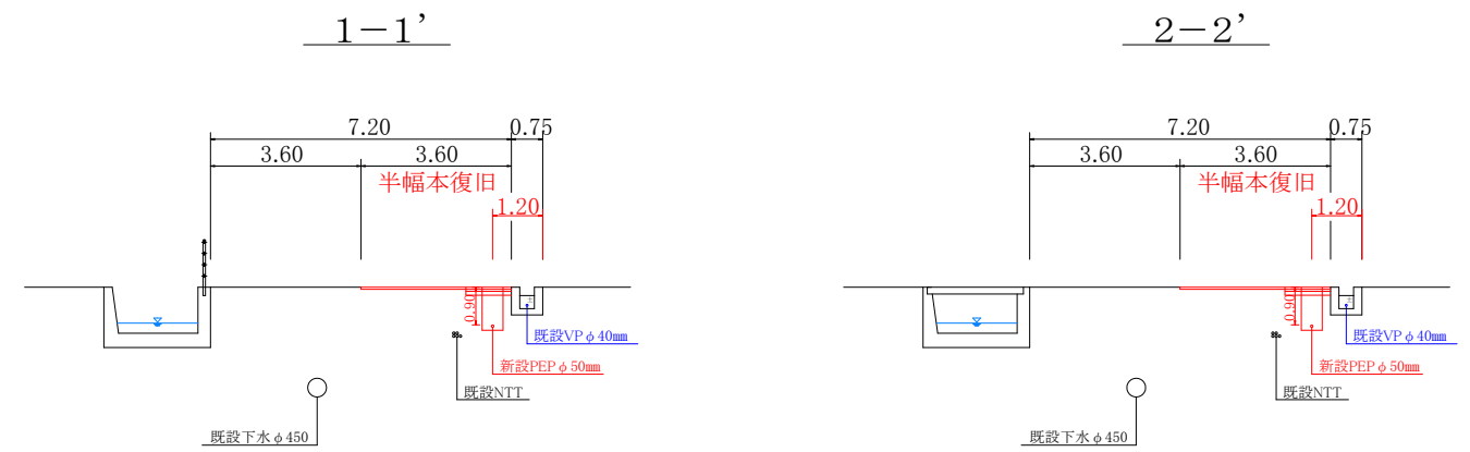
横断面図 S=1/100
