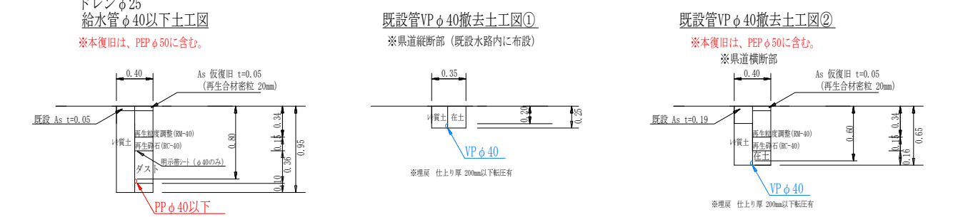
ドレンφ25 給水管φ40以下土工図
