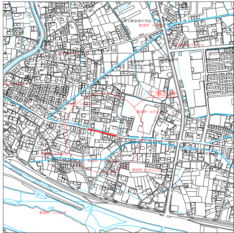
位置図 S=1/5000
