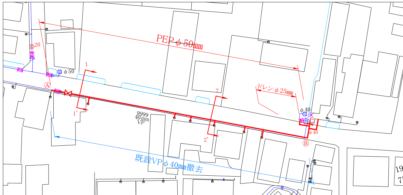
平面図 S=1/500
