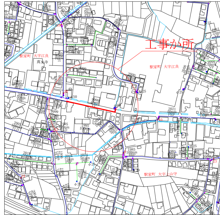
配管図 S=1/2500
