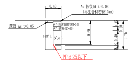
給水管φ25以下土工図
