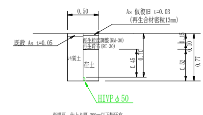
仮設管φ50土工図
