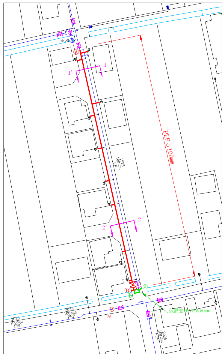
平面図 S=1/500
