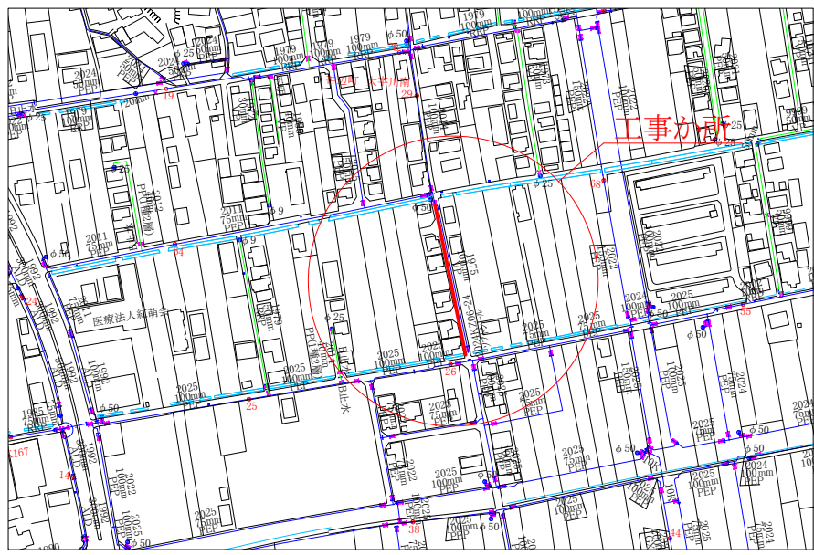
配管図 S=1/2500
