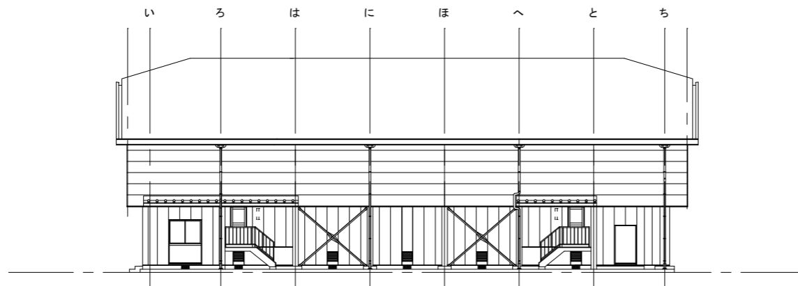
西側立面図 1:200
