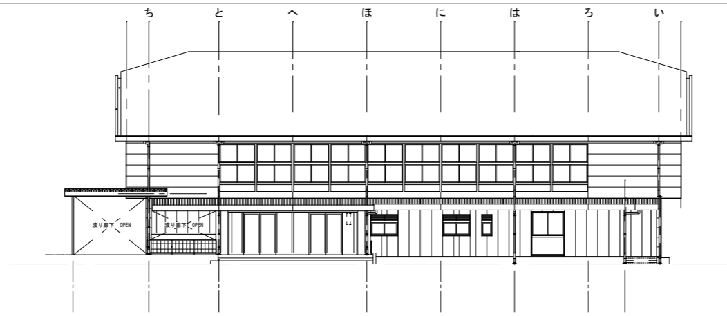
東側立面図 1:200
