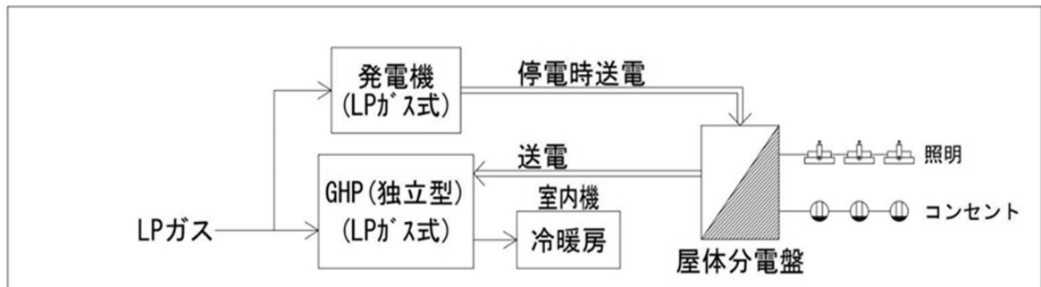
図1. 設備フロー図(福山中・高等学校、鞆の浦学園)
