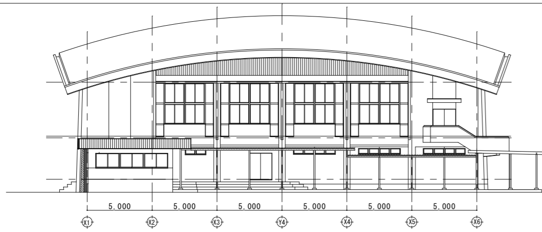
東側立面図 1:200
