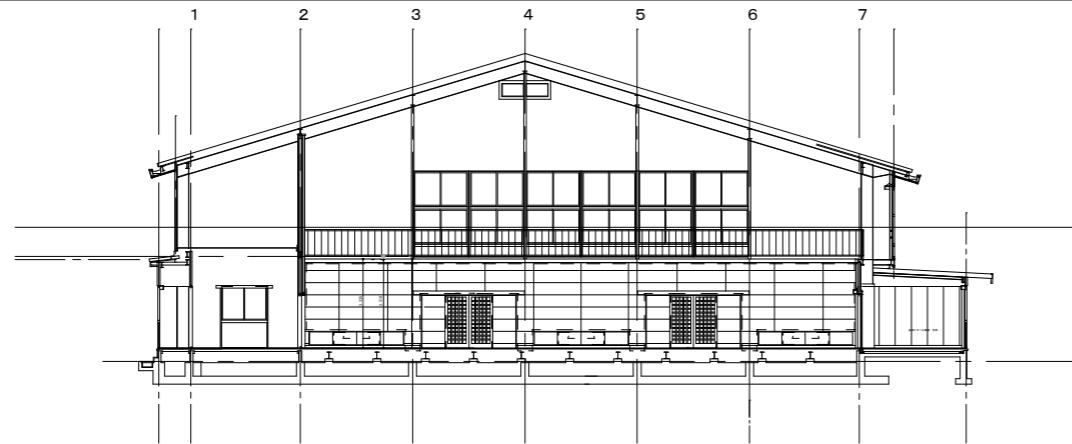
西側立面図 1:200
