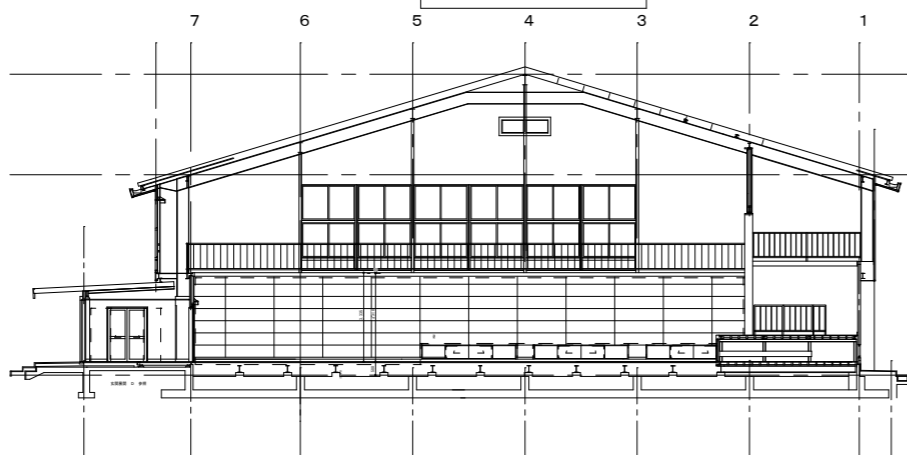
南面展開図 1:200
