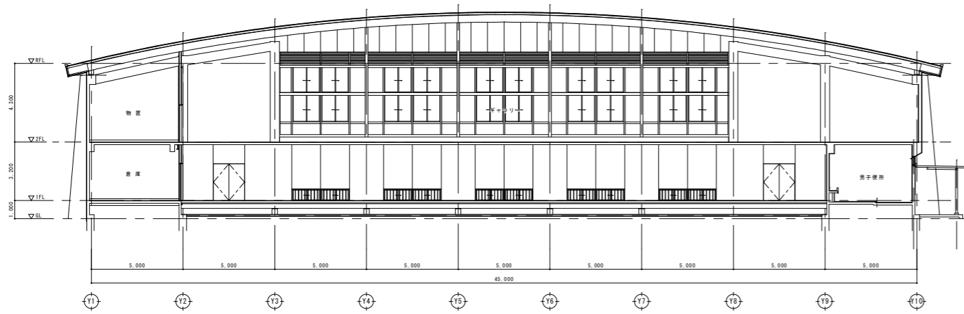
北面展開図 1:200
