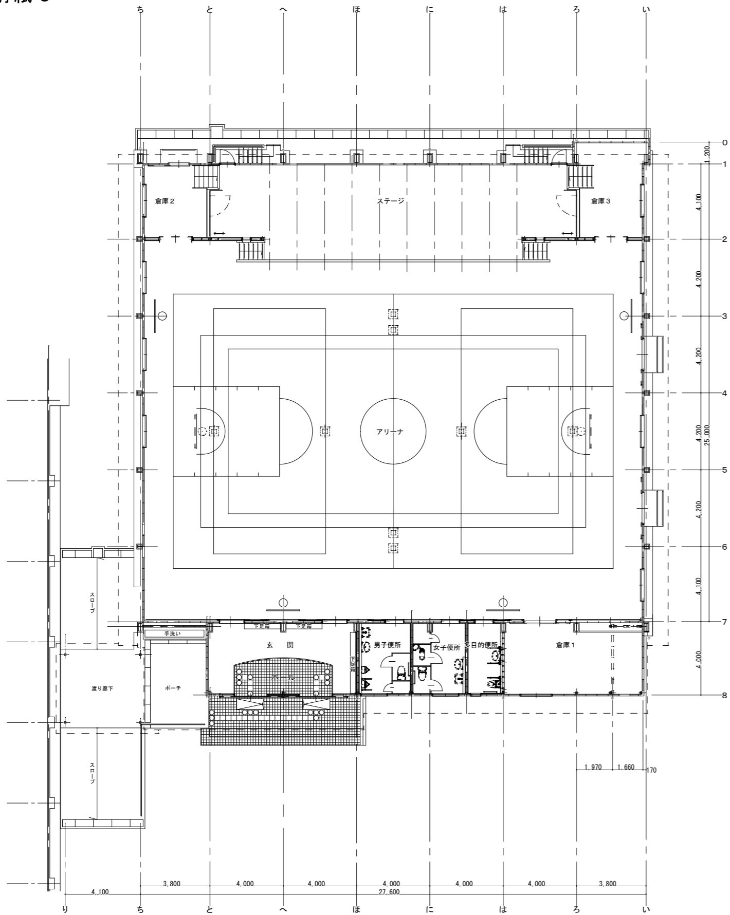
1階平面図 1:150
