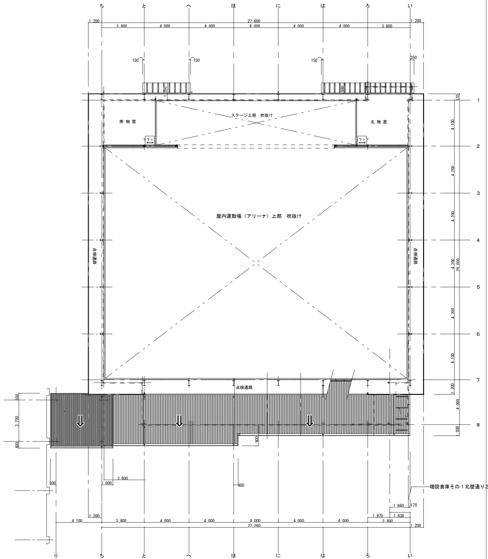
ギャラリー平面図 1:150
