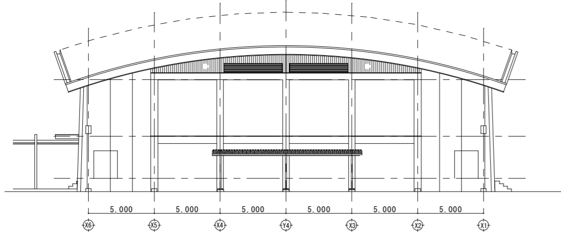
西側立面図 1:200
