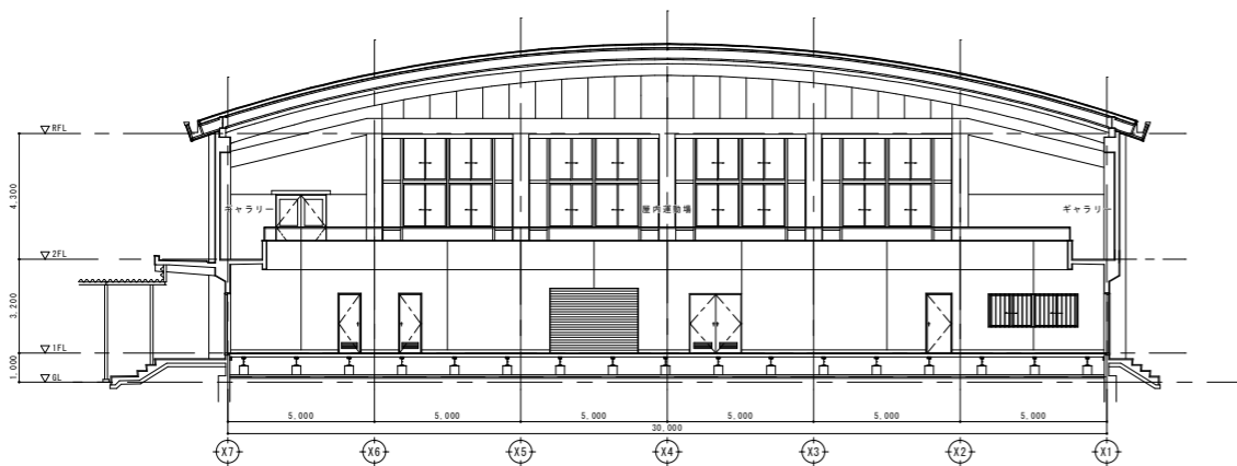
北面展開図 1:200
