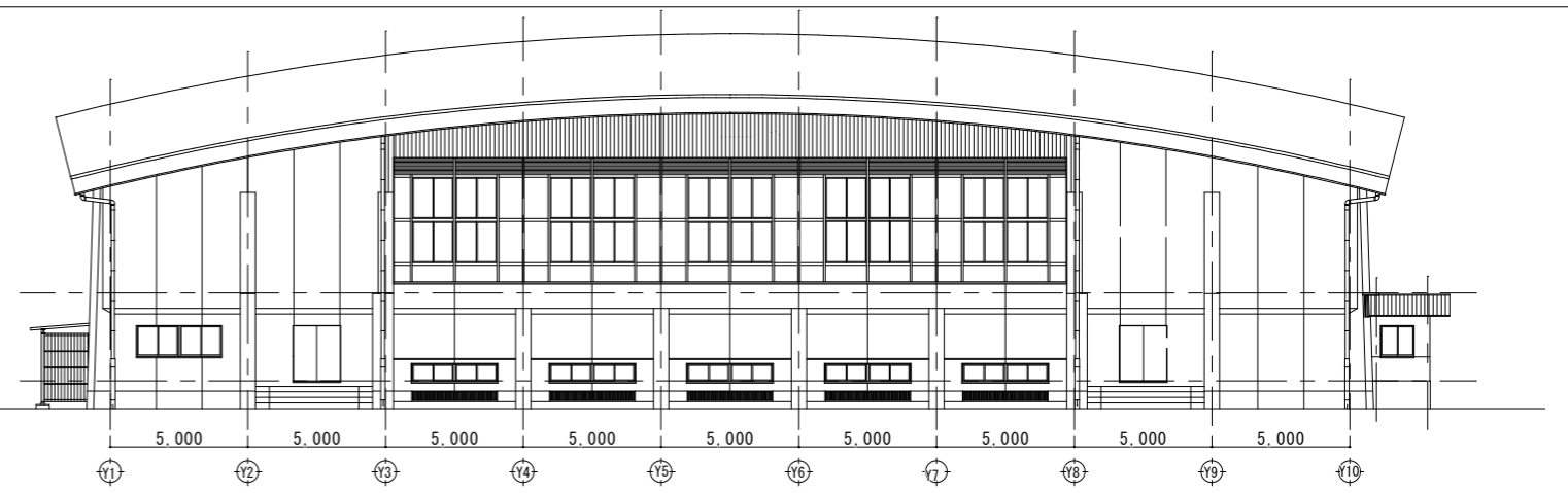
南側立面図 1:200
