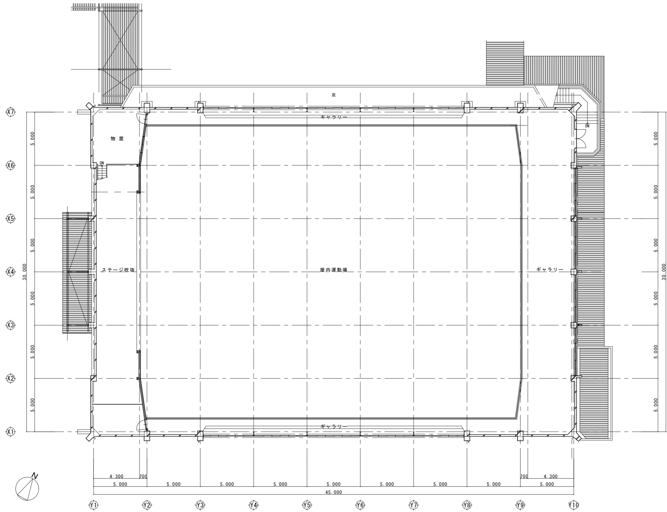
2階平面図 1:150
