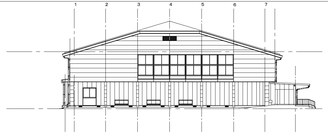
南側立面図 1:200
