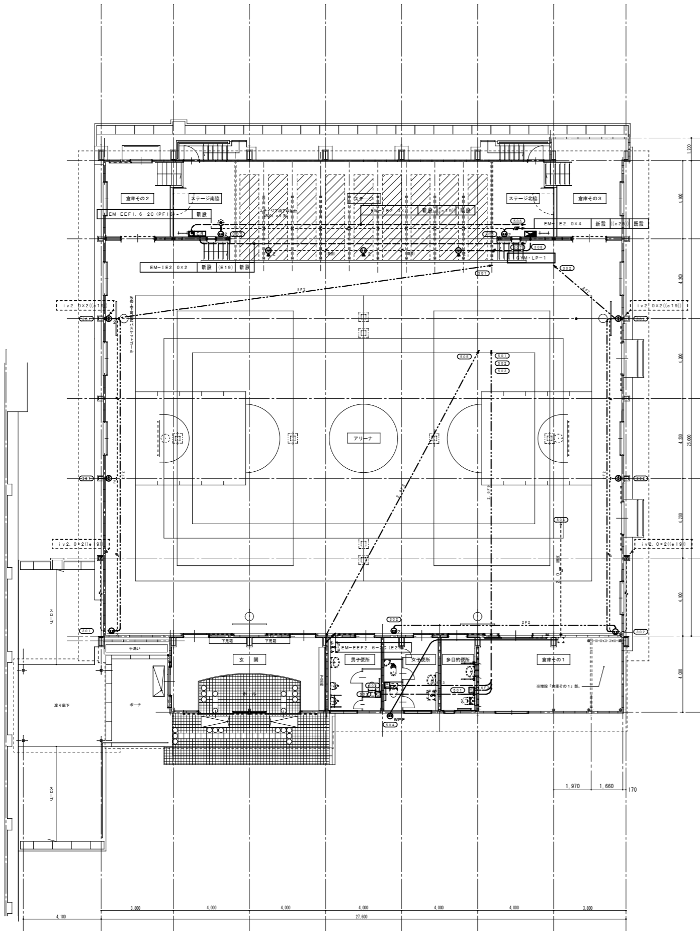
1階平面図 (コンセント設備図)
