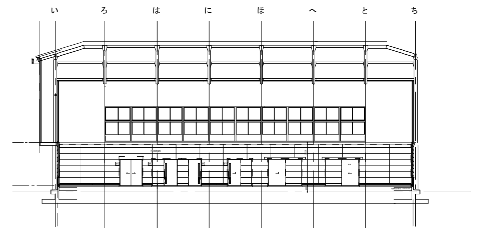
東面展開図 1:200
