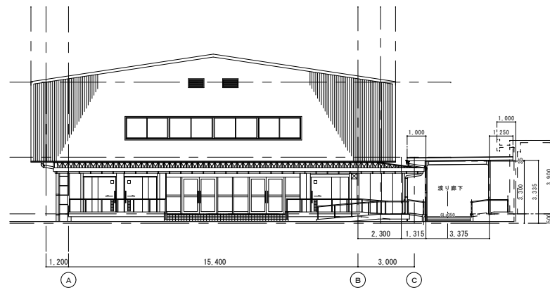
西側立面図 1:200
