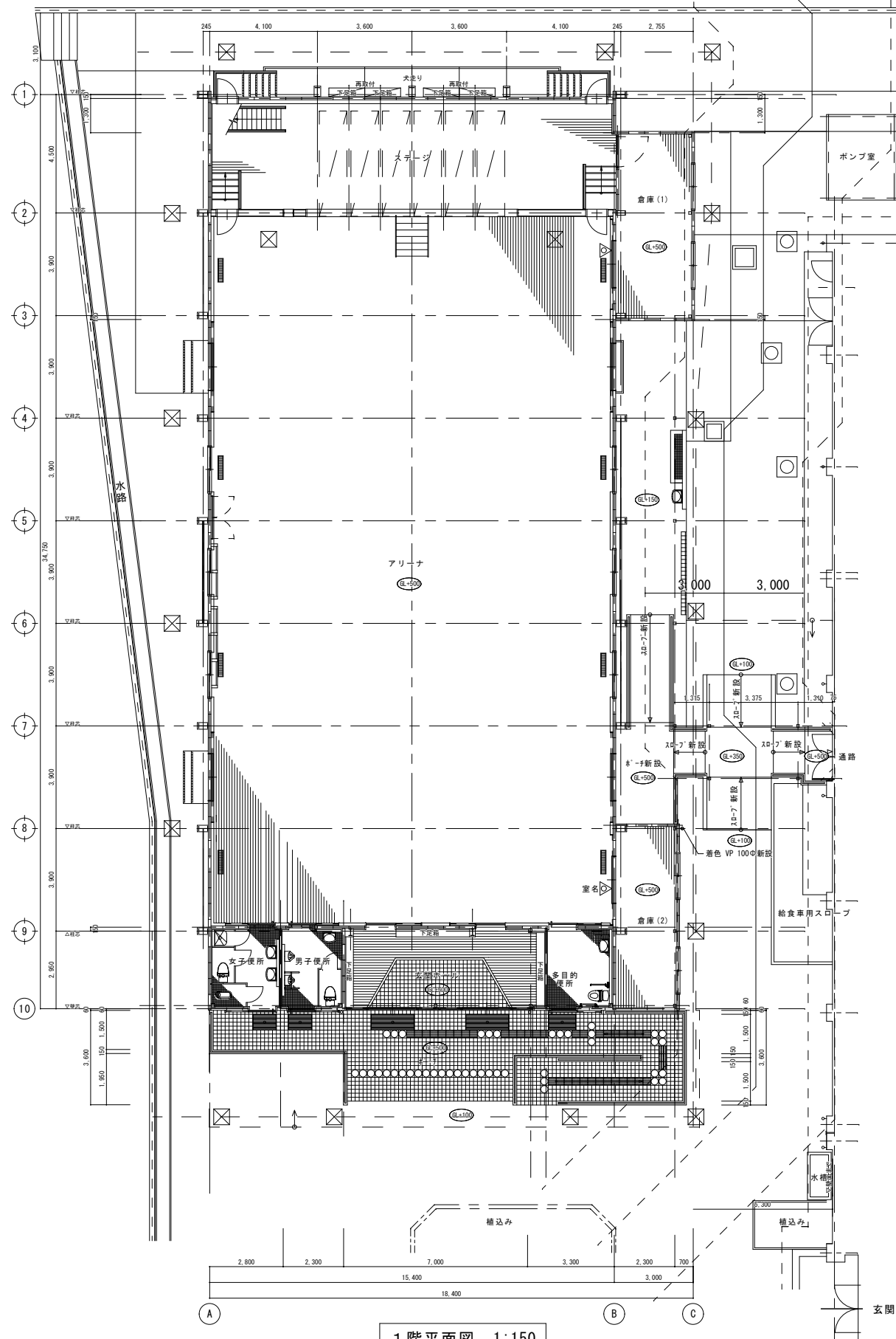
1階平面図 1:150
