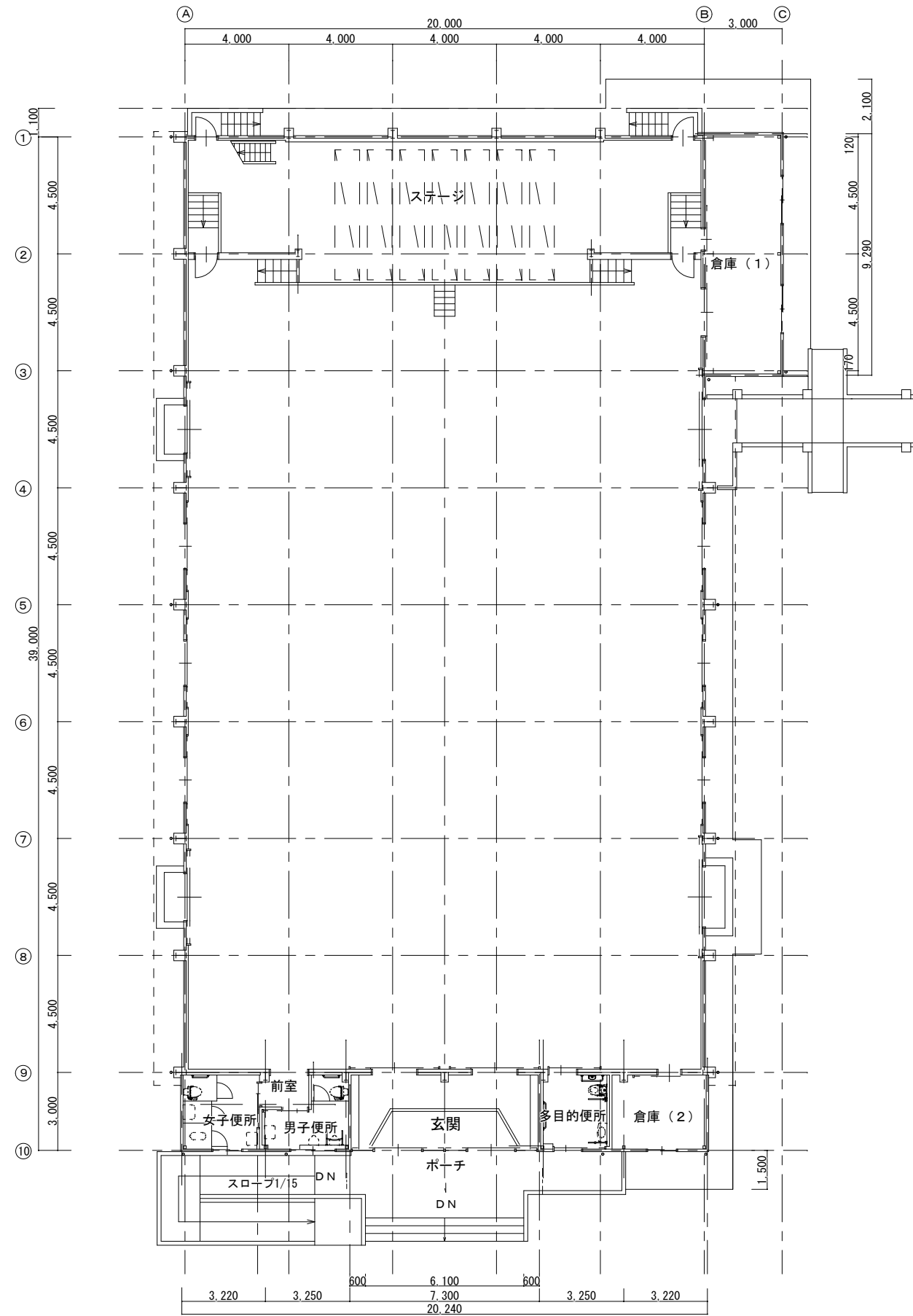
1階平面図 1:150
