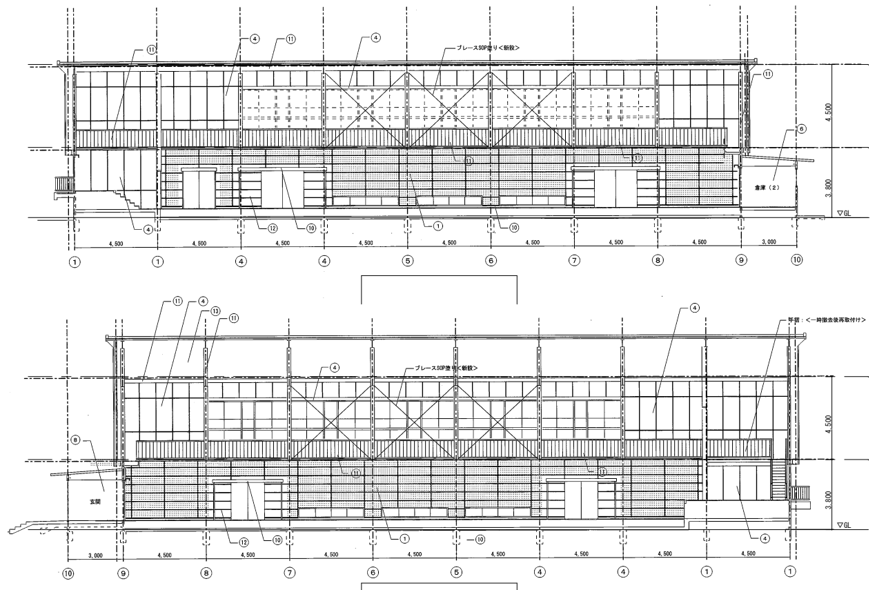
東面展開図 1:200
