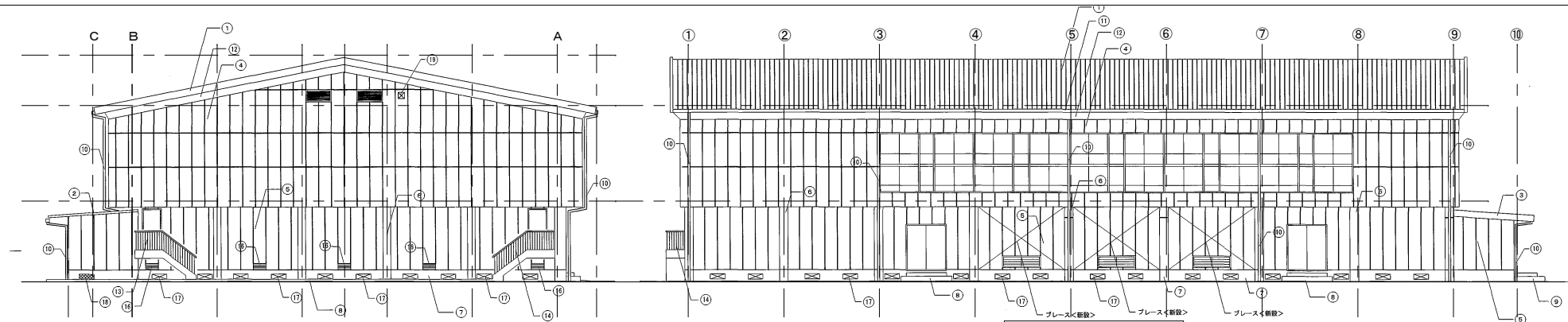
北側立面図 1:200
