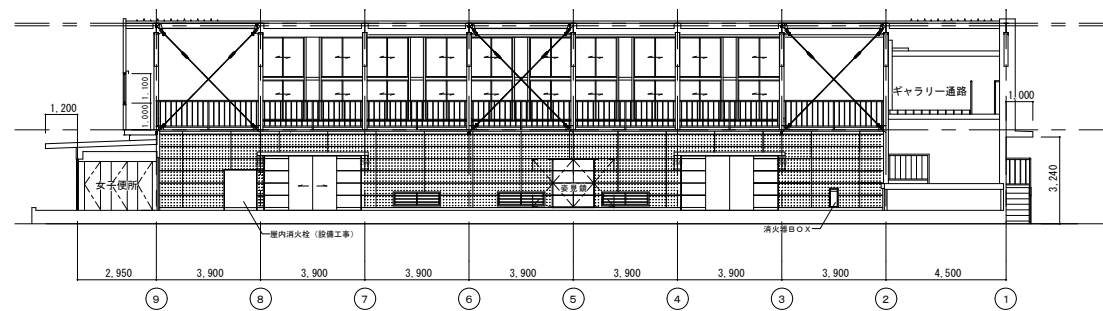
北面展開図 1:200
