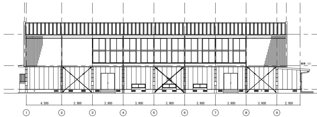
北側立面図 1:200
