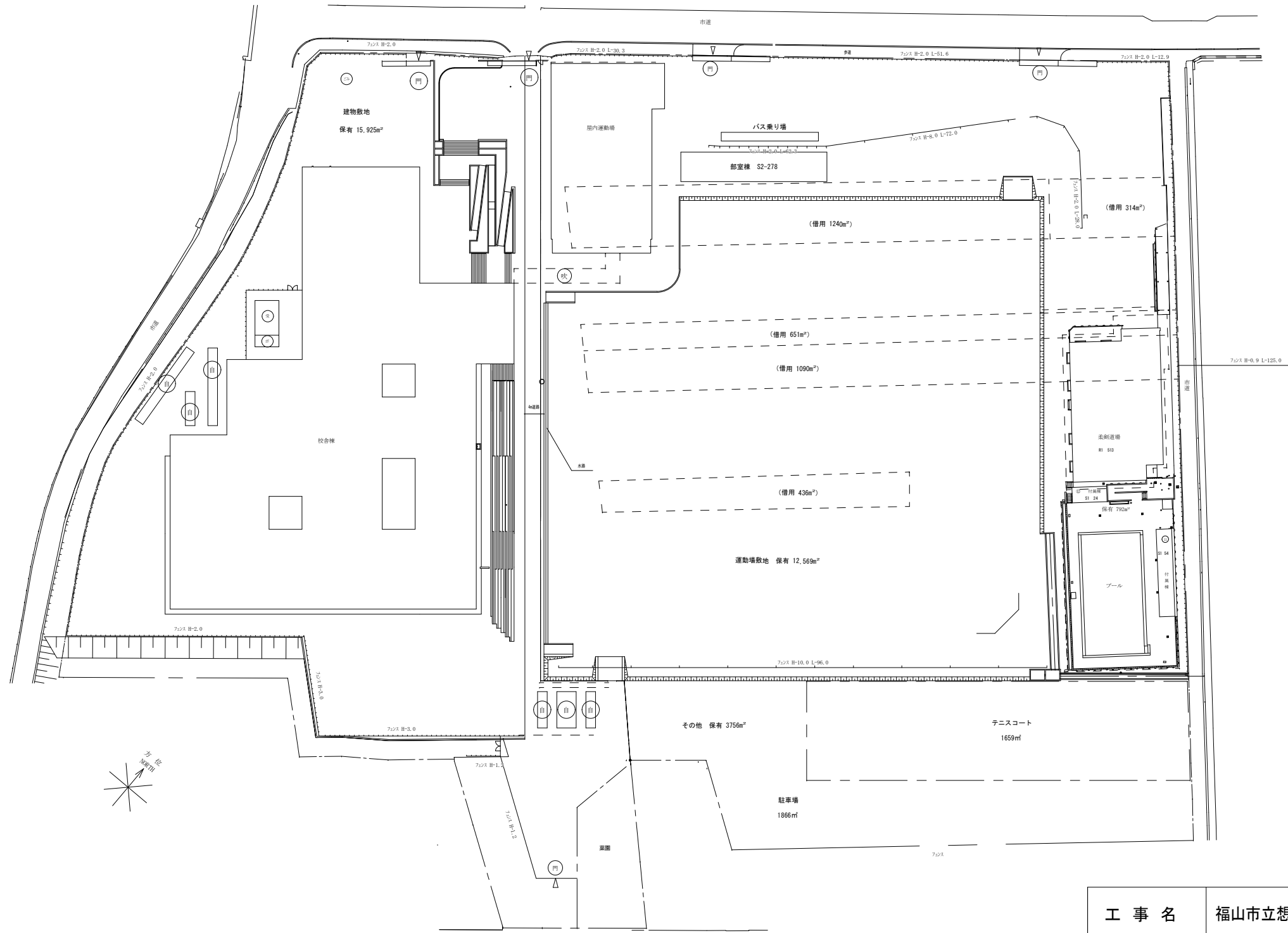
配置図 1:700
