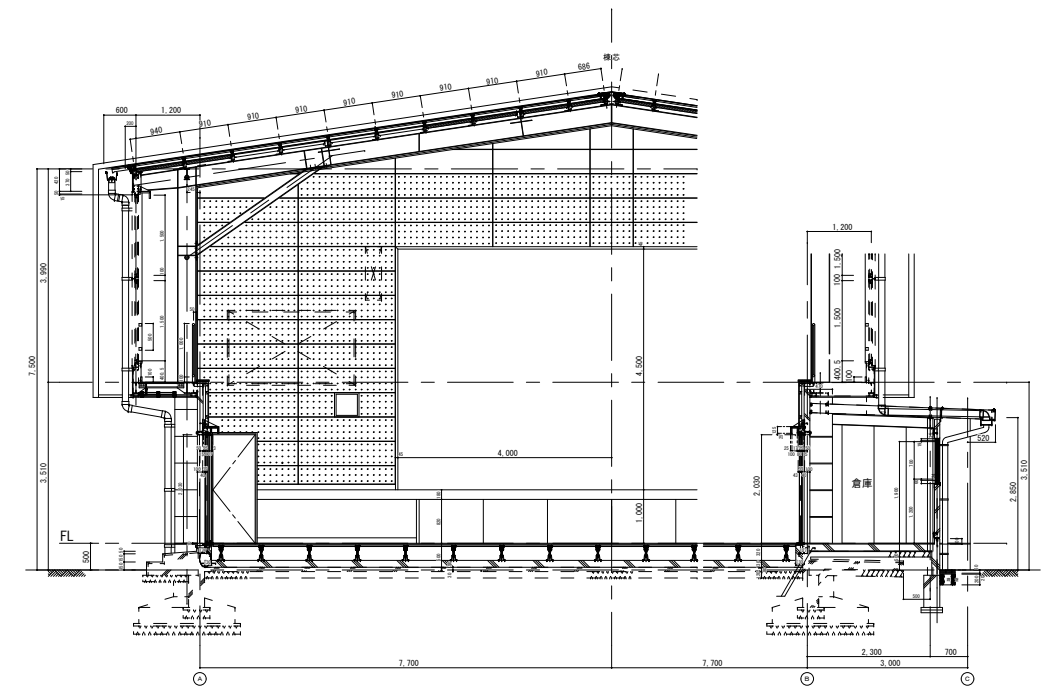
断面詳細図 1:100
