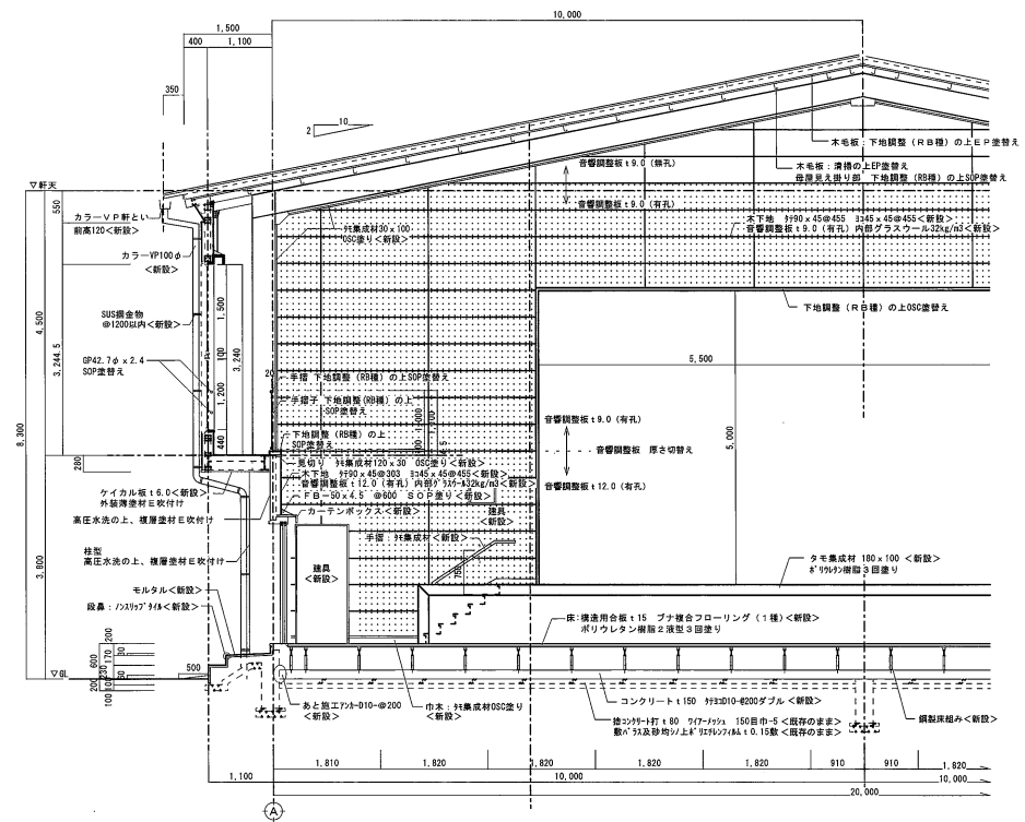
断面詳細図 1:100
