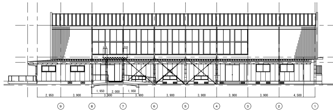
南側立面図 1:200
