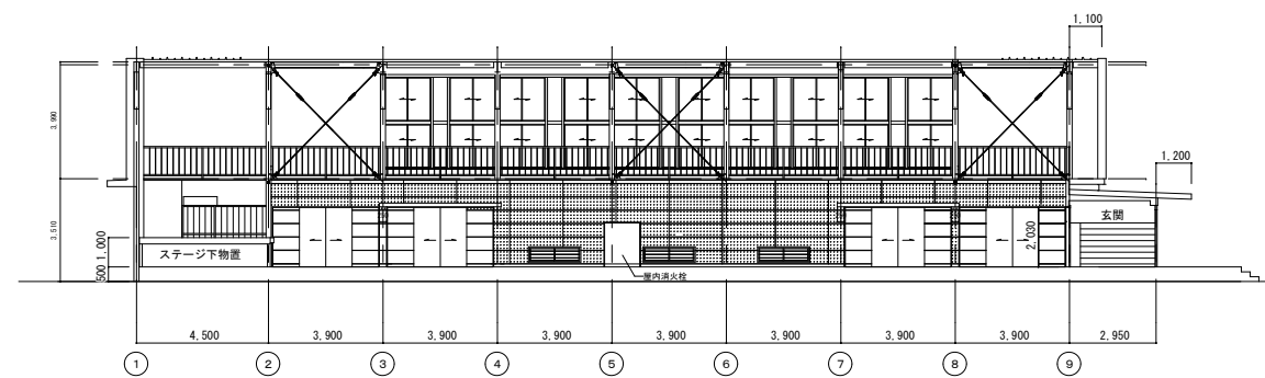
南面展開図 1:200
