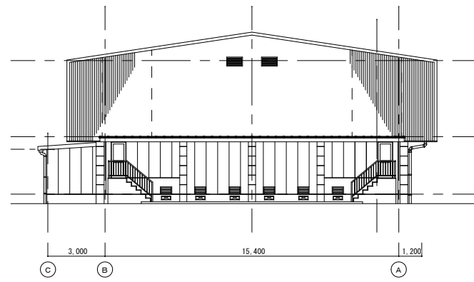
東側立面図 1:200
