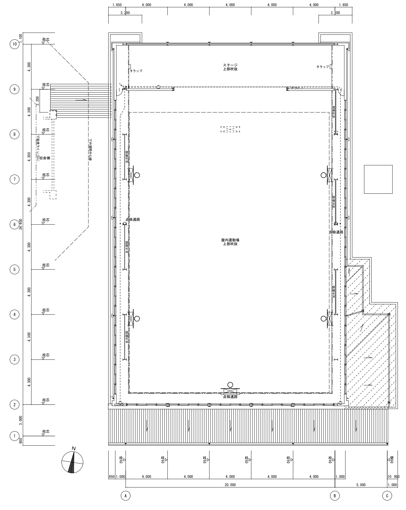
2階平面図 S=1:150
