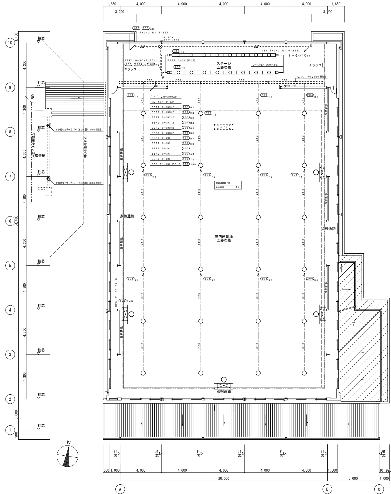
屋内運動場上部平面図 S=1:150
