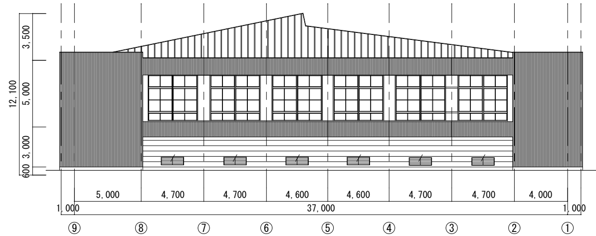
西側立面図 1:200
