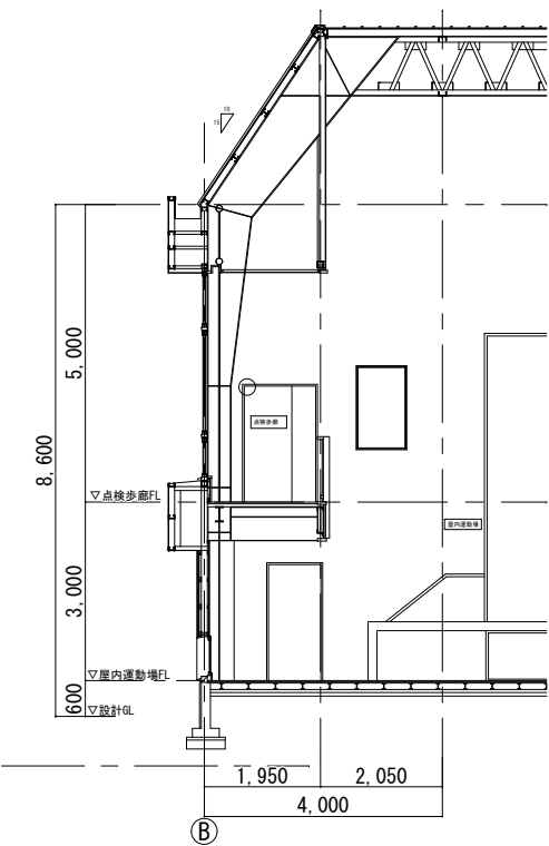
断面詳細図 1:100
