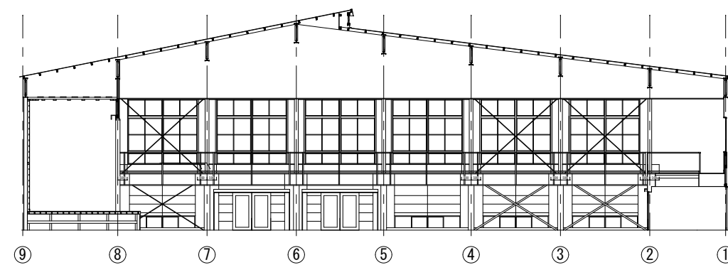
東面展開図 1:200
