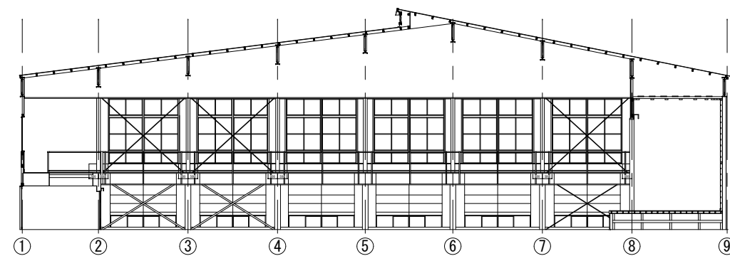
西面展開図 1:200
