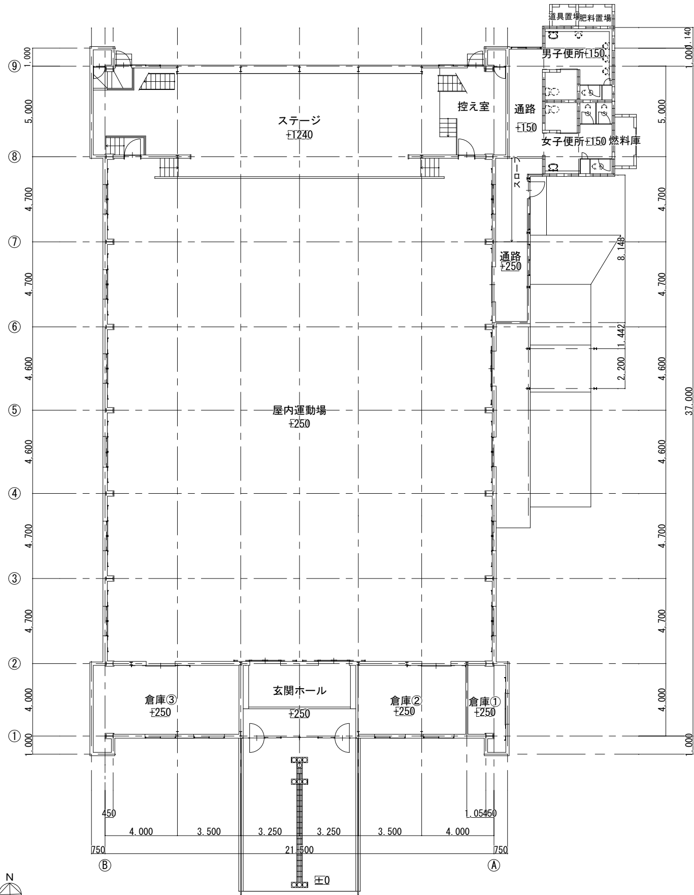
1階平面図 1:150
