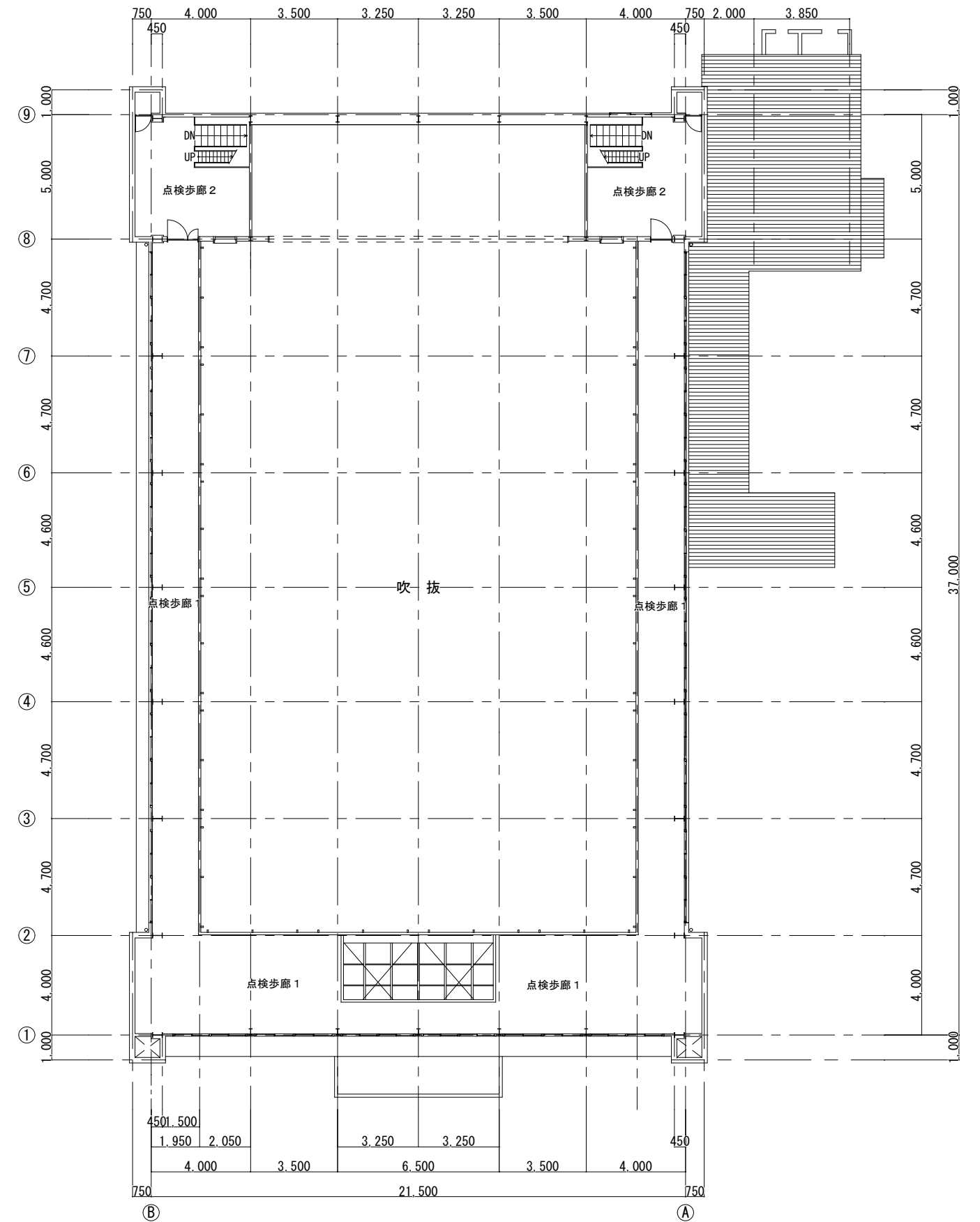
ギャラリー平面図 1:150
