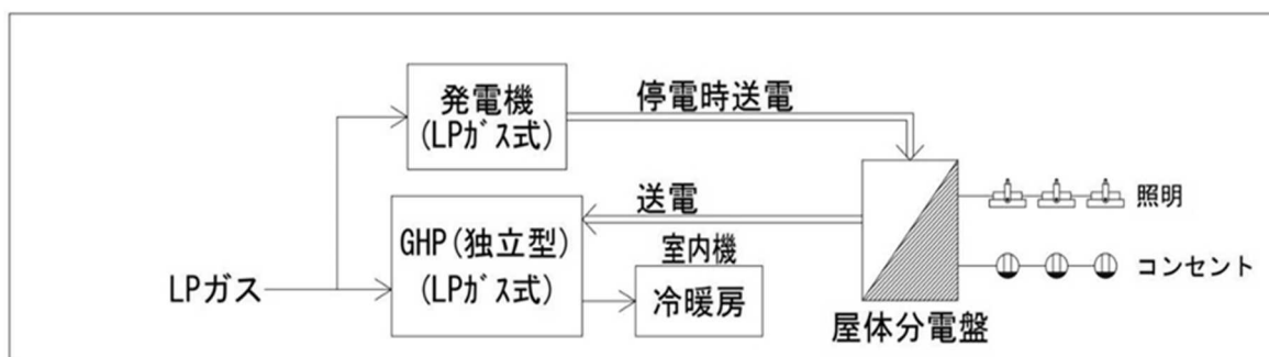
図1. 設備フロー図(宜山小、新市小)
