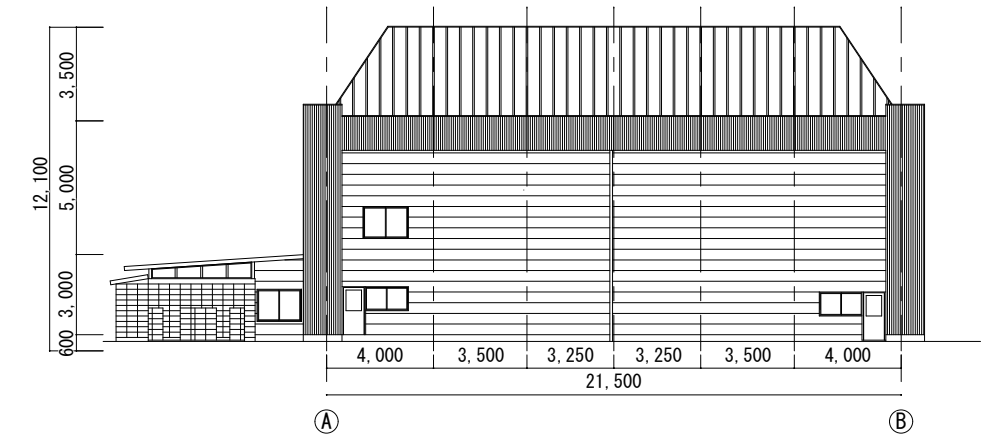
南側立面図 1:200
