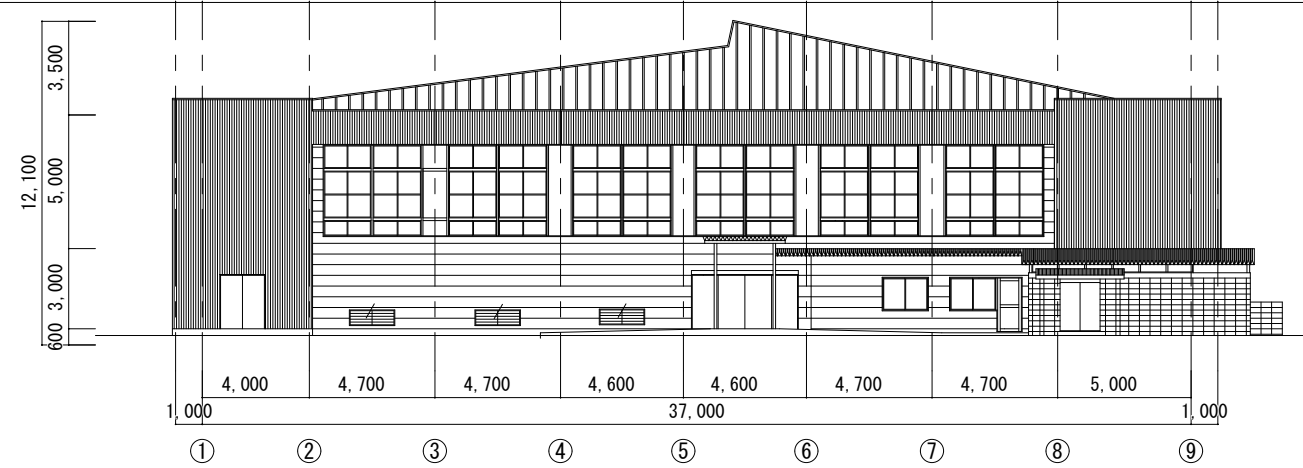
東側立面図 1:200
