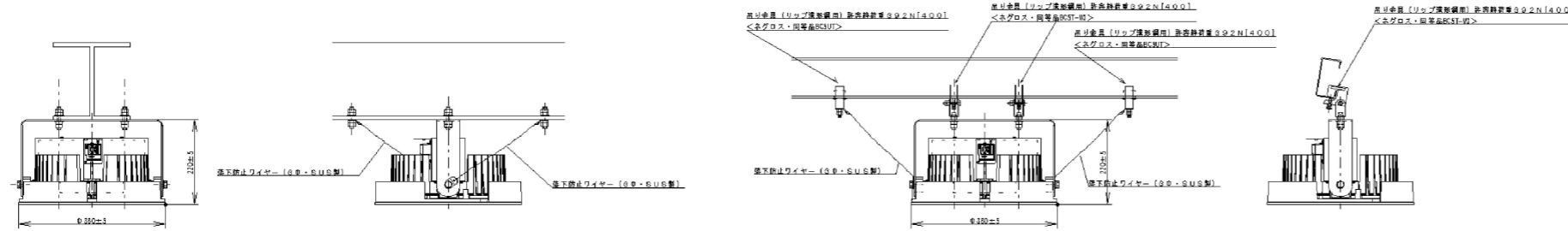
灯具取付要領図 S=1/10
