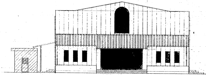
西側立面図 1:200
