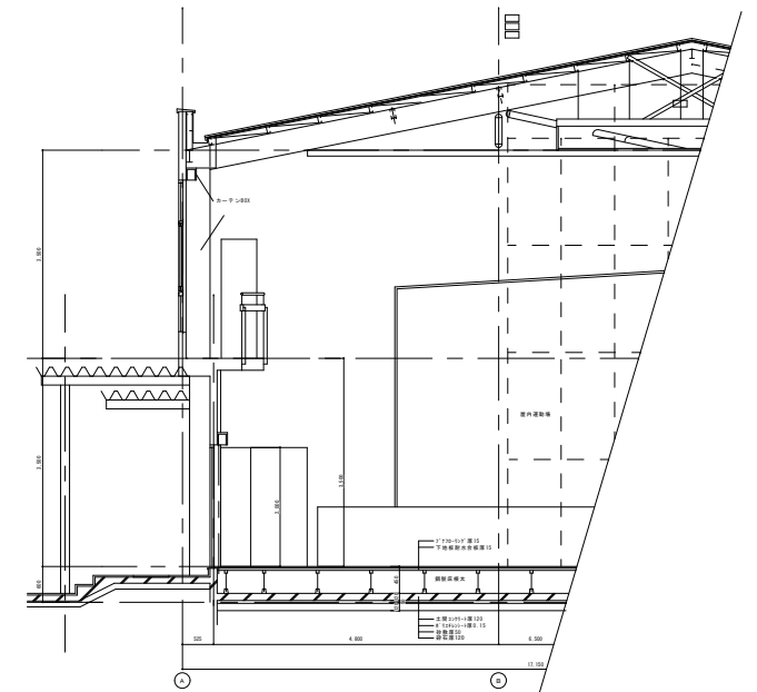
断面詳細図 1:100
