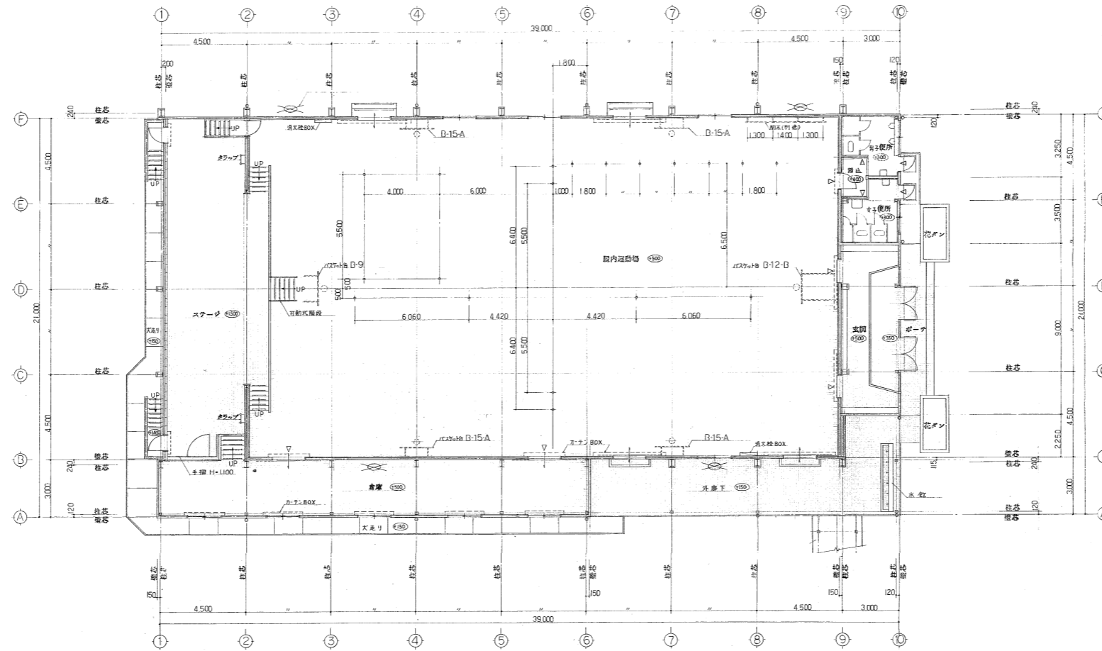
1階平面図 1:200
