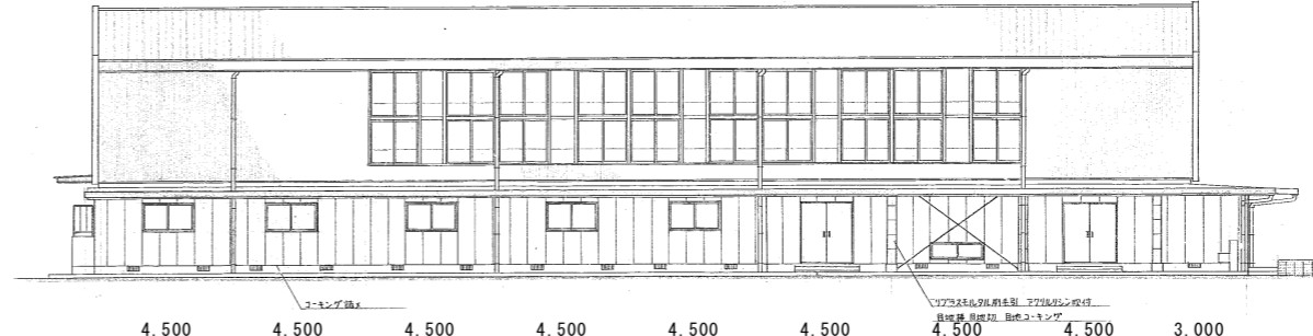
南側立面図 1:200
