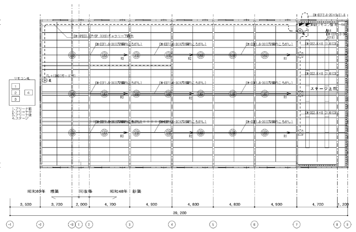
照明器具配置図・配線図 S=1/150
