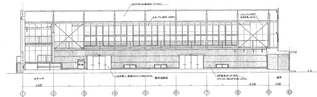
南面展開図 1:200
