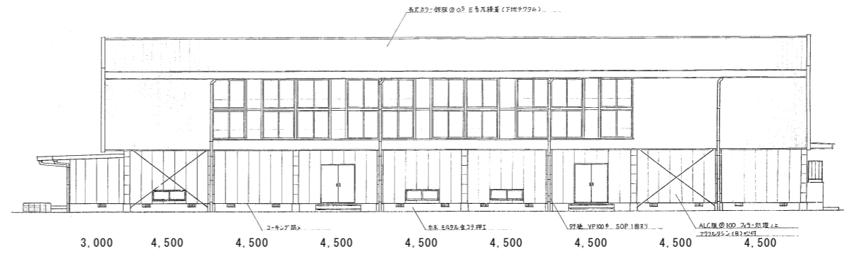
北側立面図 1:200
