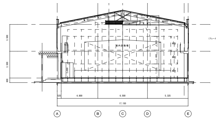
西面展開図 1:200
