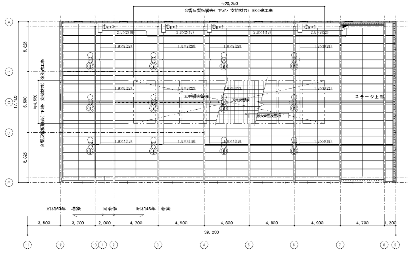
既存照明器具・配線・配管・撤去図 S=1/150
