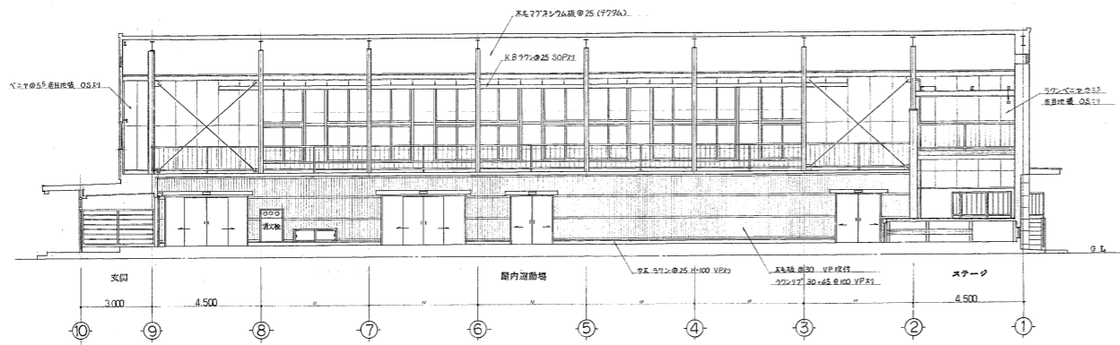
北面展開図 1:200
