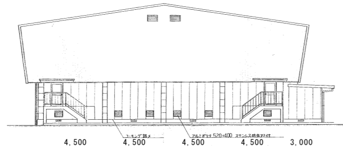
西側立面図 1:200
