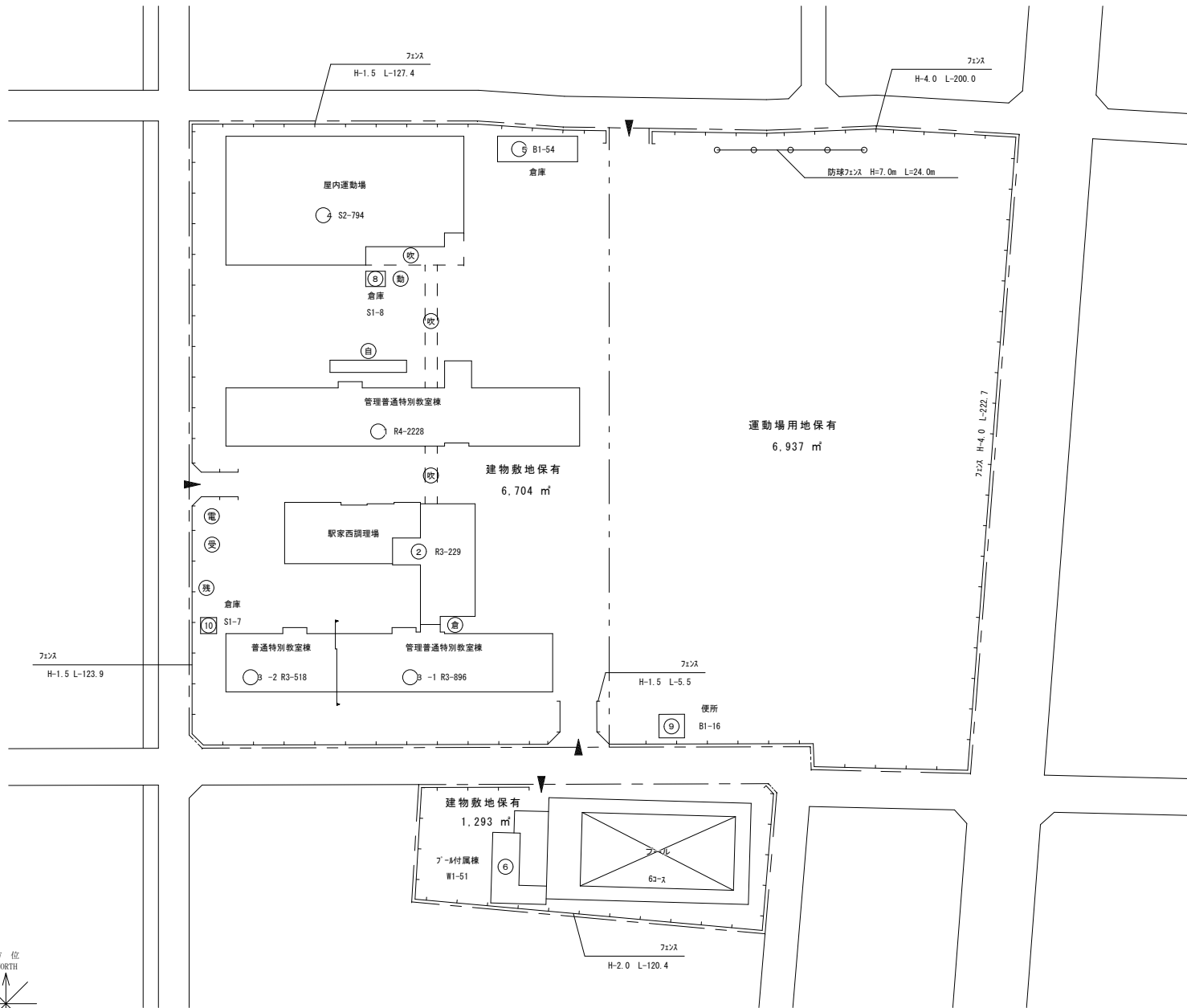
配置図 1:700
