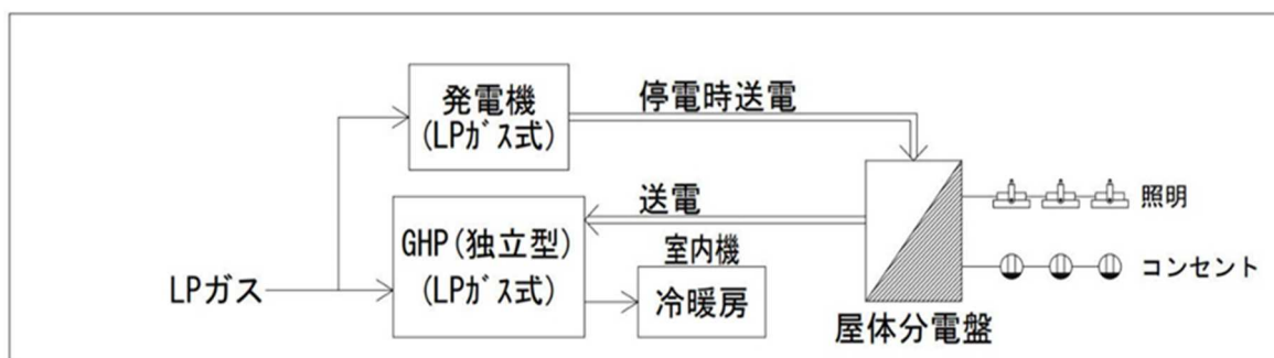
図1. 設備フロー図(駅家西小、道上小)
