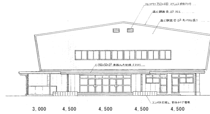
東側立面図 1:200
