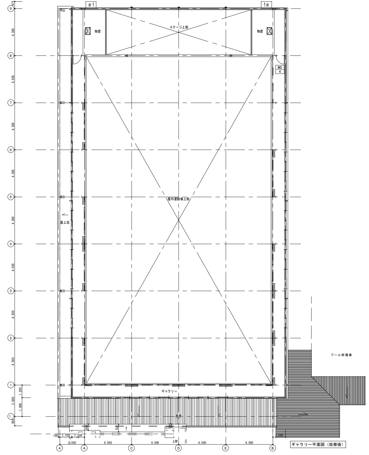
ギャラリー平面図 1:150
