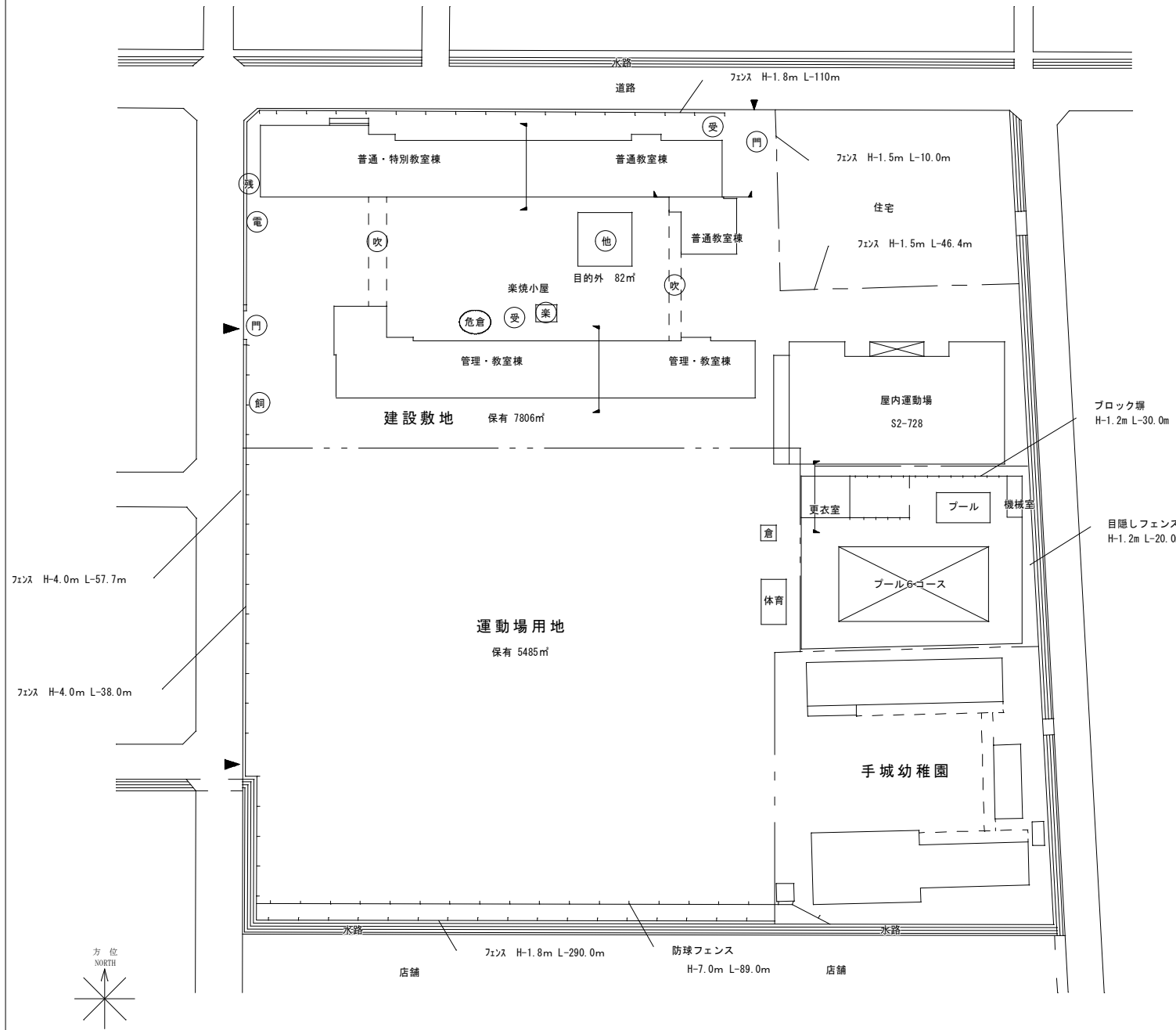
配置図 1:700
