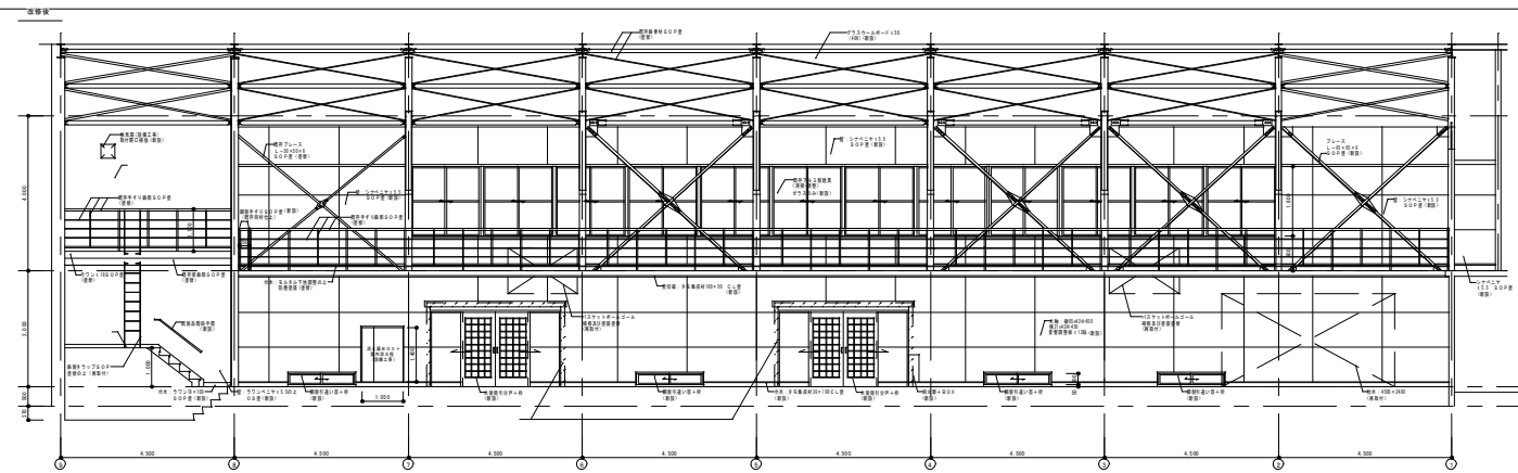
東側立面図 1:150
