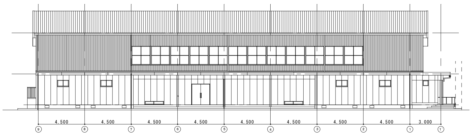
北側立面図 1:150
