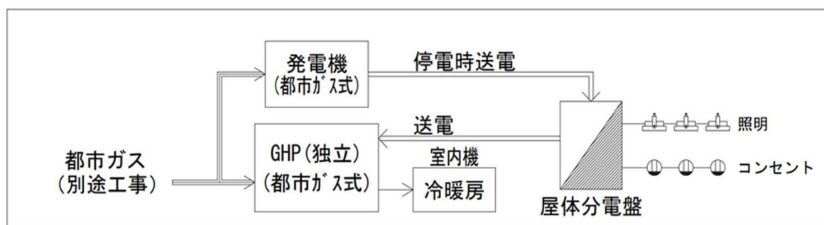
図1. 設備フロー図(城東中学校、手城小学校)
