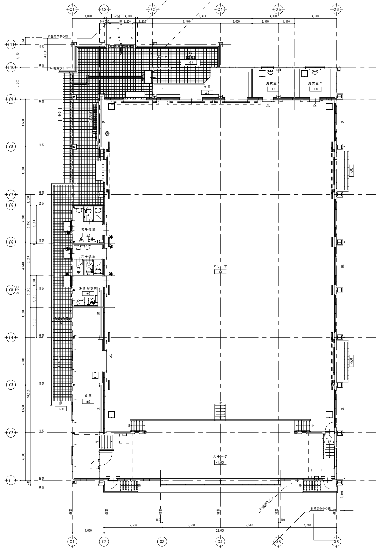
1階平面図 1:150
