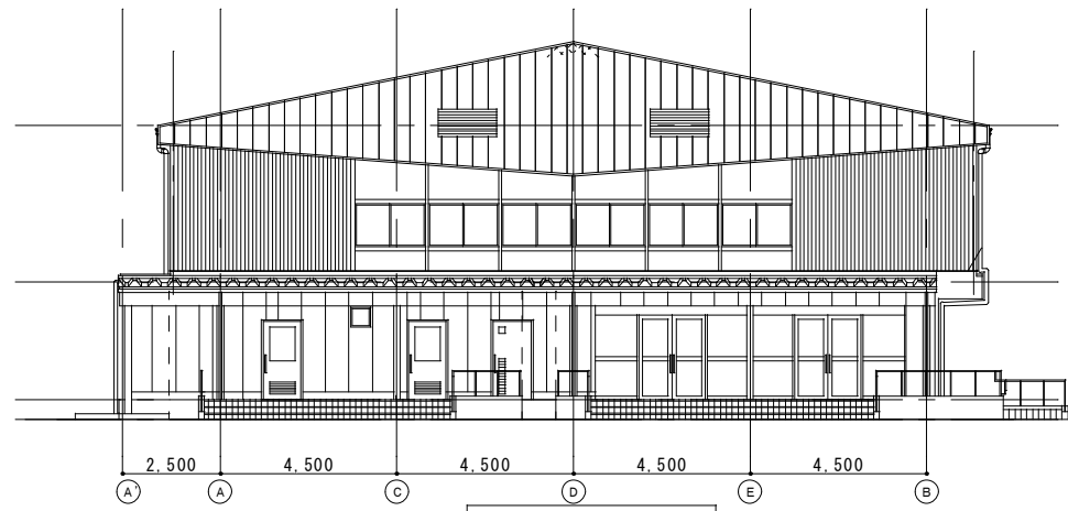
西側立面図 1:150
