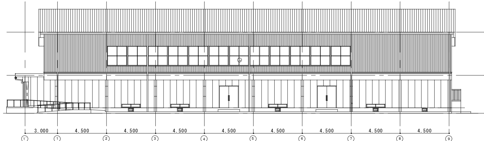
南側立面図 1:150
