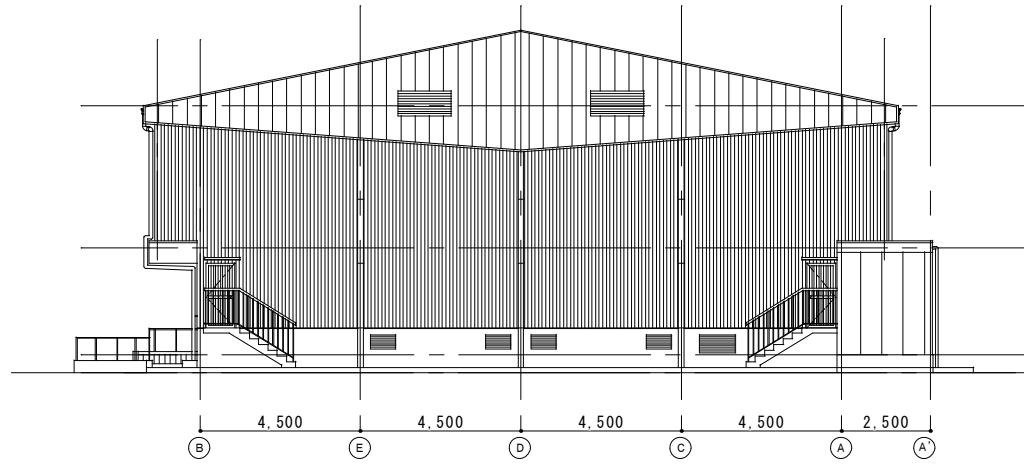
東側立面図 1:150
