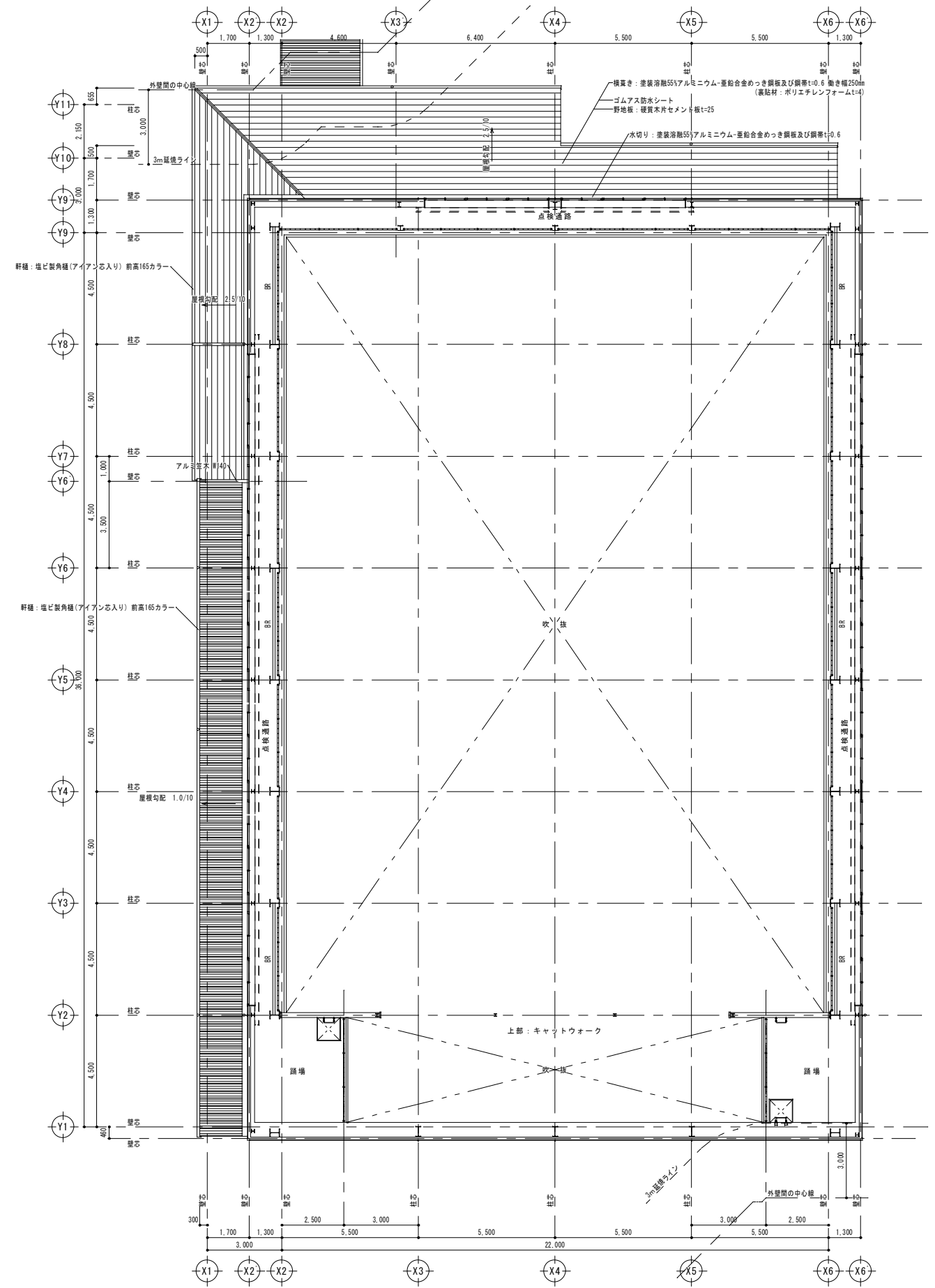
ギャラリー平面図 1:150
