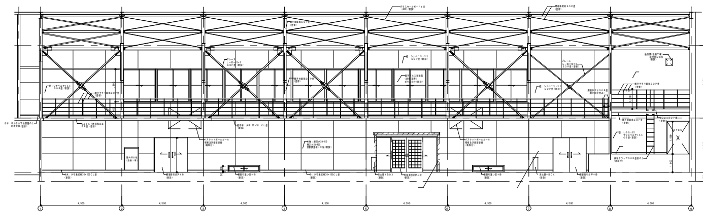
東面展開図 1:200
