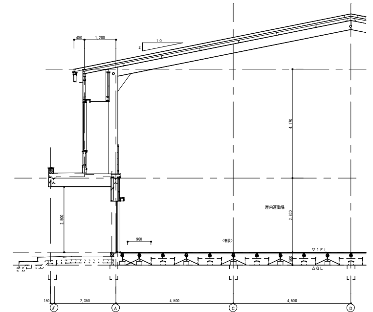
断面詳細図 1:100
