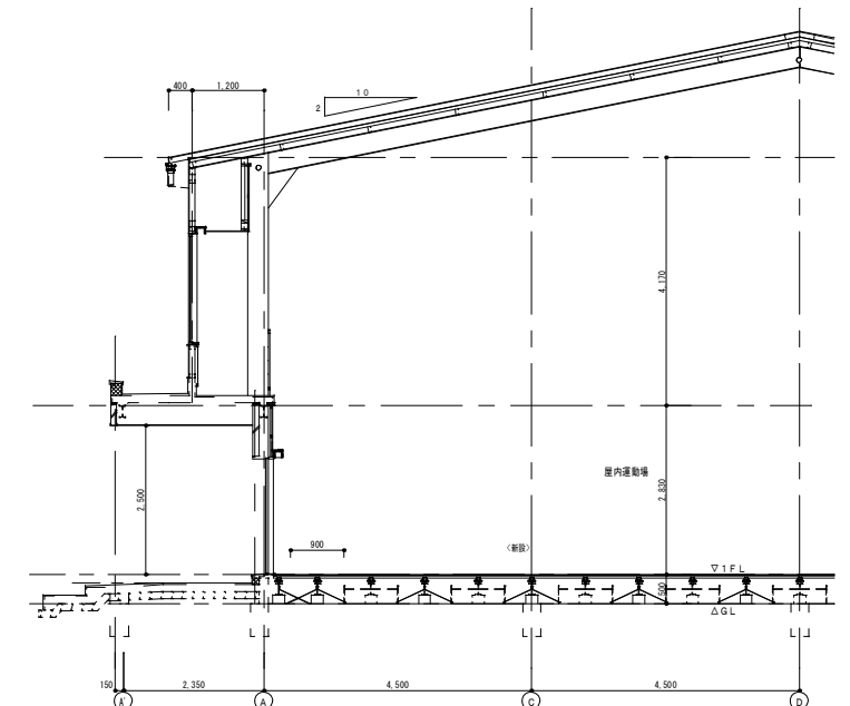
断面詳細図 1:100
