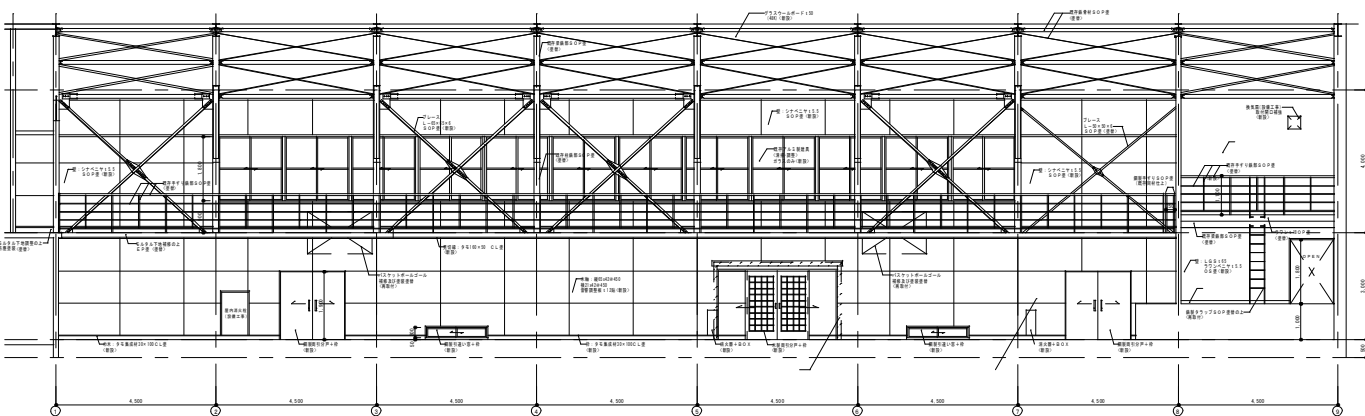
東面展開図 1:200
