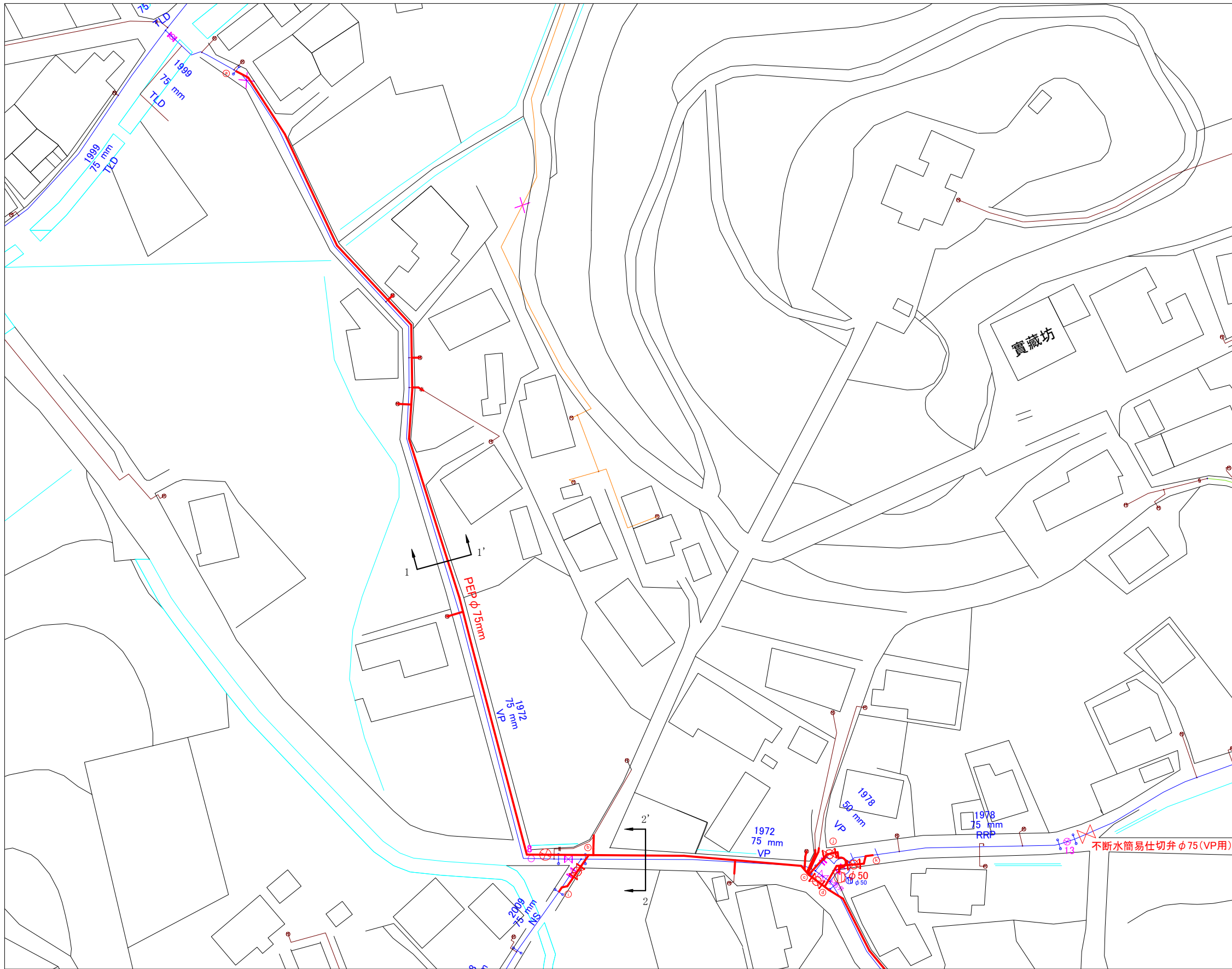
平面図(1) S=1/500
