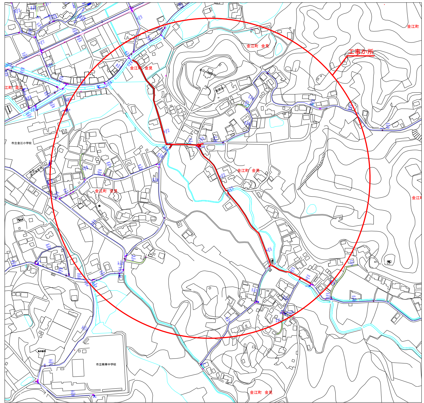
配管図 S=1/2500
