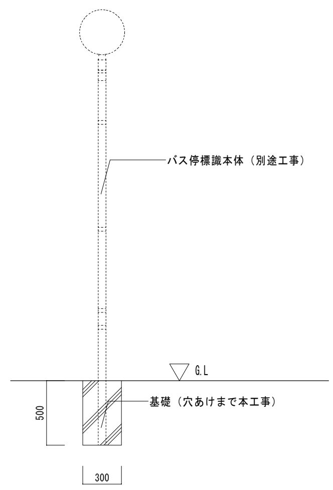
側面図
