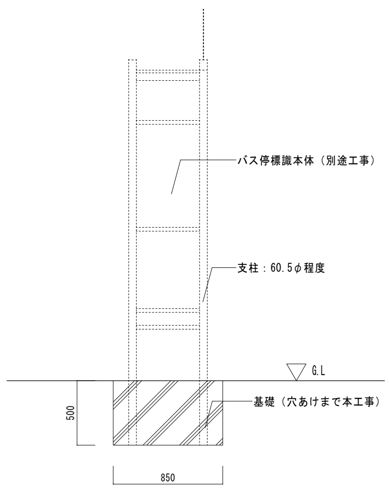
正面図
