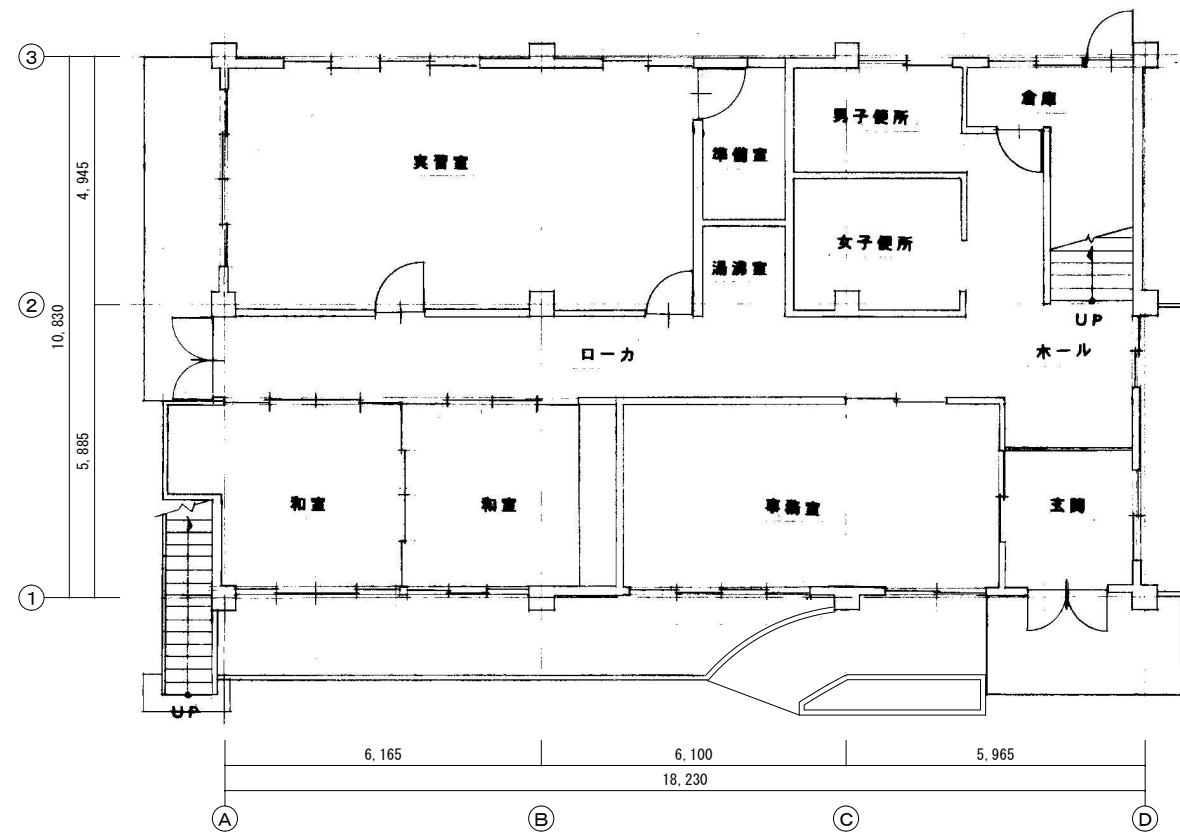
1階平面図(新築時) S=Non Scale
