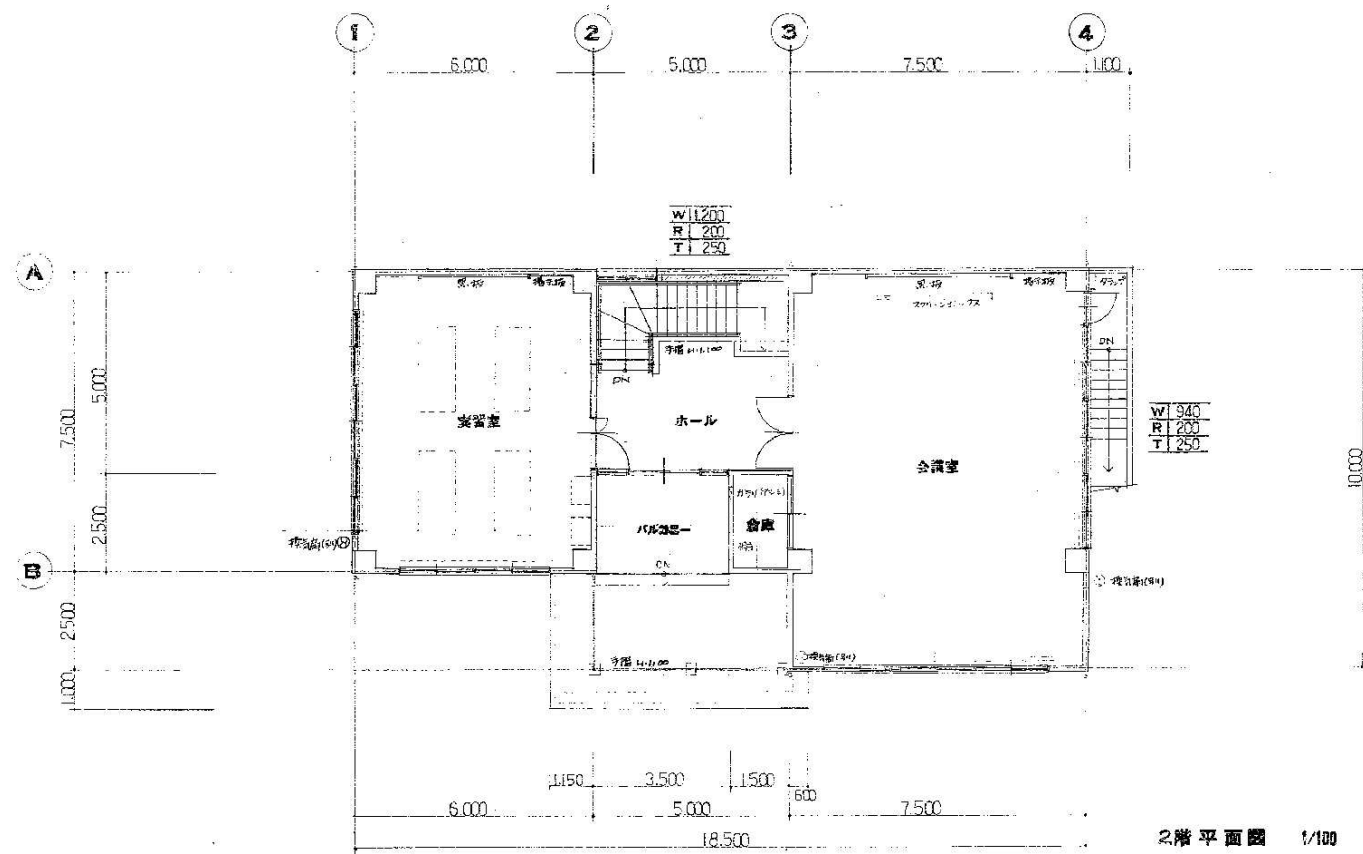
2階平面図(新築時) S=Non Scale
