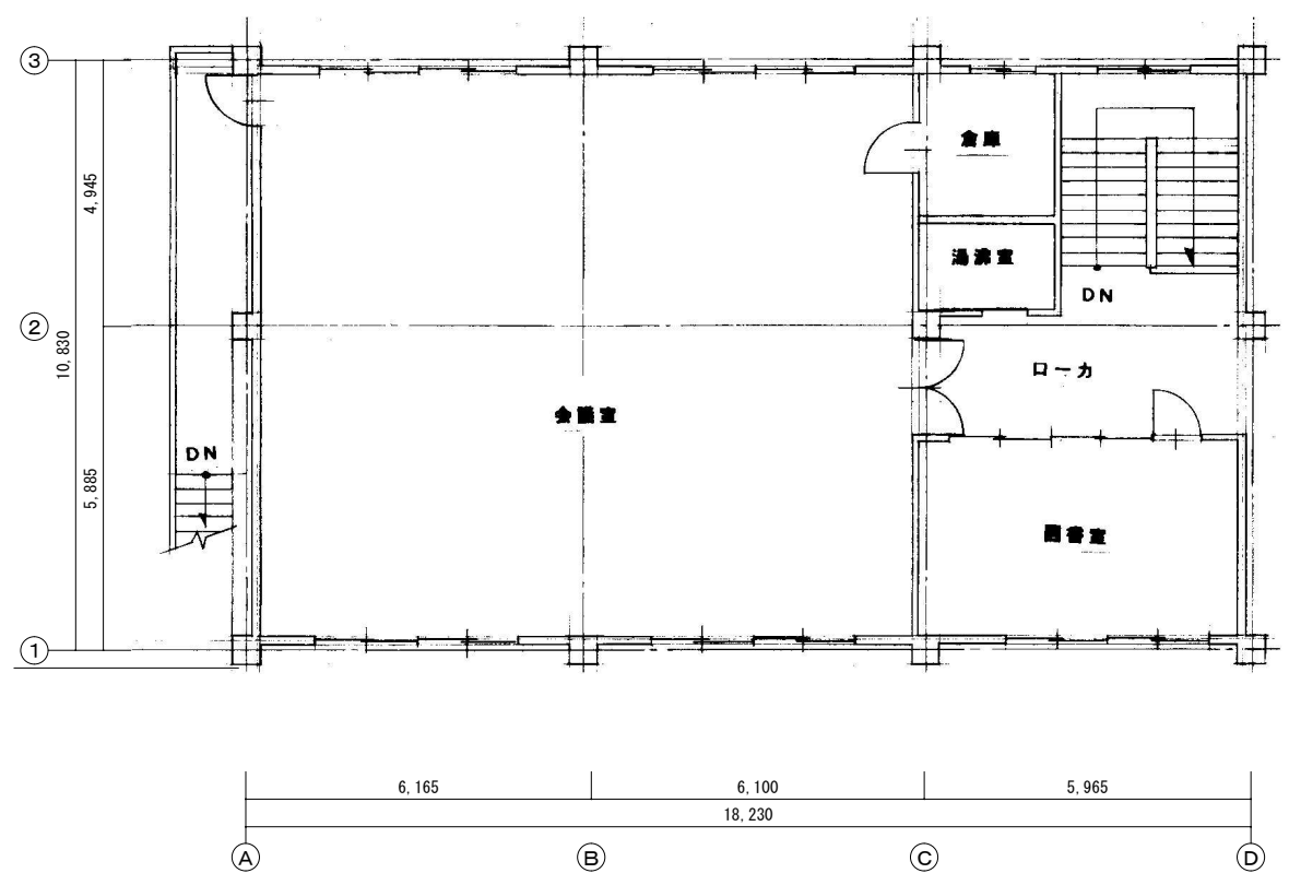
2階平面図(新築時) S=Non Scale
