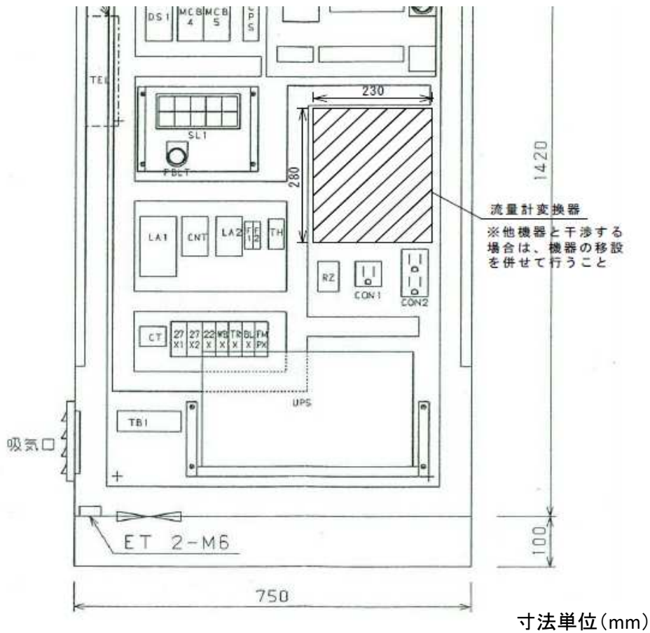
盤内配置図
