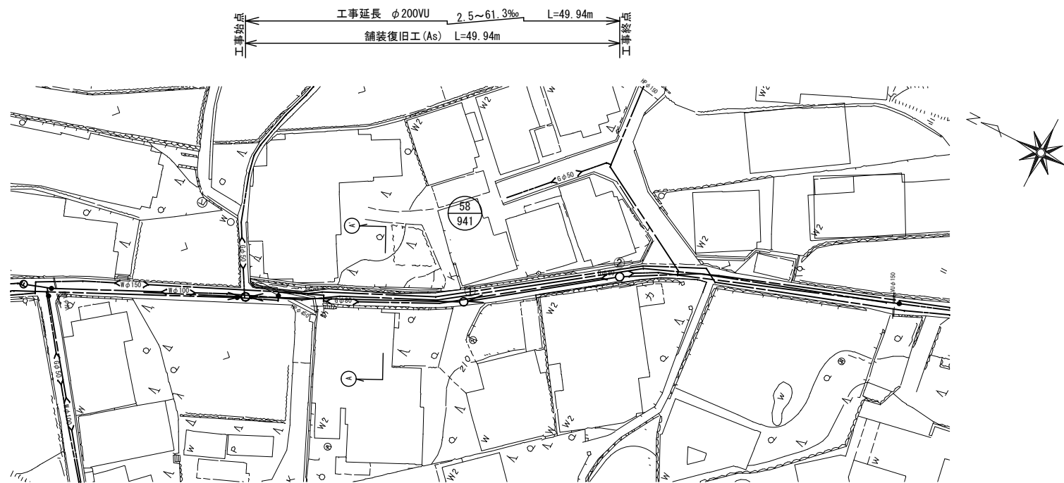
管渠埋設平面図 S=1/500
