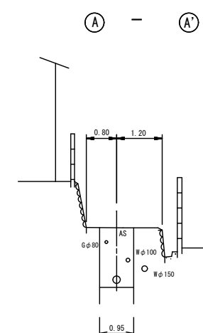
標準断面図 S=1/100
