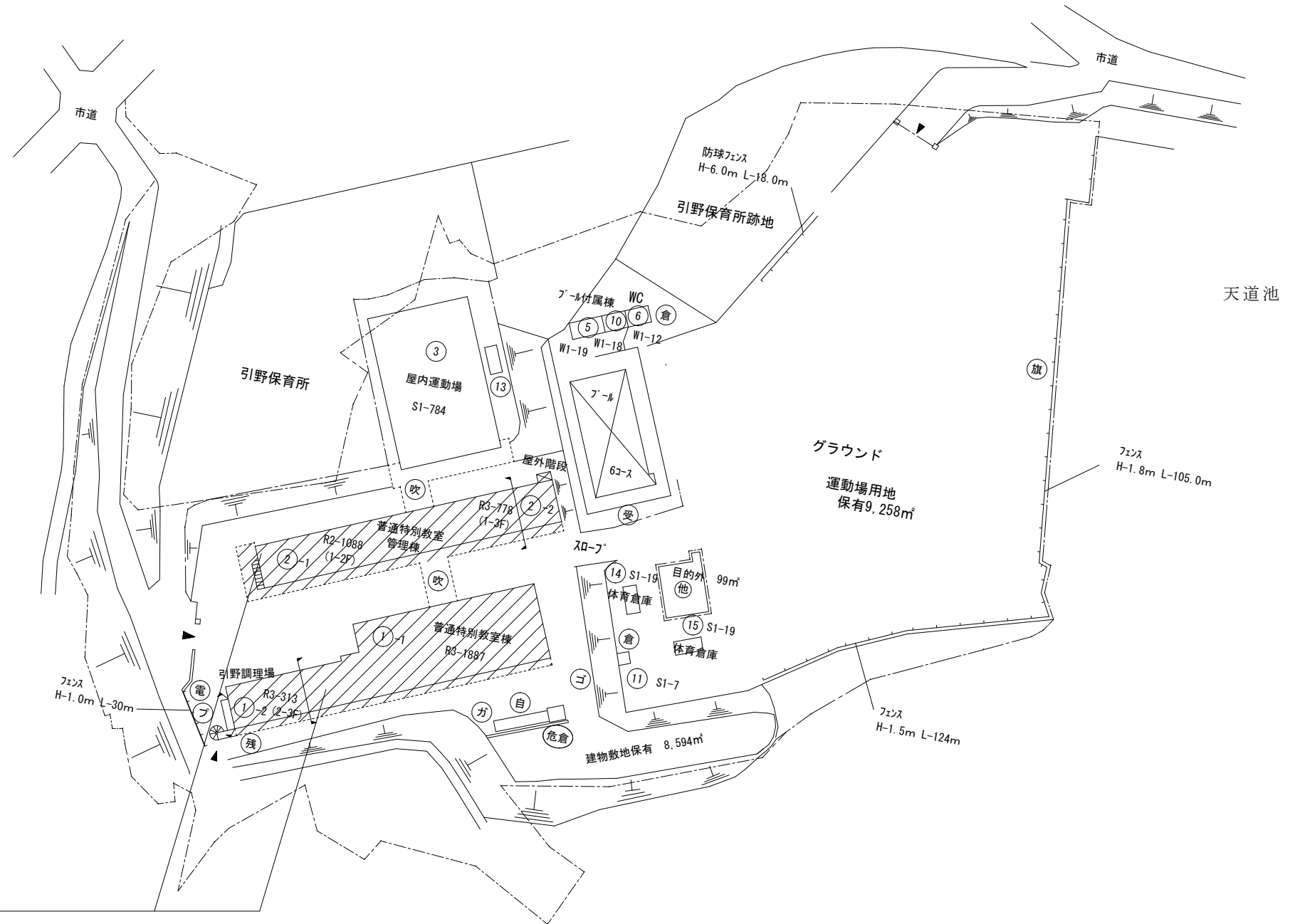
配置図 S=1/800
