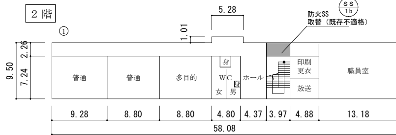
2階平面図 S=1/300
