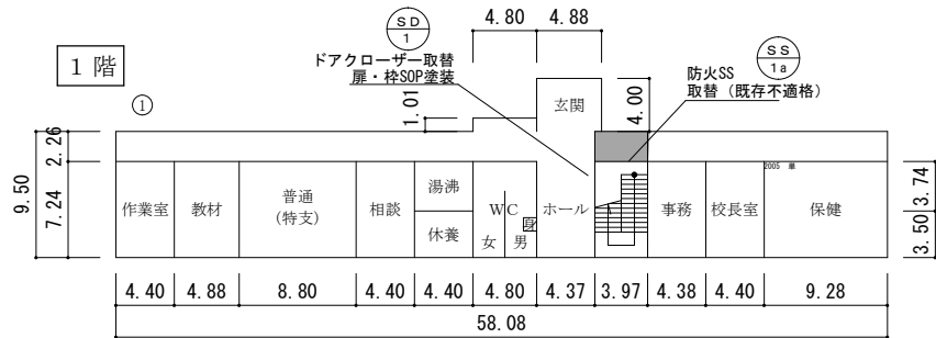
1階平面図 S=1/300
