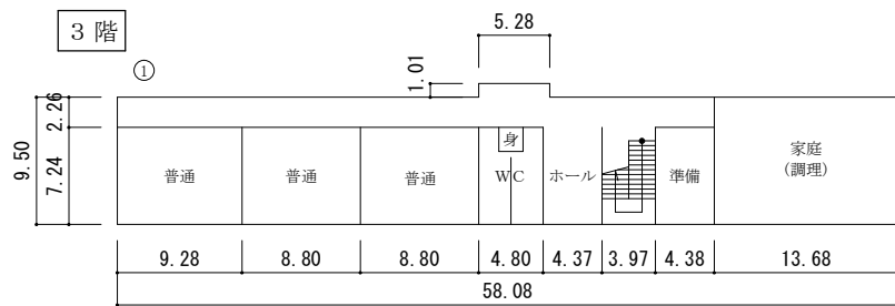
3階平面図 S=1/300
