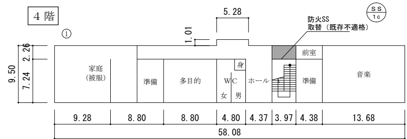
4階平面図 S=1/300
