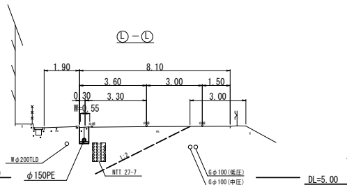
標準横断面図 S=1/100
