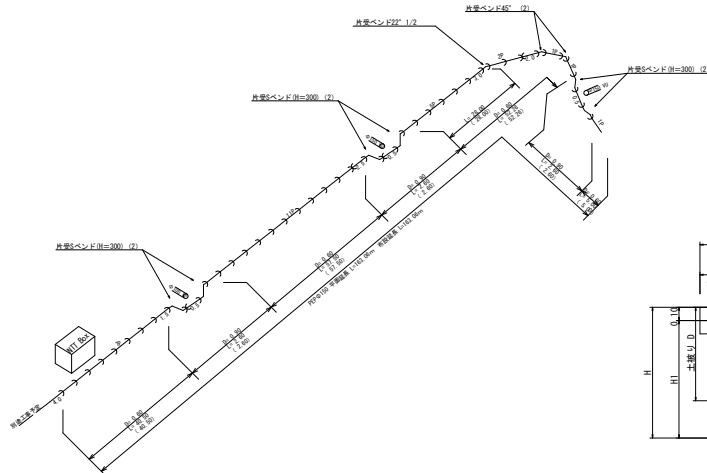
圧送管詳細図 S=Non
