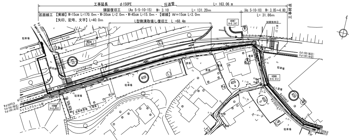
管渠埋設平面図 S=1/500
