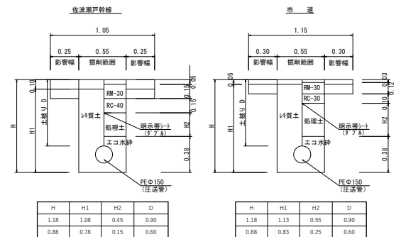
舗装断面図 S=1/50
