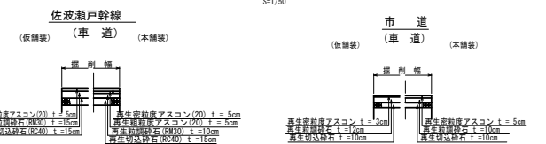
舗装断面図 S=1/50
