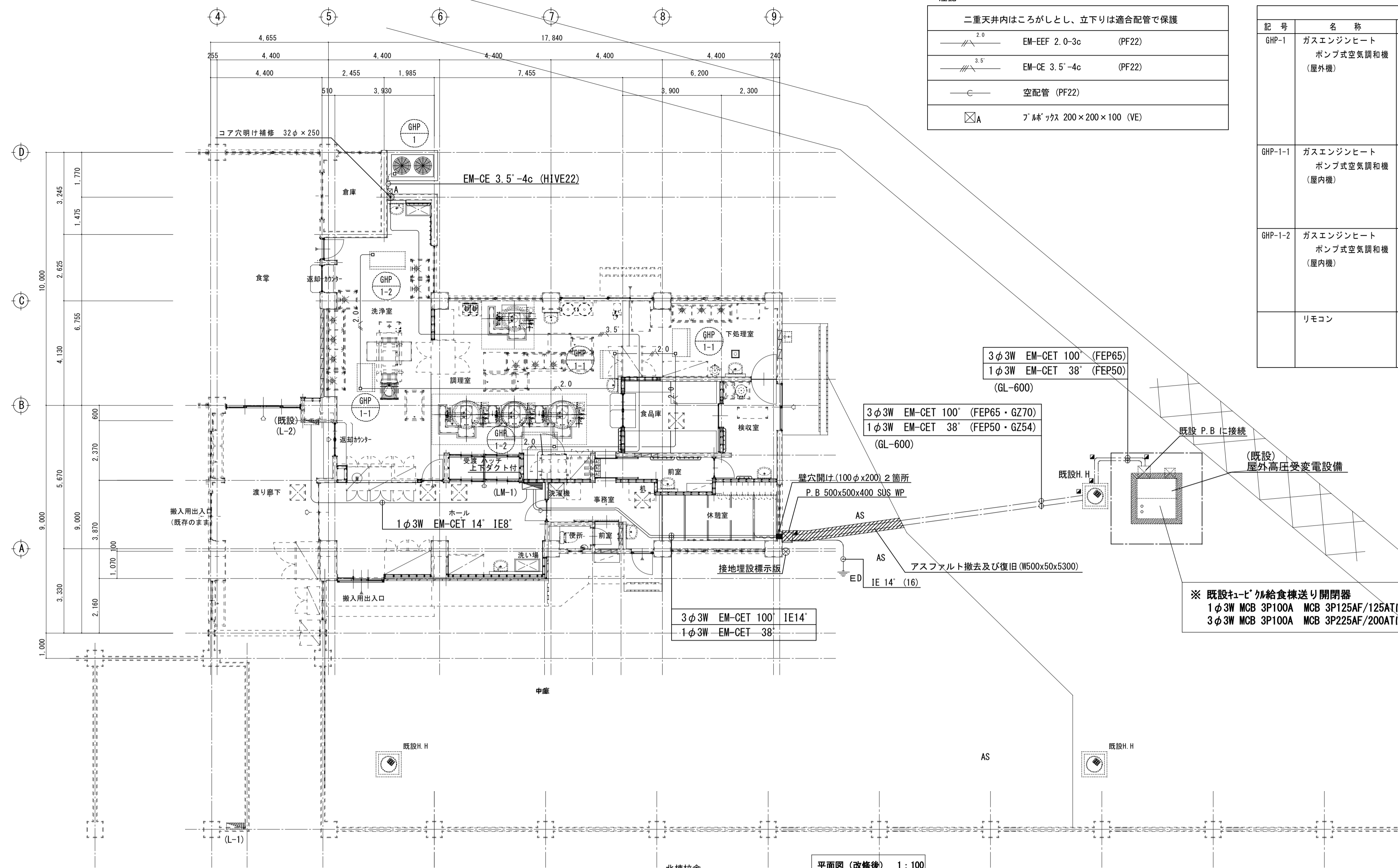
北棟校舎 平面図 (改修後) 1:100
