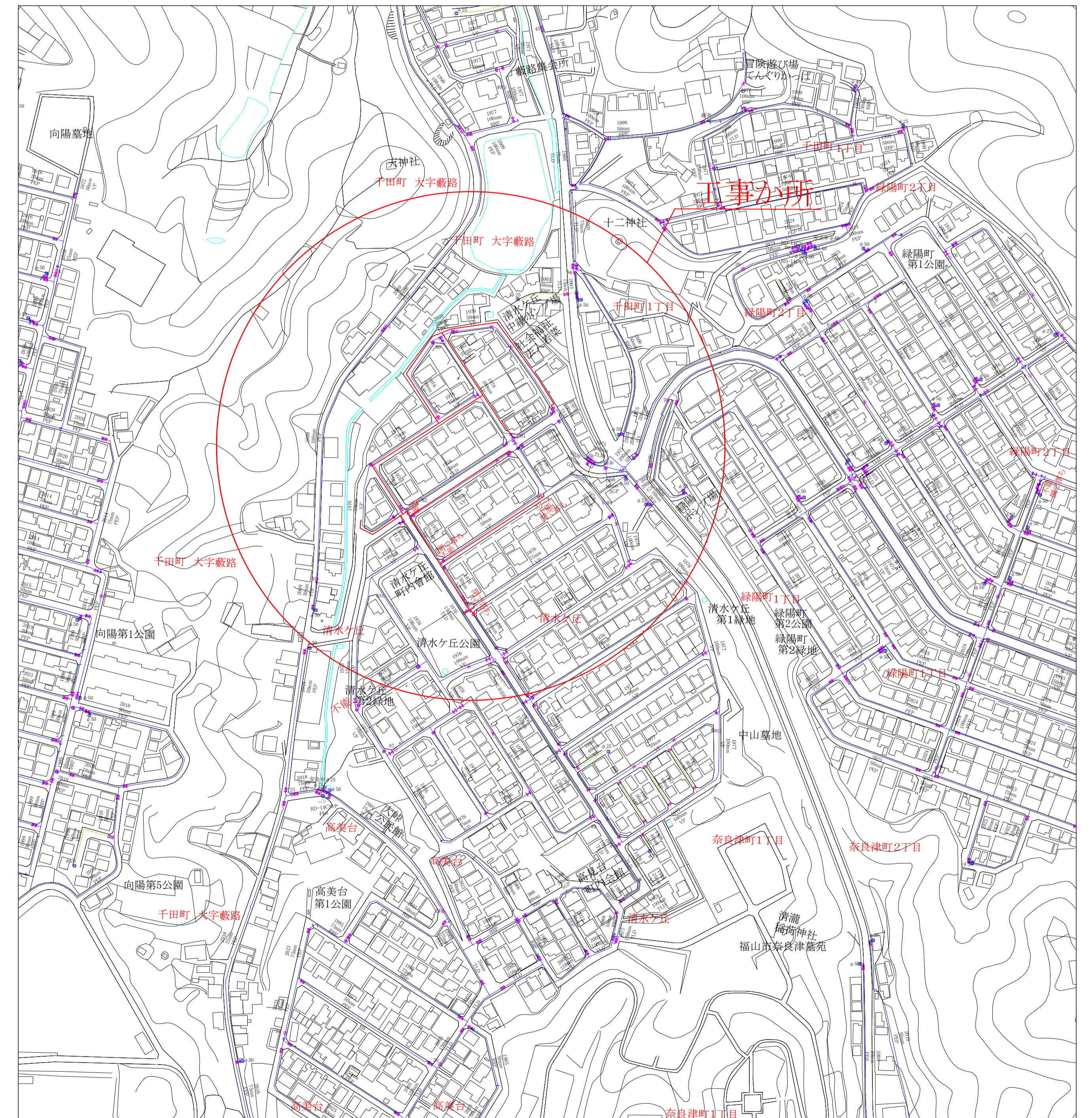
配管図 S=1/2500
