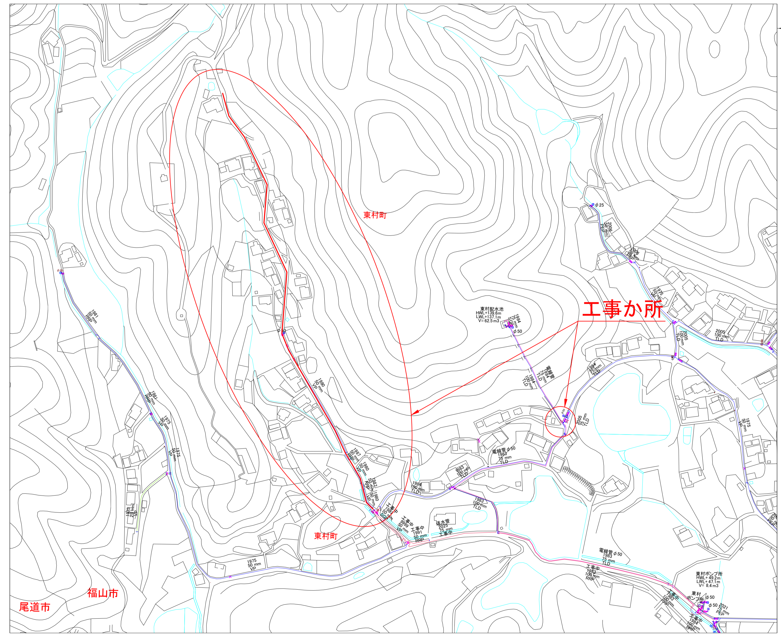
配管図 S=1/2500
