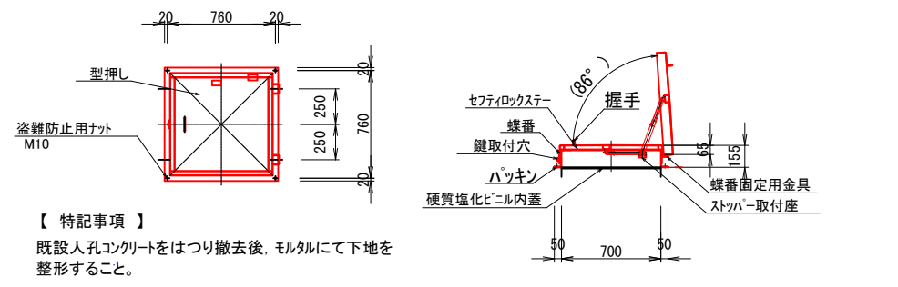
人孔蓋詳細図 S=1/25 SUS304
