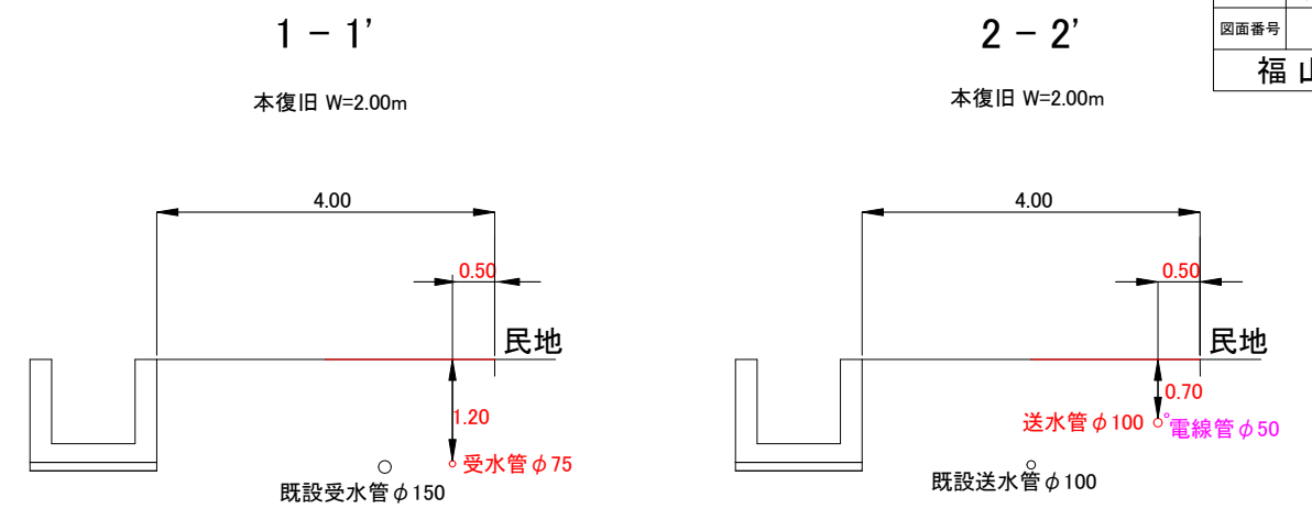
ハンドホール改良詳細図 S=1/25
