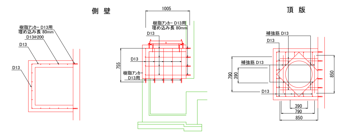
ハンドホール配筋図 S=1/25
