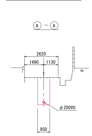
横断面図 S=1/100
