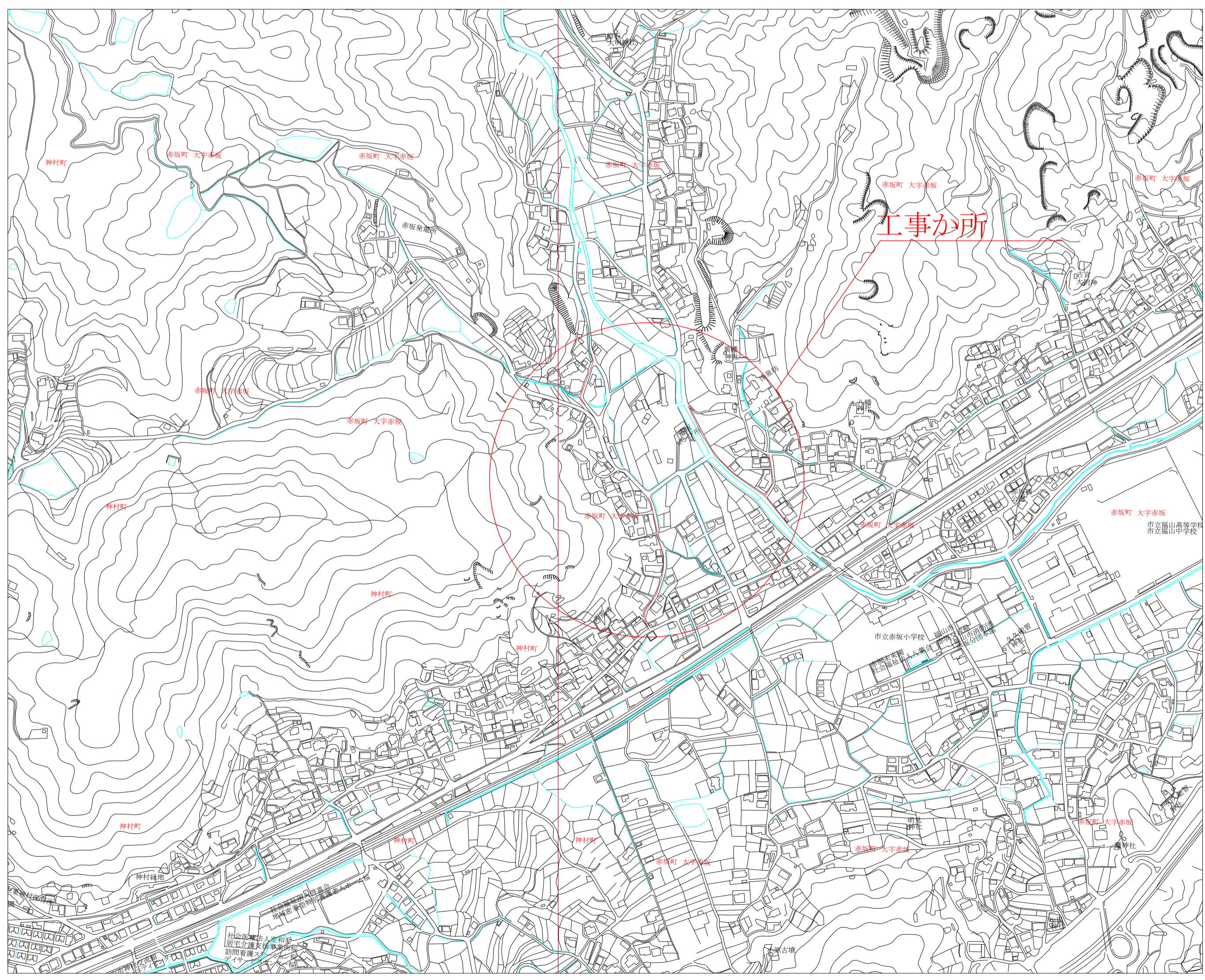
位置図 S=1:5000
