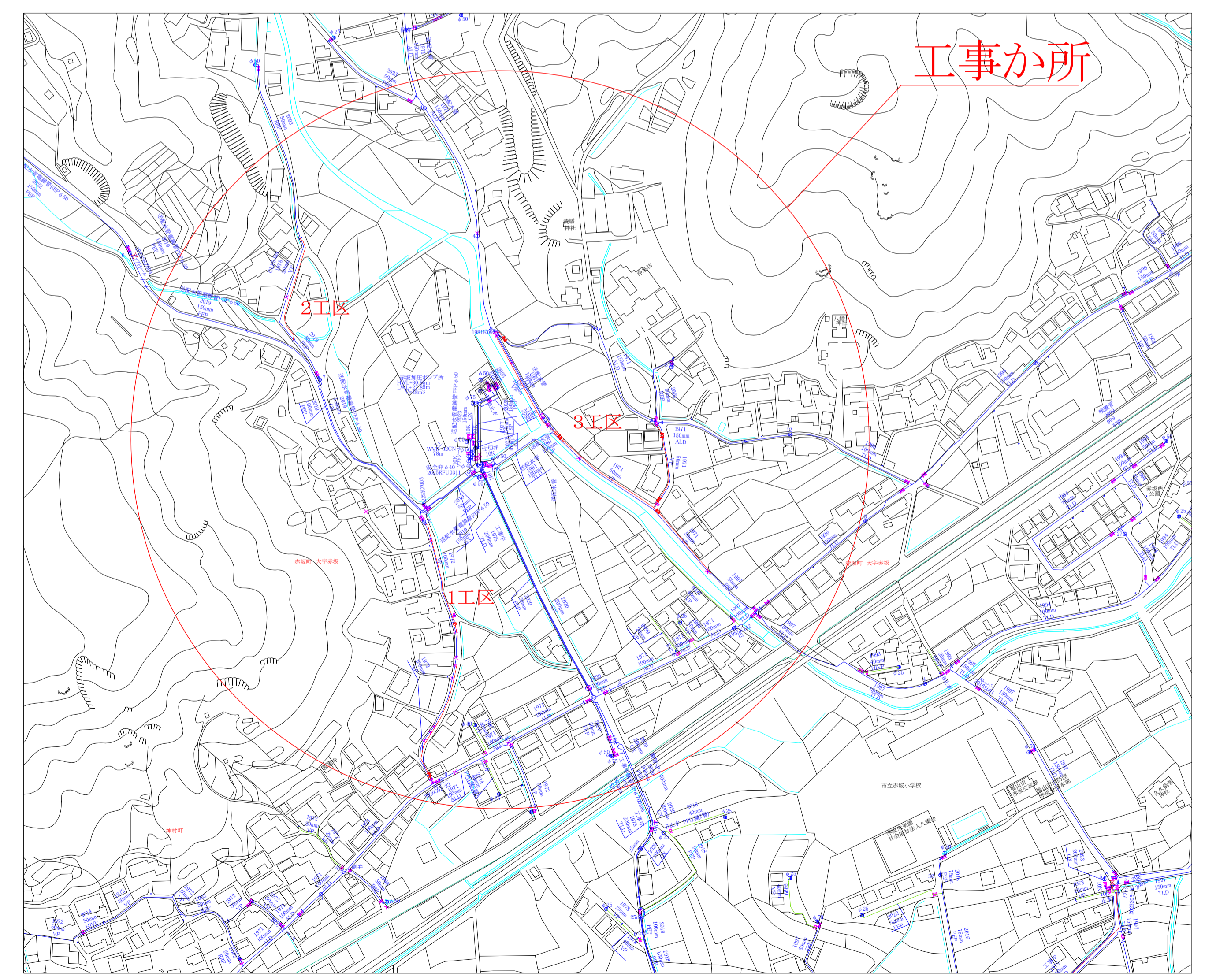
配管図 S=1:2500
