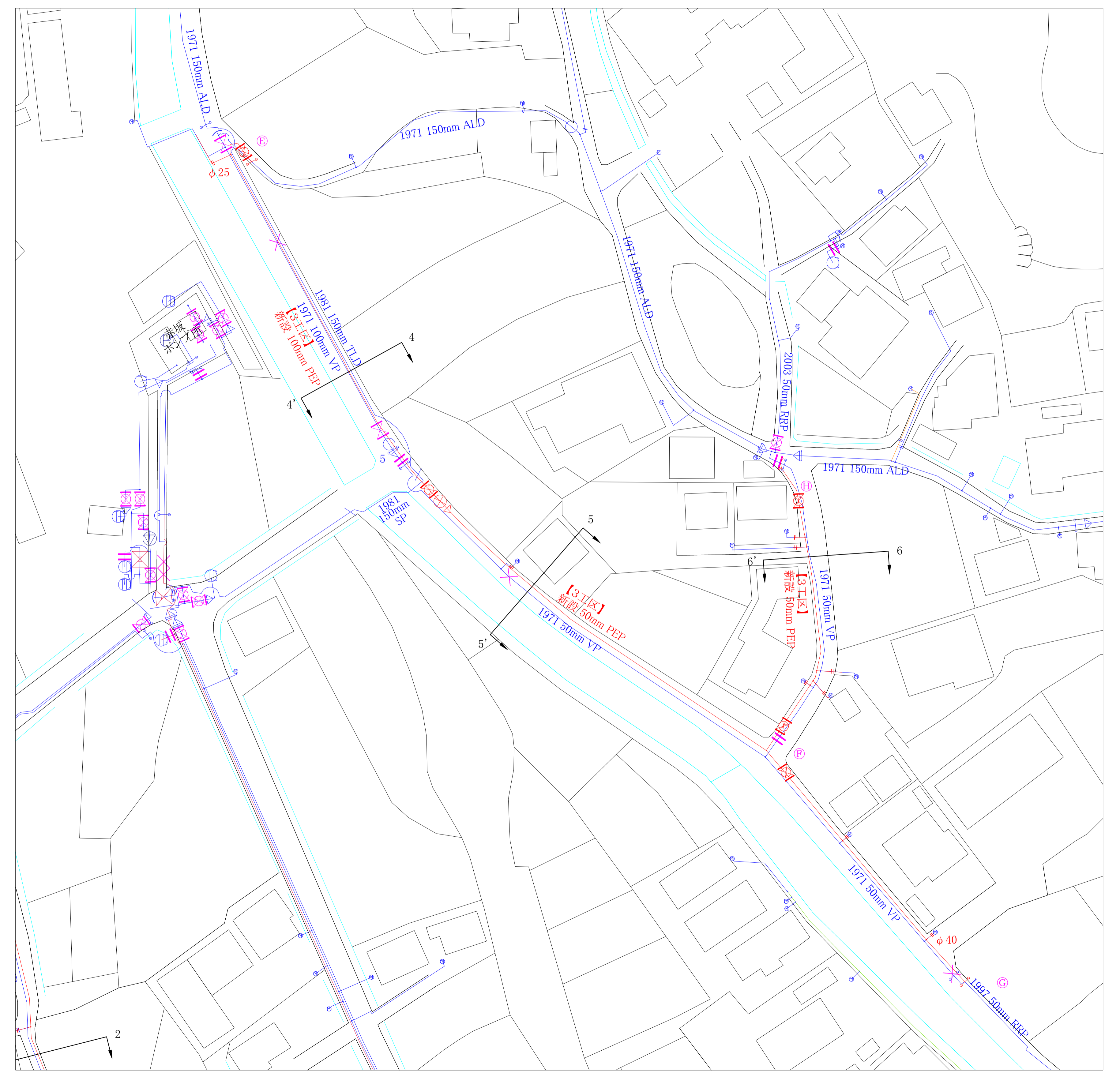
平面図(3工区) S=1:500
