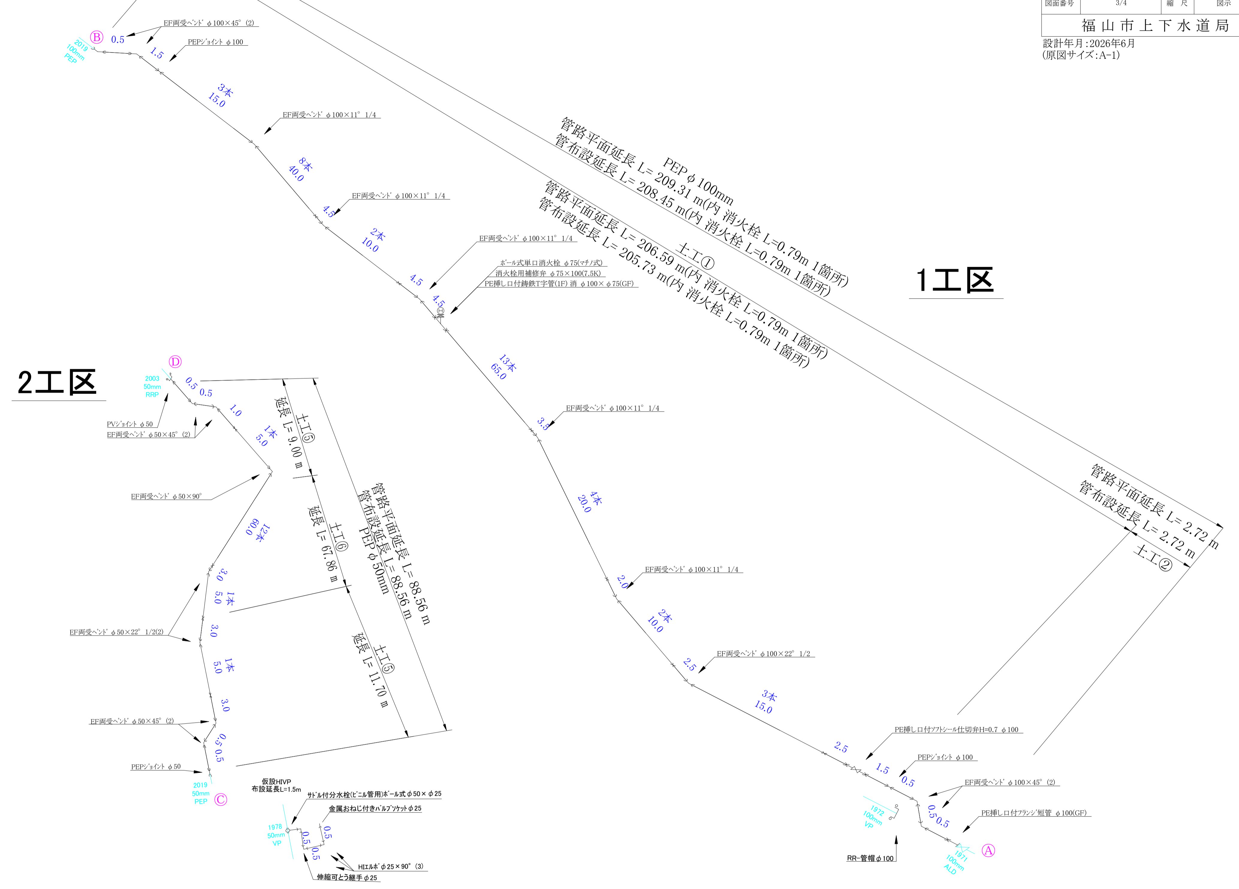
配管系統詳細図(1) S=Non
