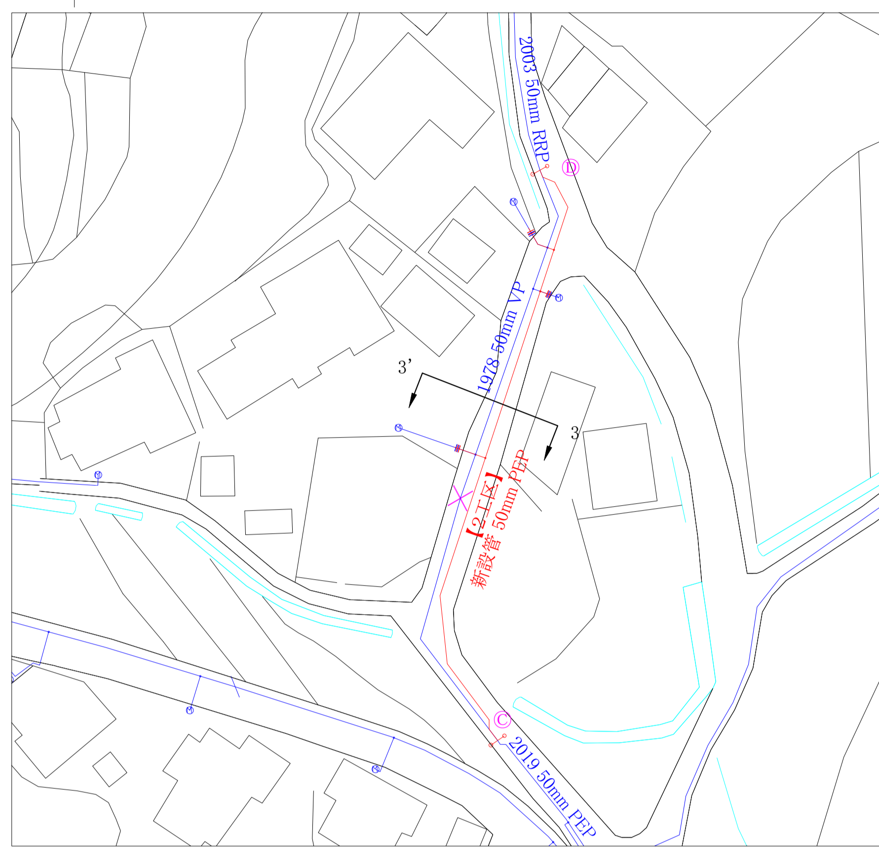
平面図(2工区) S=1:500
