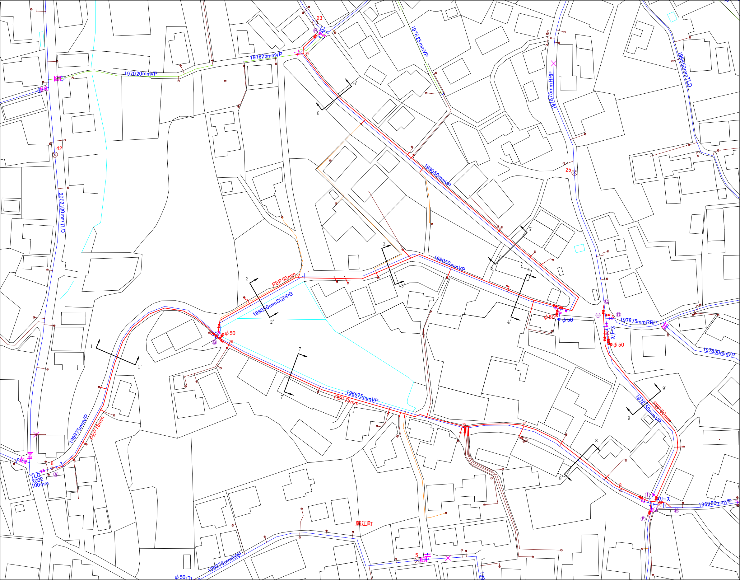
平面図 S=1/600
