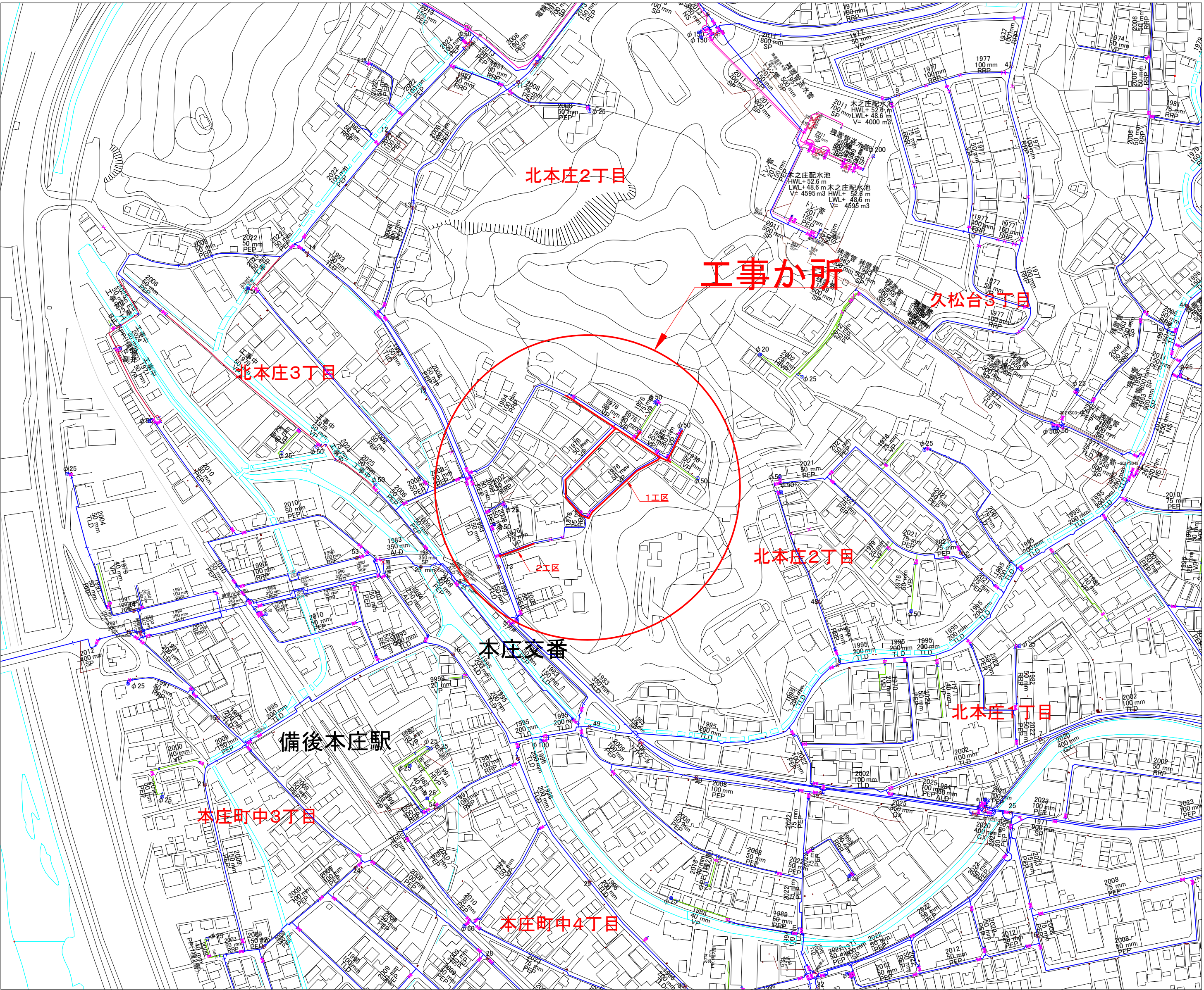
配管図 S=1:2500
