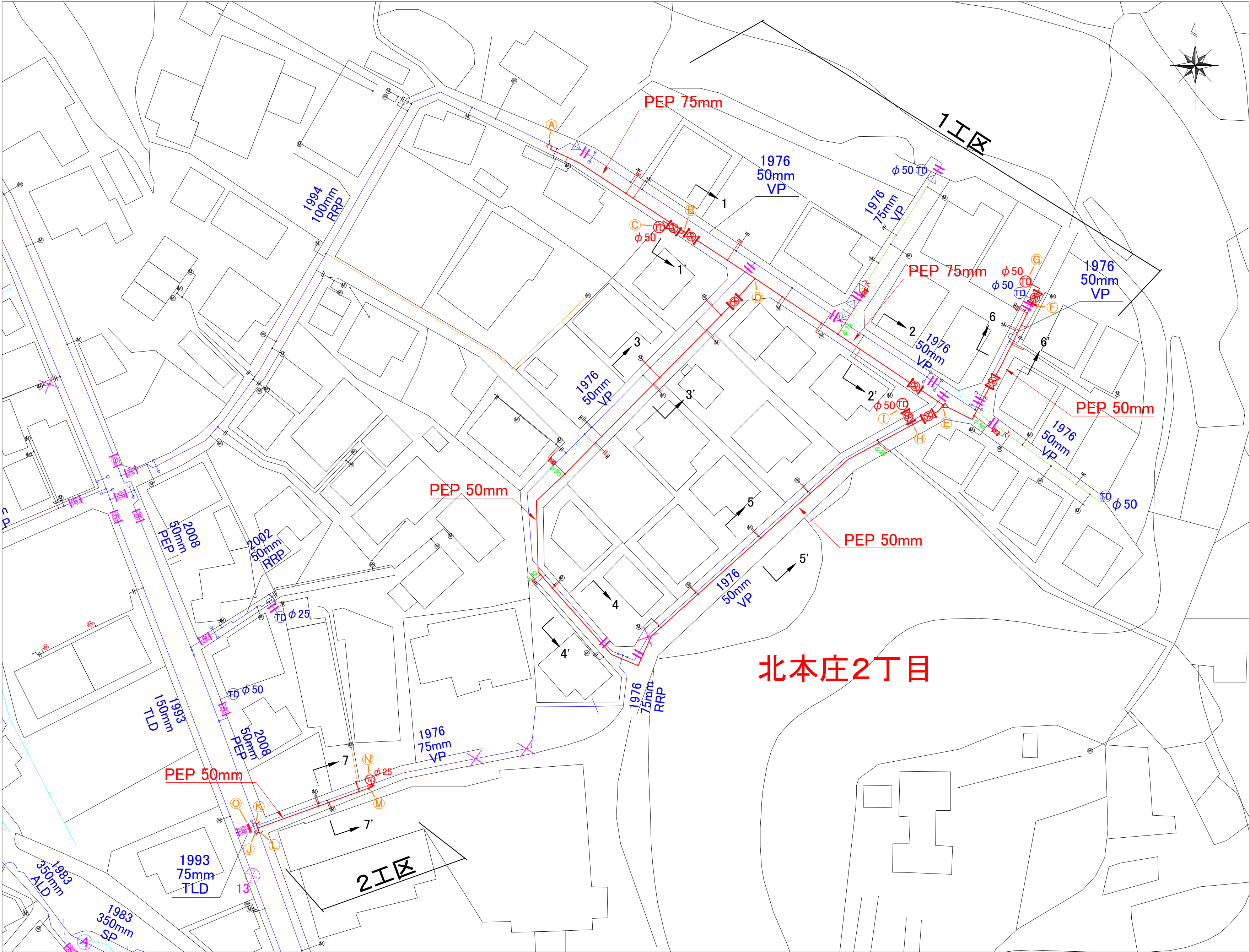
平面図 S=1/500
