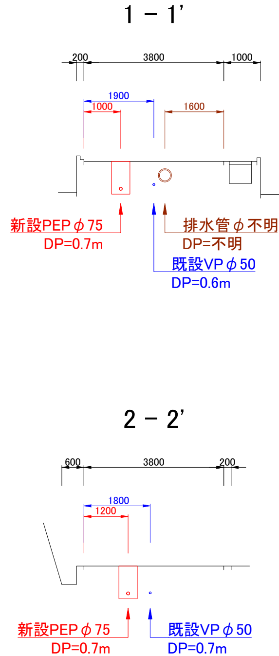
横断面図 S=1/100
