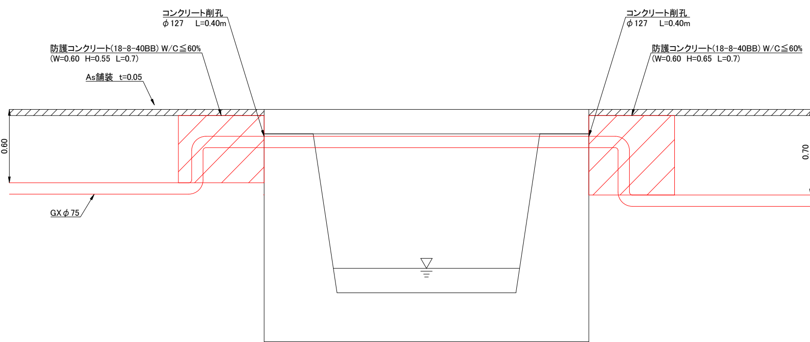
水路添架部詳細図 S=NON
