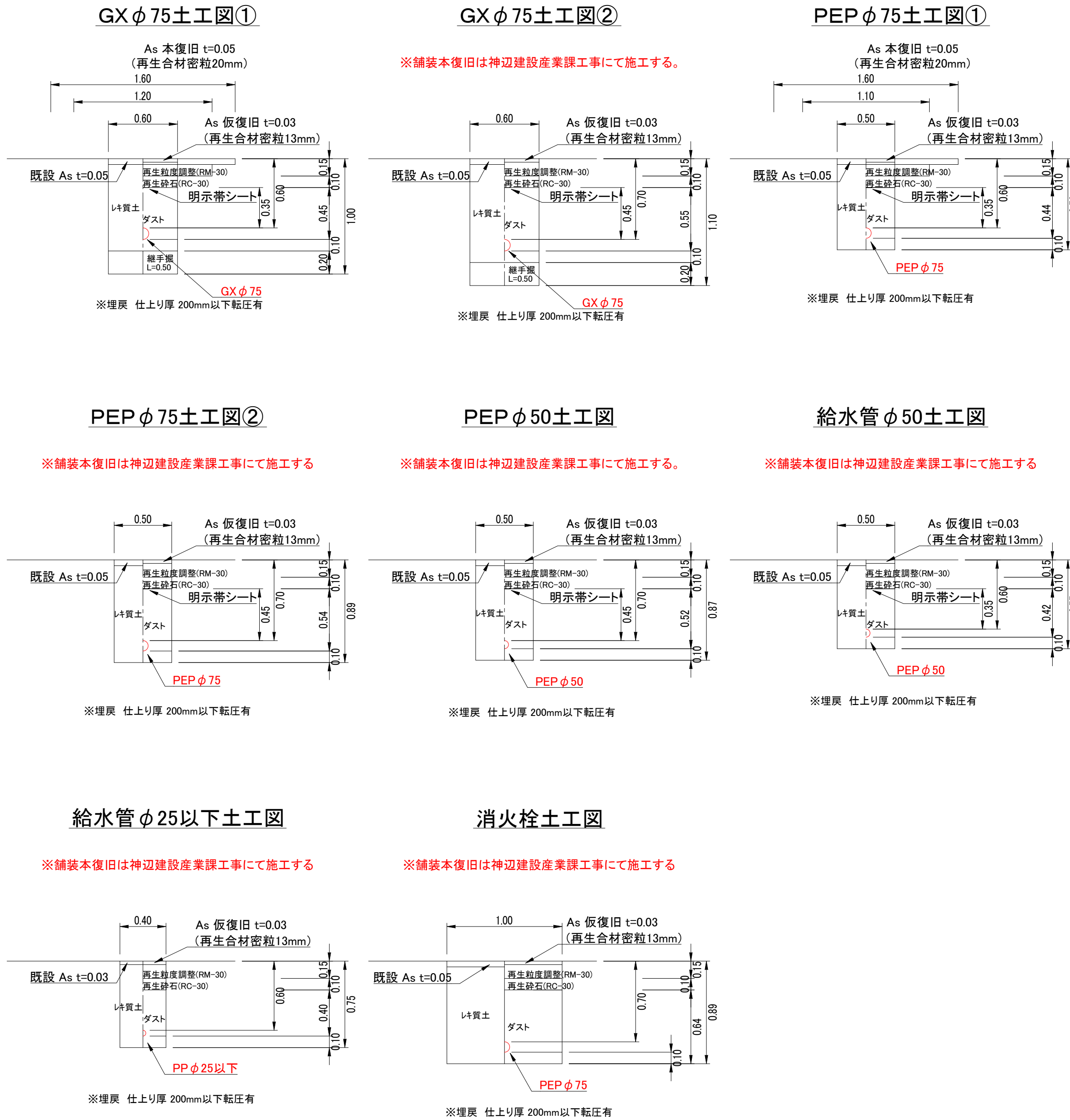
土工図 S=1/30
