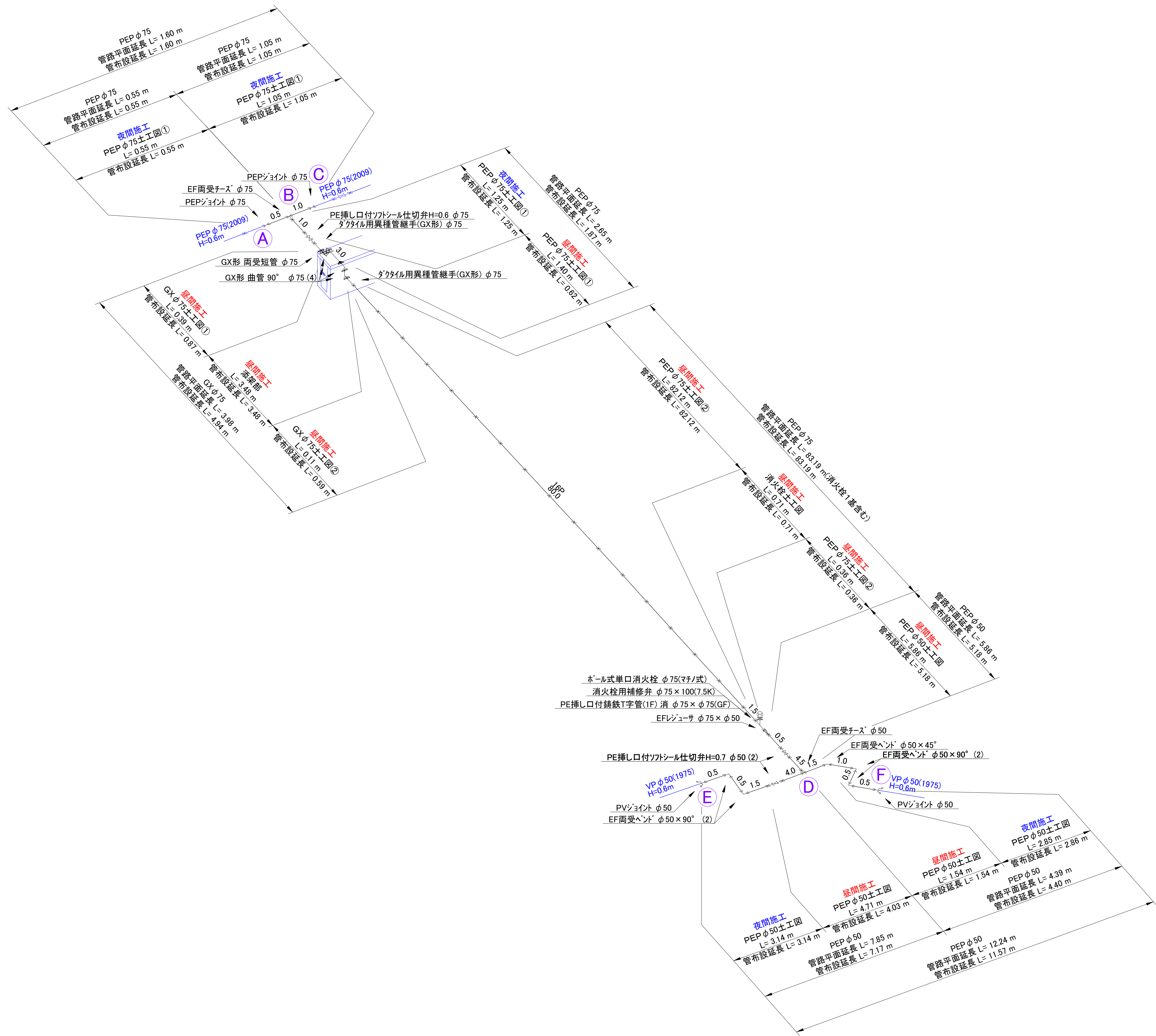
配管系統詳細図 S=NON
