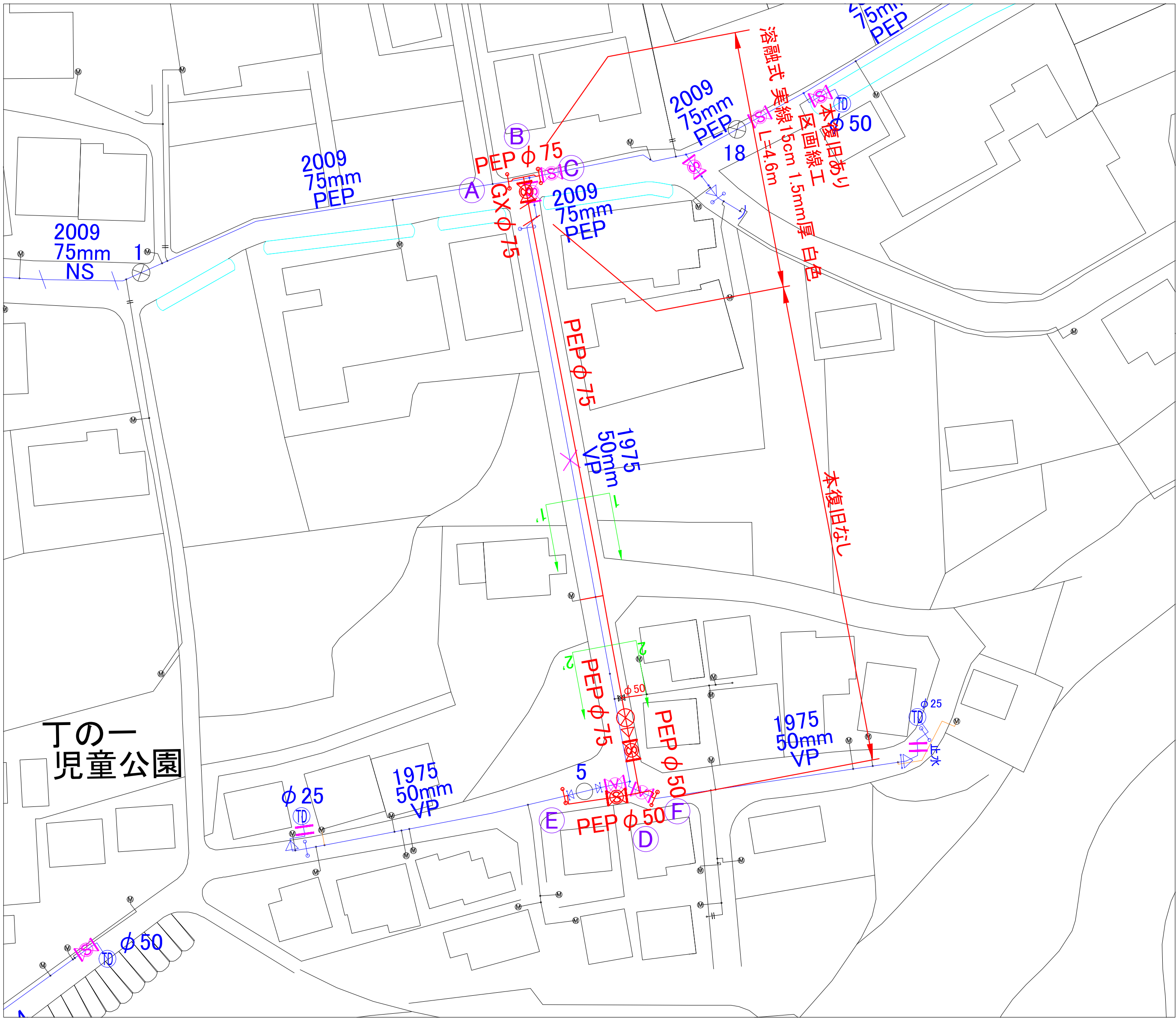
平面図 S=1/500
