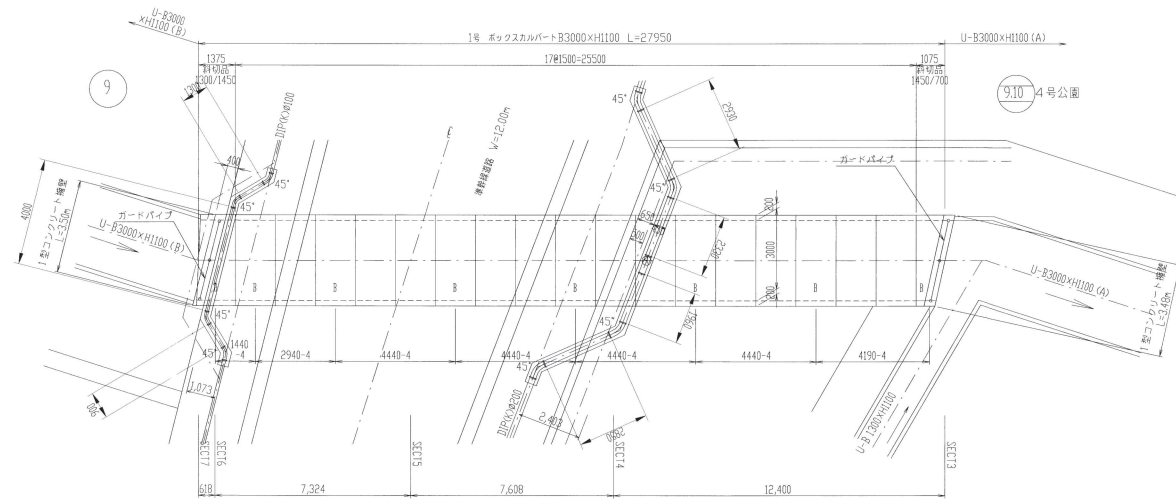
平面図
