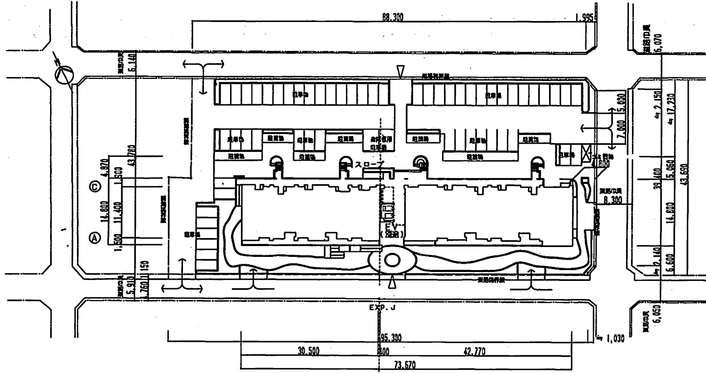
配置図
