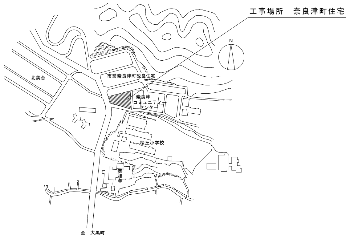
附近見取図
