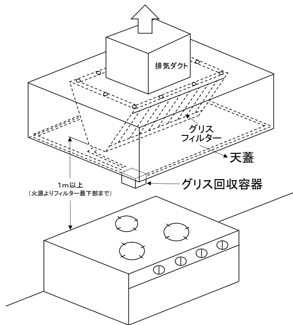
図 3 - 4 - 4 グリスフィルターの設置例
