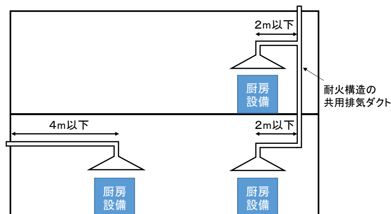
図 3－4－6 火炎伝送防止装置の設置を要しない例
