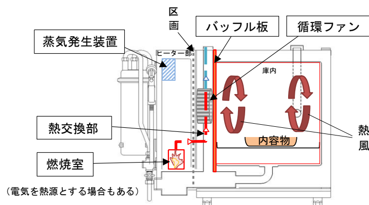
＜コンベクションオープンのイメージ図（ガス式・蒸気発生装置付）＞
