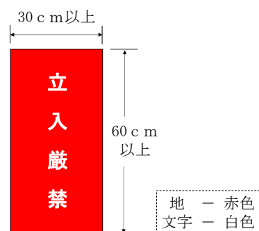
図18-1 立入りを禁止する旨を表示した標識の例
