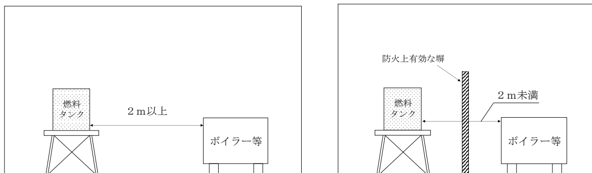
図 3 2 - 4 - 3 燃料タンクとボイラー等を併設する場合の例
