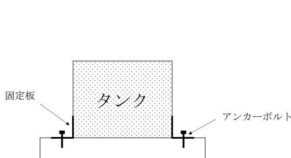
図 3 2－4－1 基礎上に固定する例
