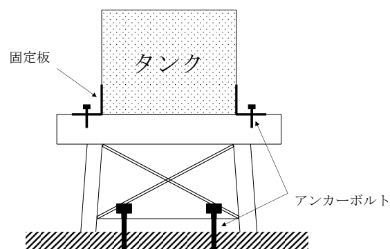
図 3 2－4－2 架台上に固定する例
