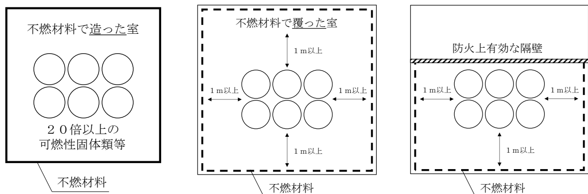
図 3 4 - 1 20 倍以上の可燃性固体類等を屋内に貯蔵し、又は取り扱う場合の例
