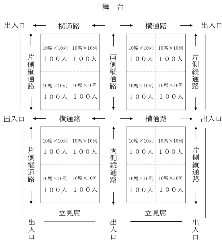
図 4 8 - 9 劇場の座席配列の設計例 (20 席×20 列の場合)
