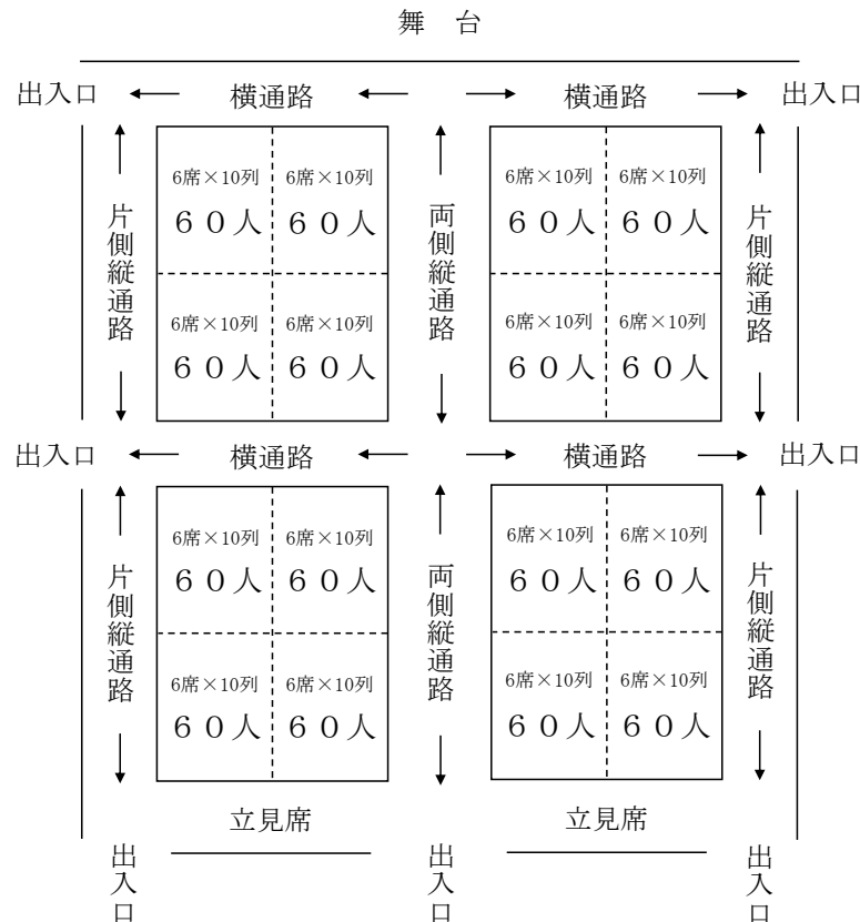
図48-8 劇場の座席配列の設計例（12席×20列の場合）
