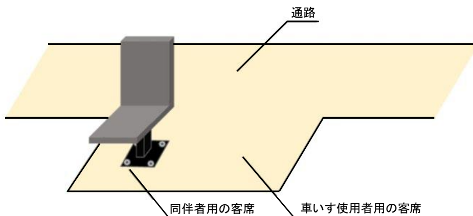
図48-1 車いす使用者用の客席に隣接してあらかじめ固定したいす席を設ける方法
