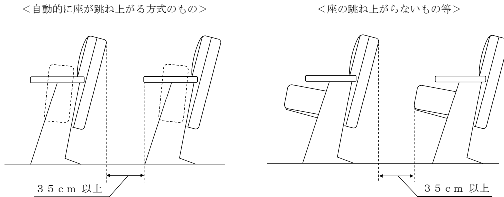
図 48-5 いす席の間隔
