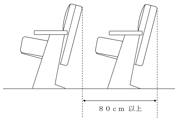
図 4 8 - 4 いす背の間隔
