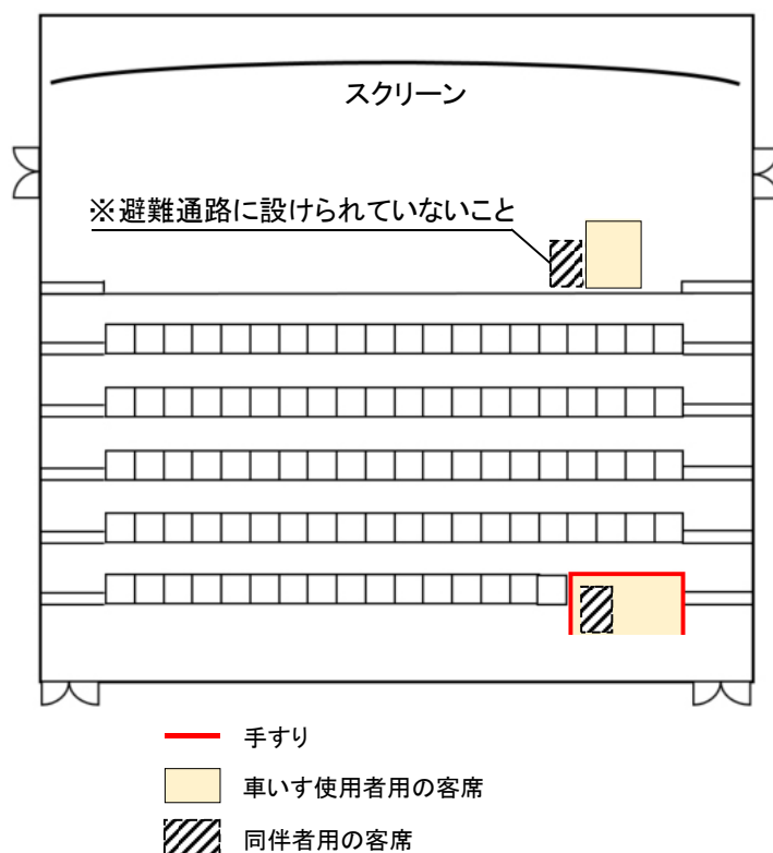
図 4 8 - 3 特例により同伴者用の客席の床への固定が免除される場合の例 【出典：令和 7 年 6 月 26 日付け消防予第 248 号「劇場等における車椅子使用者客席の同伴者席の固定に係る取扱いについて」】
