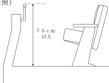
図 48-7 落下防止の手すり
