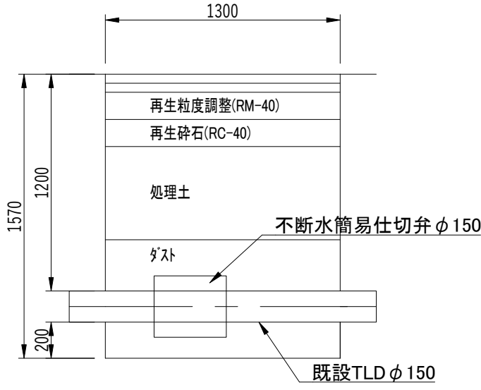
断面図1
