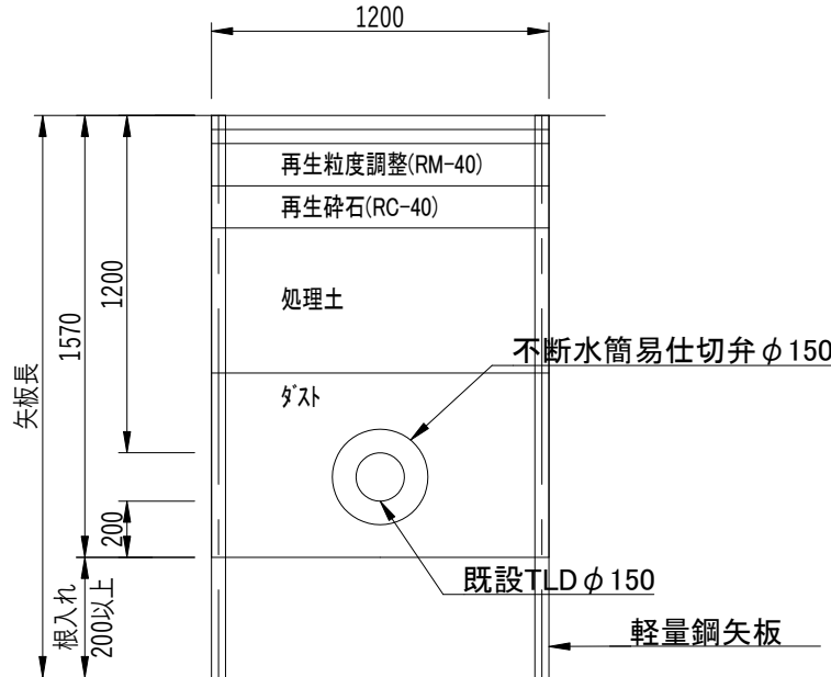
断面図2
