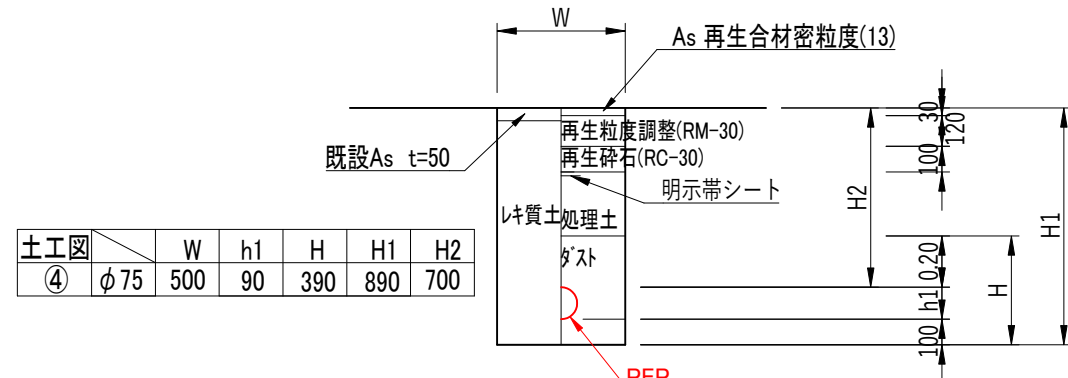
PEP土工図 (市道車道部)
