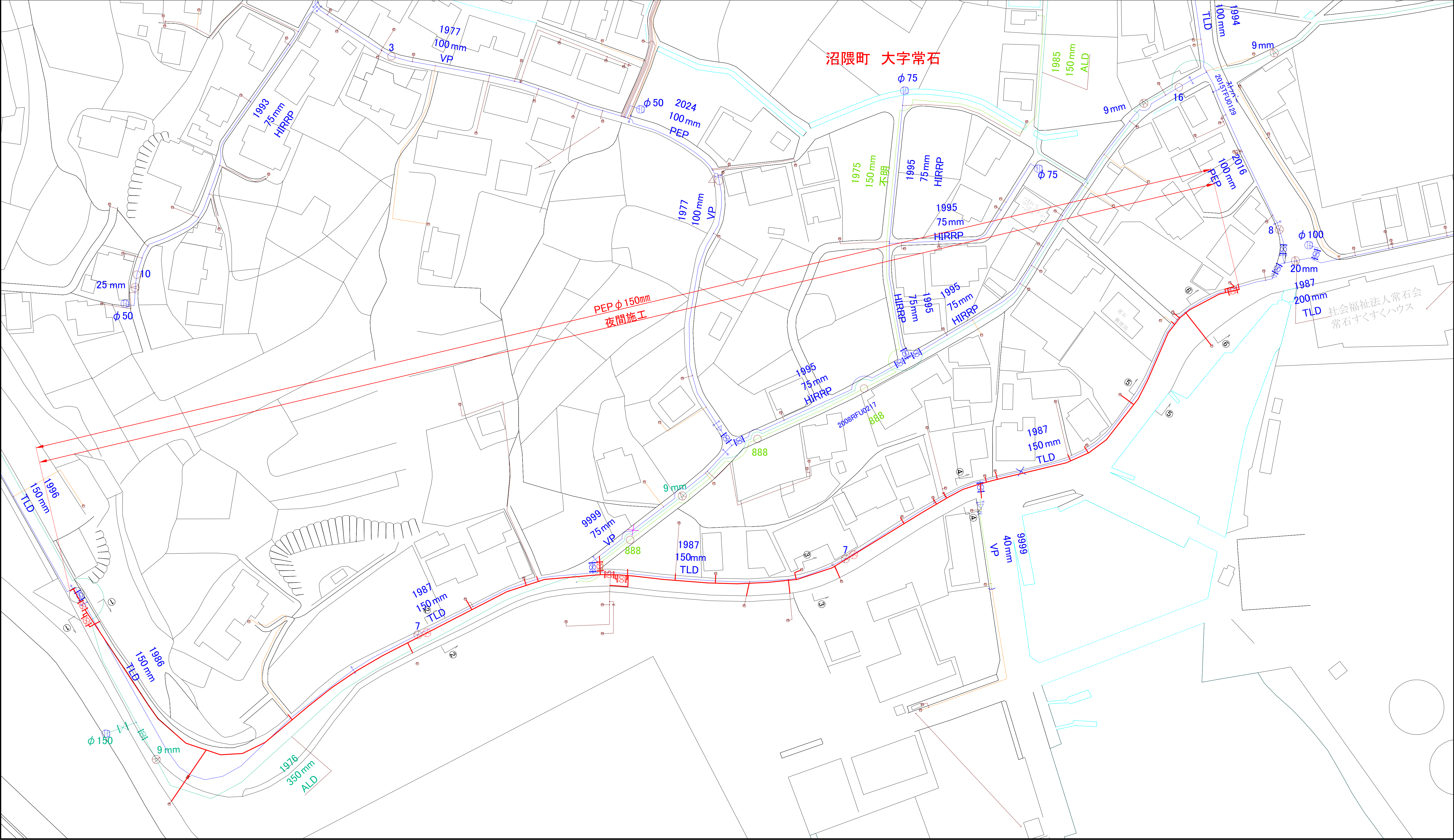
平面図 S=1/600
