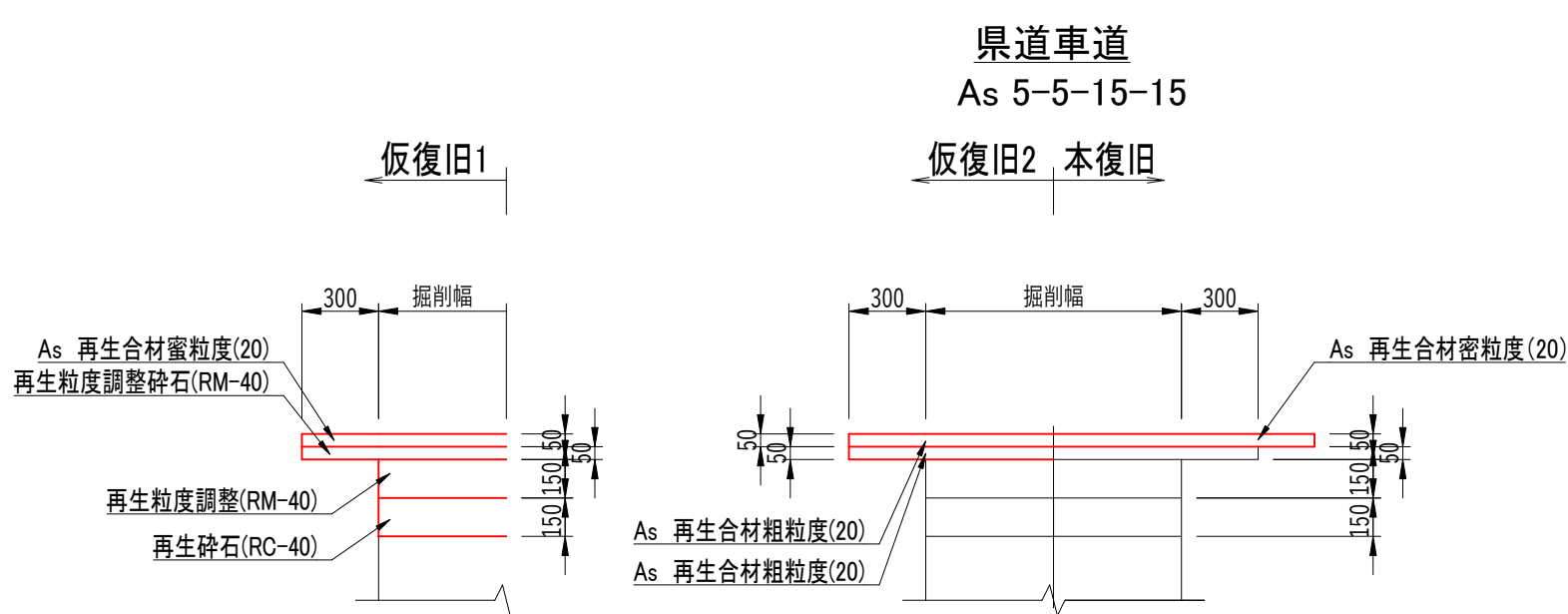
舗装復旧図 S=Non
