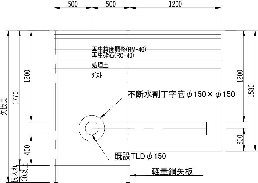
断面図
