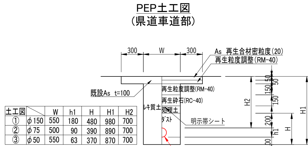
標準土工図 S=1/30
