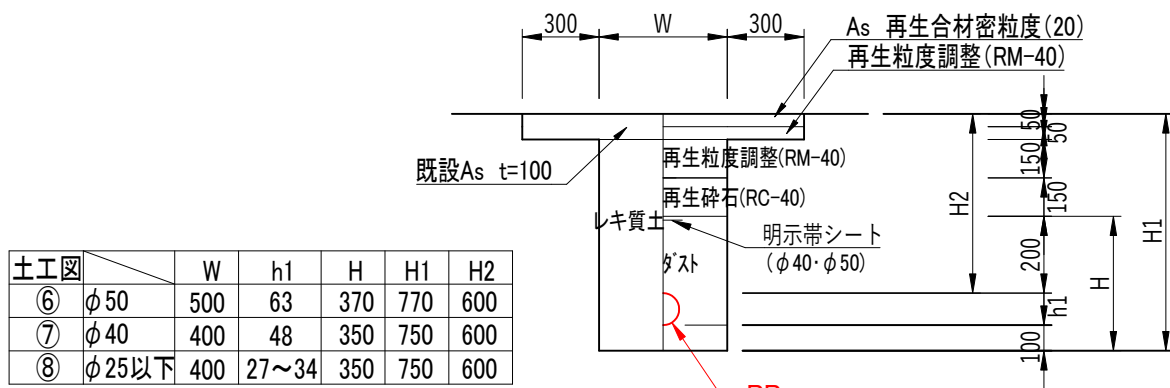
②PP土工図 (県道車道部)
