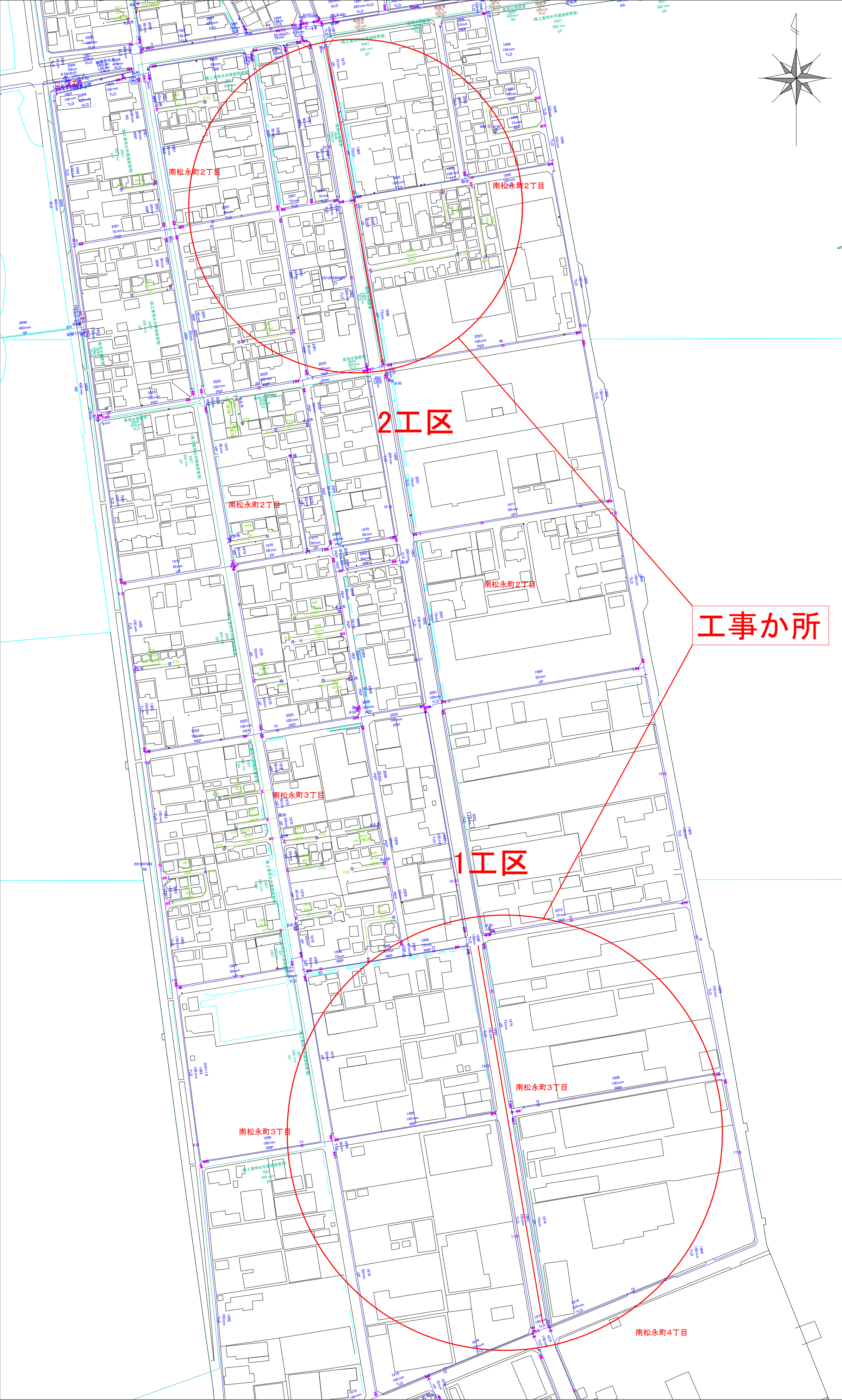
配管図 S=1/2,500
