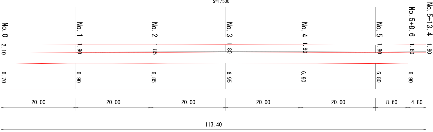
舗装展開図 S=1/500
