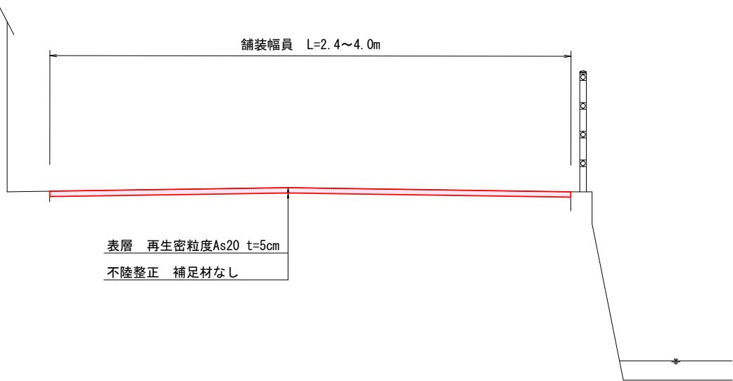
標準断面図 S=1:50
