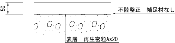
舗装構成 S=1:10
