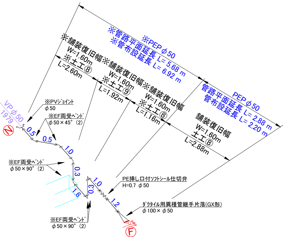
PEP φ 50(4) (※は単独分)
