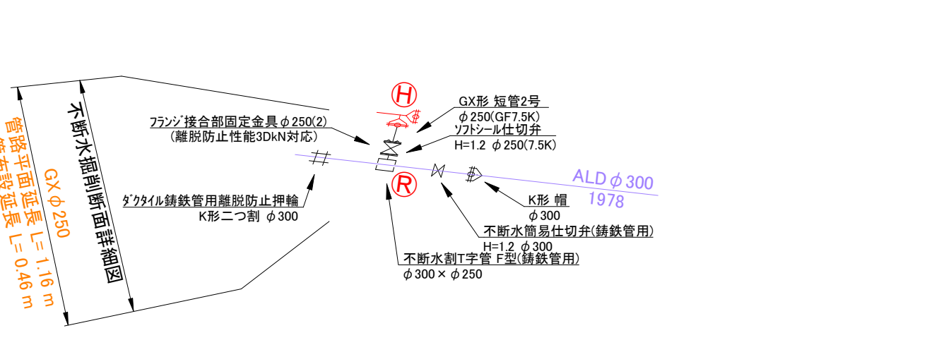
不断水分岐部 φ 300 × φ 250 (すべて単独分)
