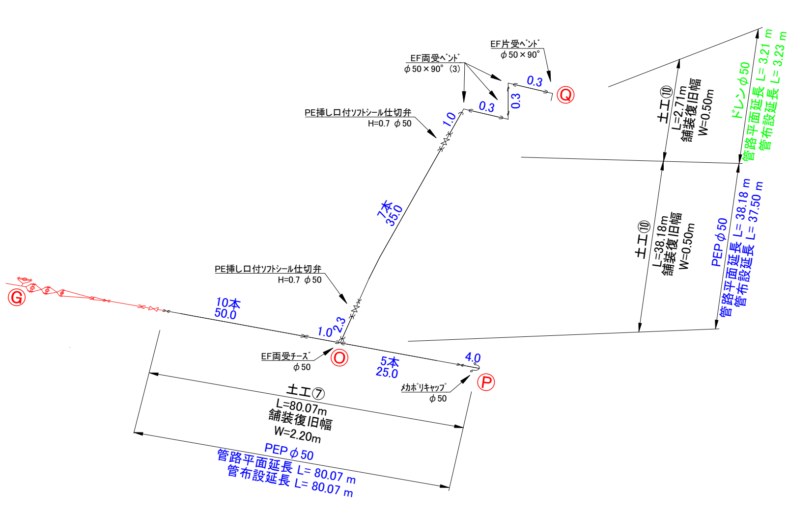
PEP φ 50・ドレン φ 50(5) (すべて単独分)
