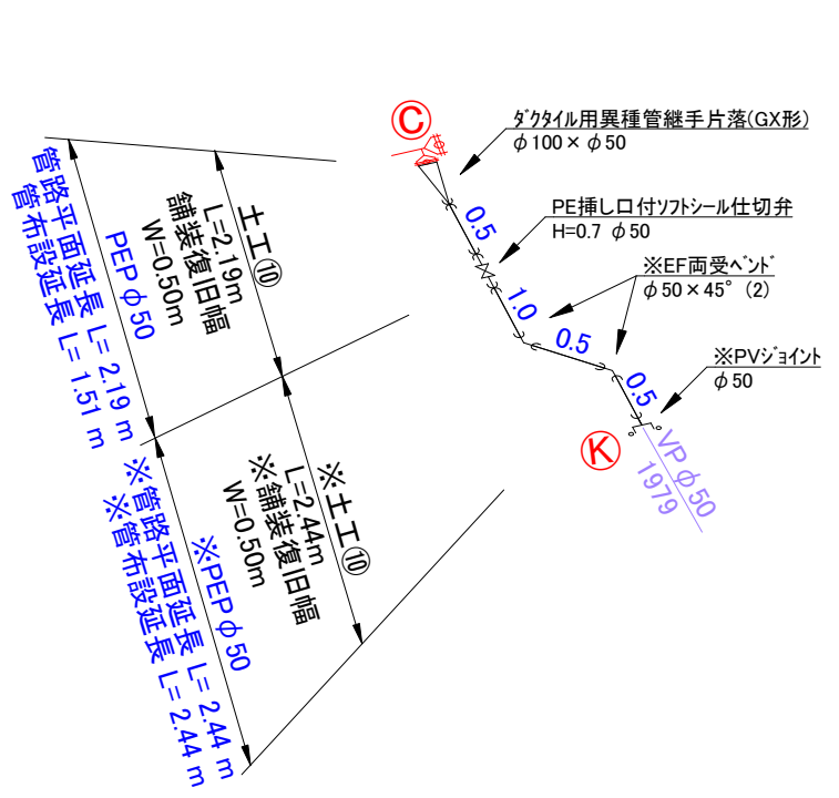
PEP φ 50・ドレン φ 50(3) (※は単独分)
