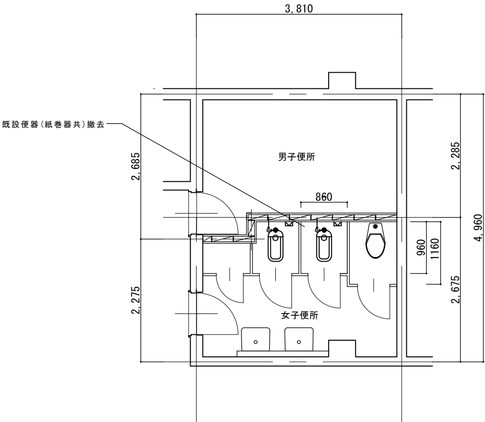
改修前 便所平面詳細図 1:50
