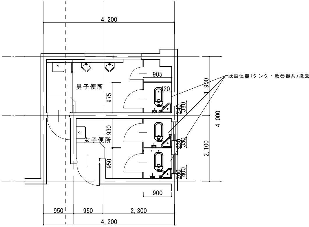
改修前 便所平面詳細図 1:50
