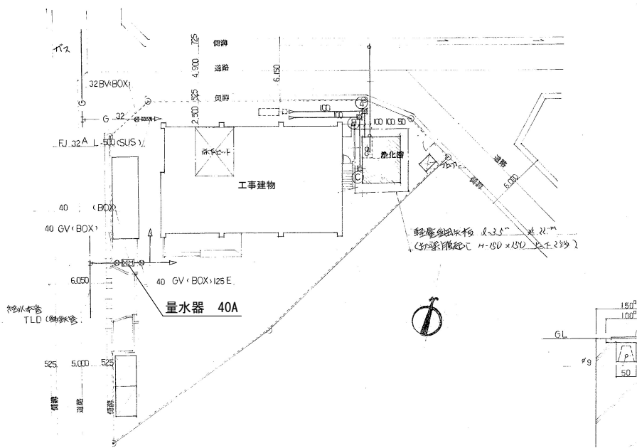
全体図 N.S.
