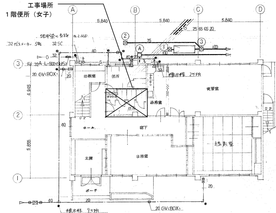
1階平面図 1:150
