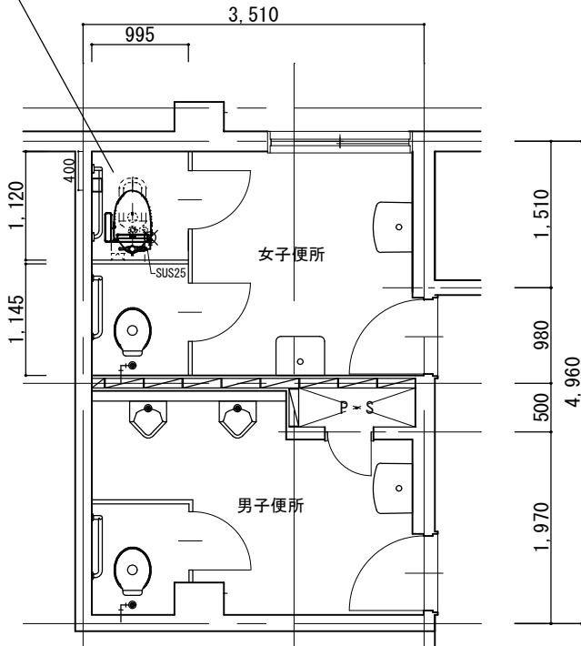
改修後 便所平面詳細図 1:50
