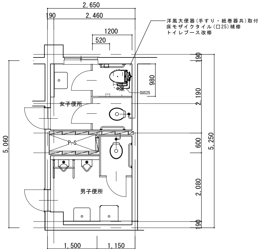
改修後 便所平面詳細図 1:50
