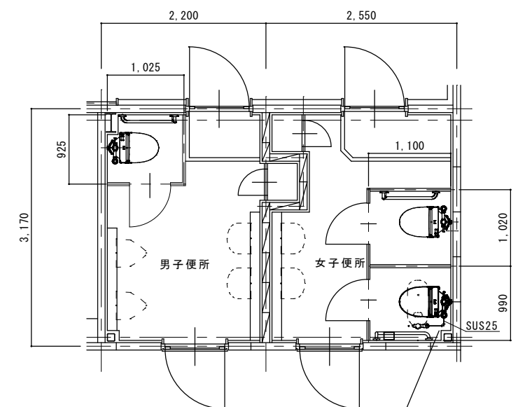
洋風大便器(手すり・紙巻器共)取付 床モザイクタイル(□25)補修
