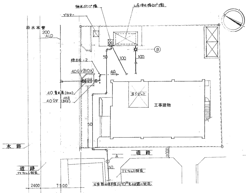
全体図 N.S.
