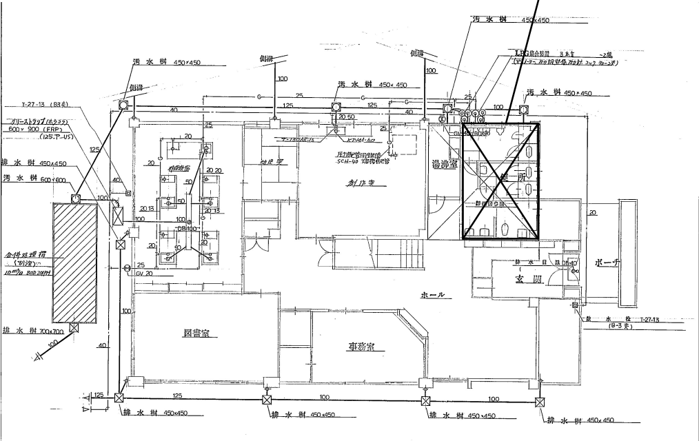
1 階平面図 1:200
