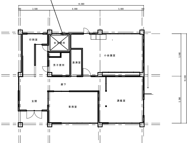
1階平面図 1:150
