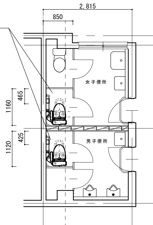
改修後 便所平面詳細図 1:50
