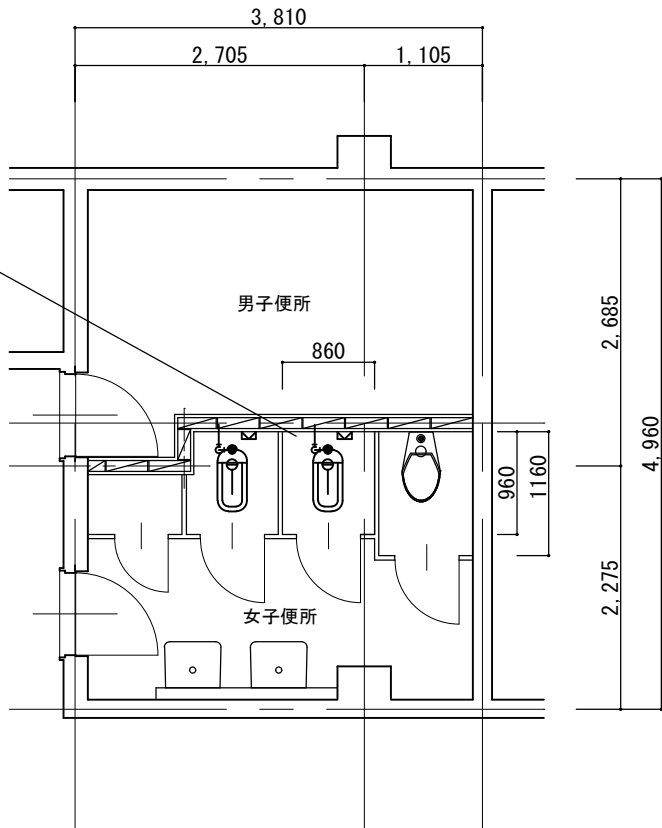
改修前 便所平面詳細図 1:50
