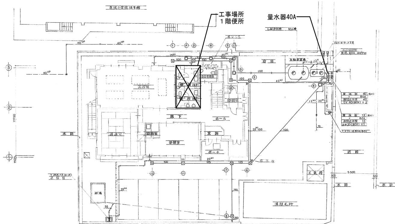
1階平面図 1:200
