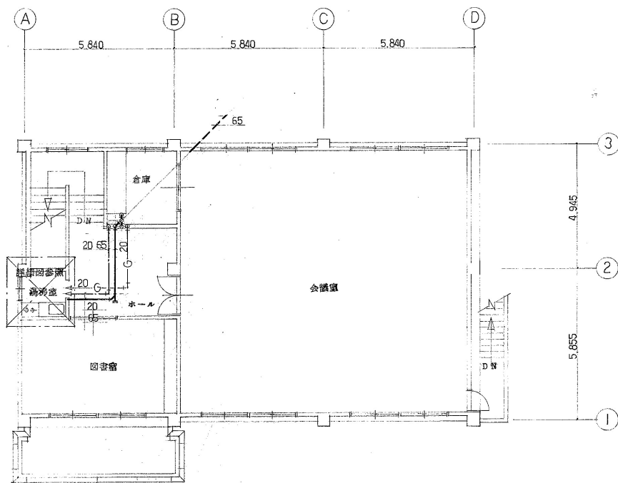
2階平面図 1:150
