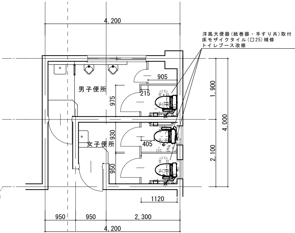
改修後 便所平面詳細図 1:50
