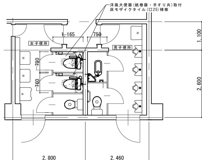
改修後
