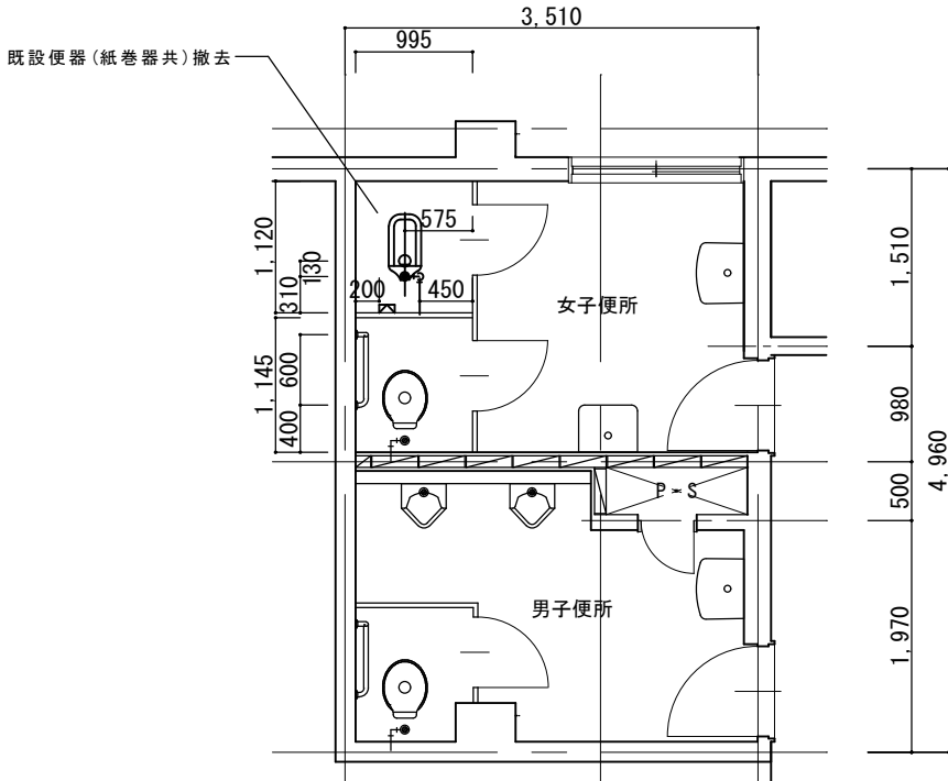
改修前 便所平面詳細図 1:50
