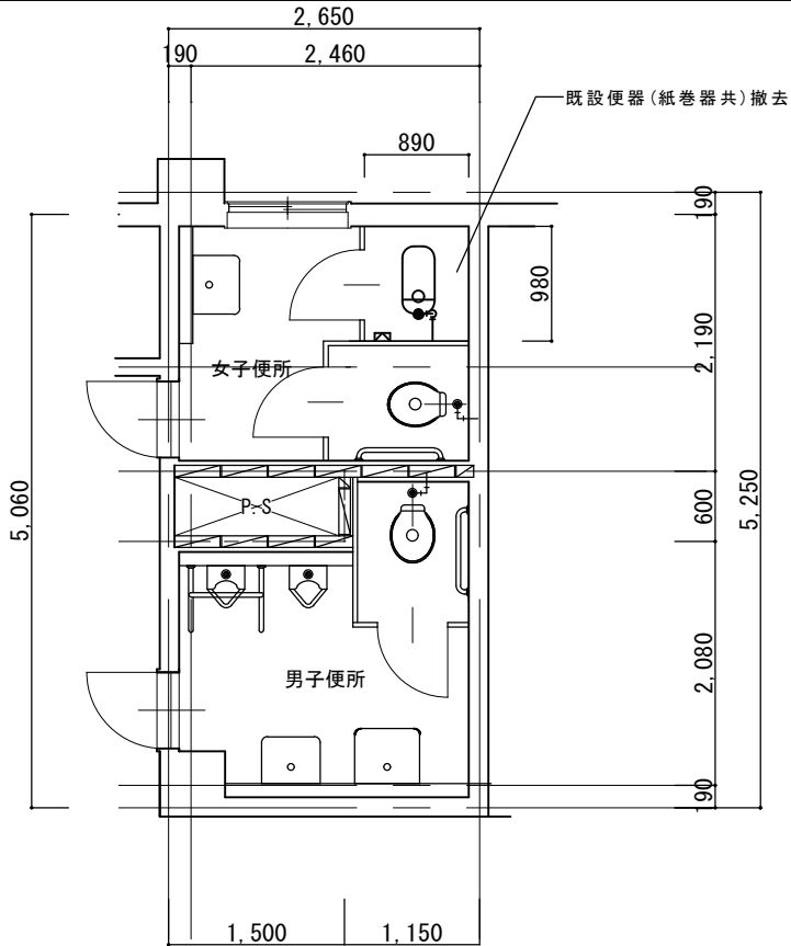
改修前 便所平面詳細図 1:50
