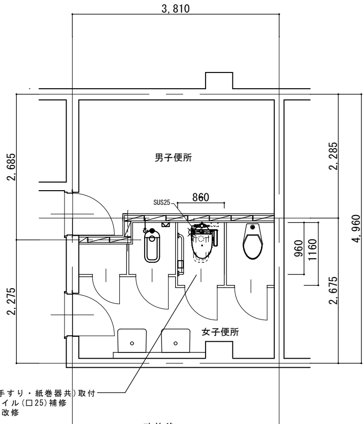
改修後 便所平面詳細図 1:50
