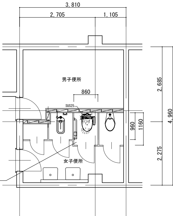
改修後 便所平面詳細図 1:50
