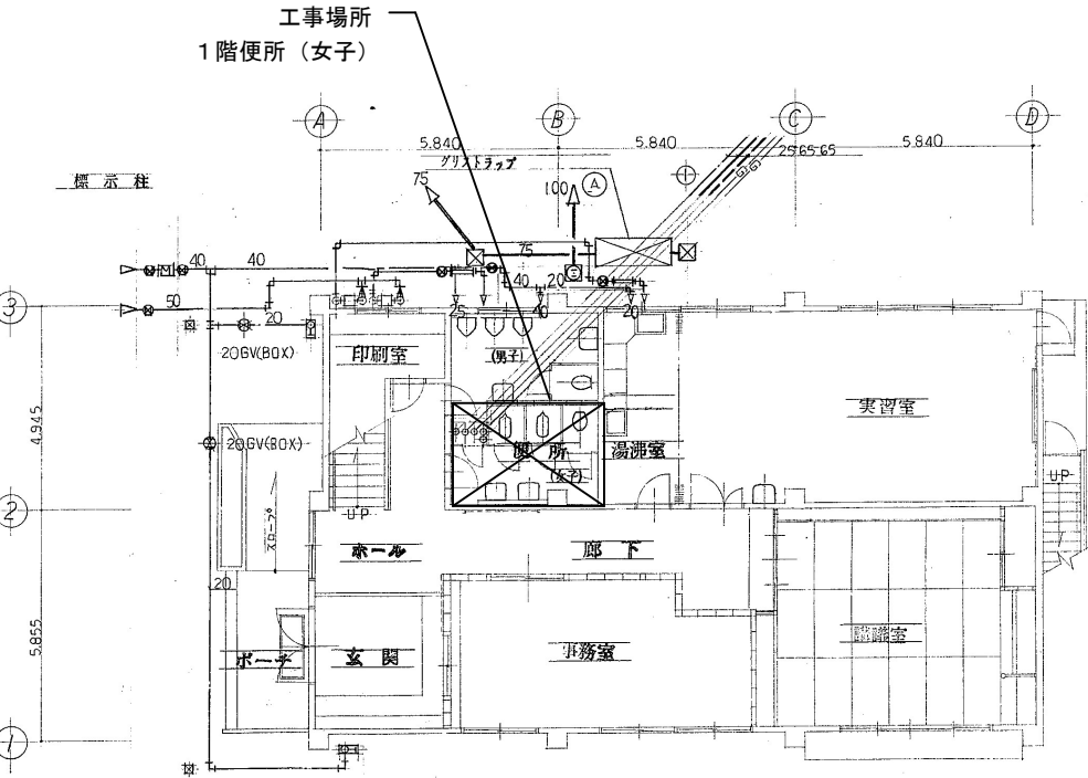
1階平面図 1:150
