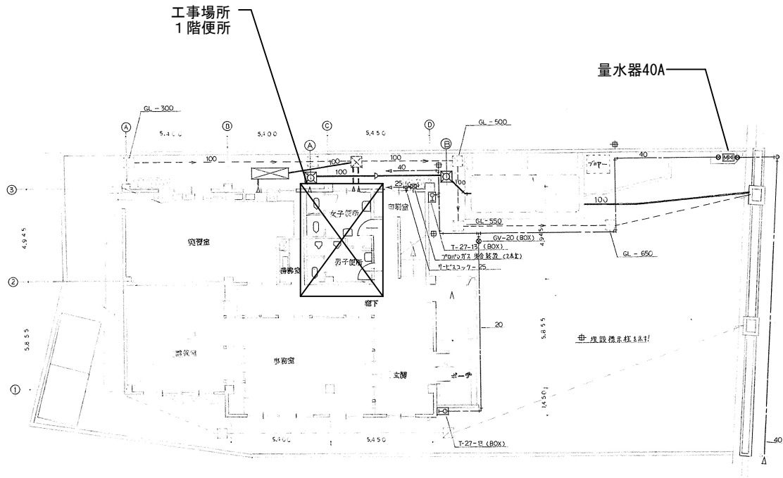
1階平面図 1:200
