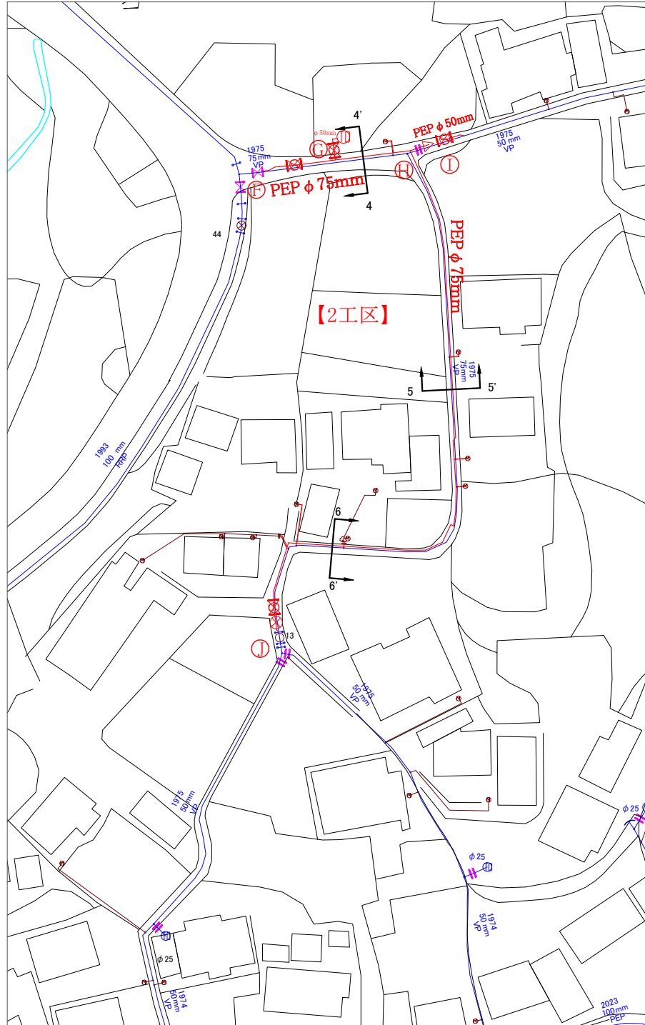
平面図 (2) S=1/500
