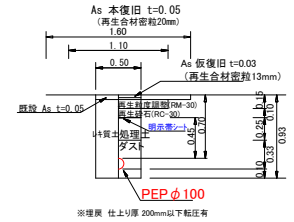
PEP φ 100土工図①
