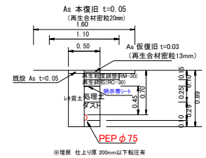
PEP φ 75土工図③
