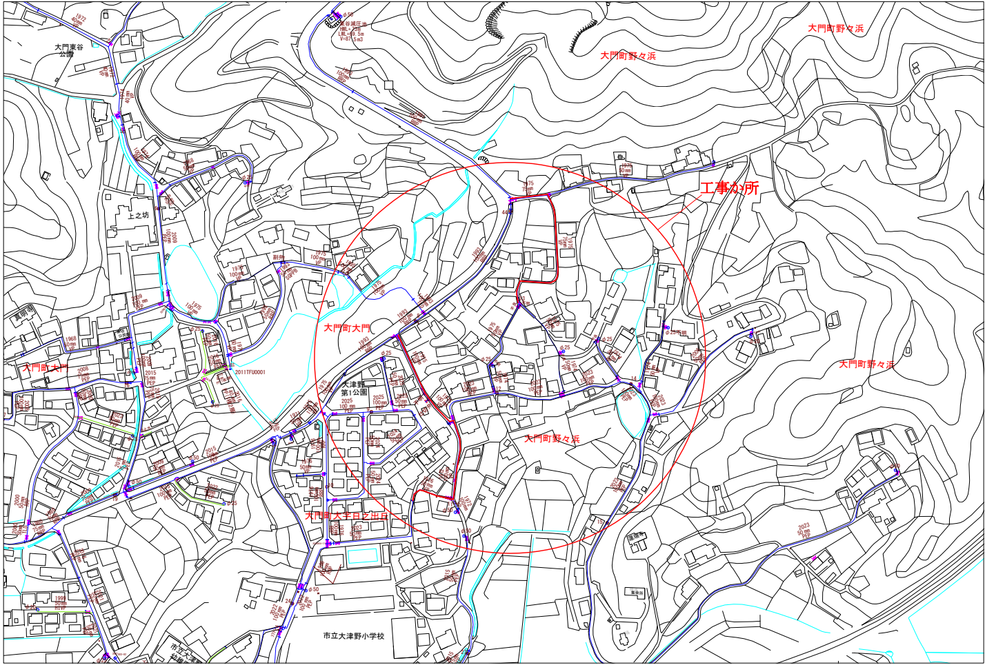
配管図 S=1/2500
