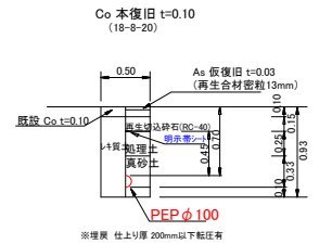
PEP φ 100土工図②
