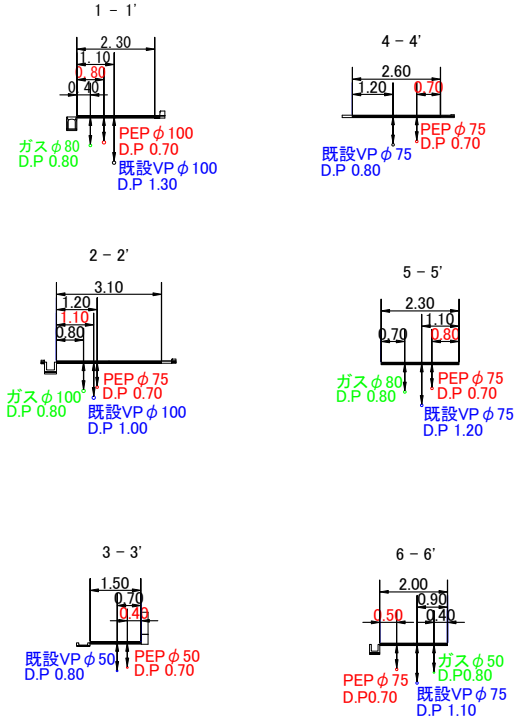
横断面図 S=1/100
