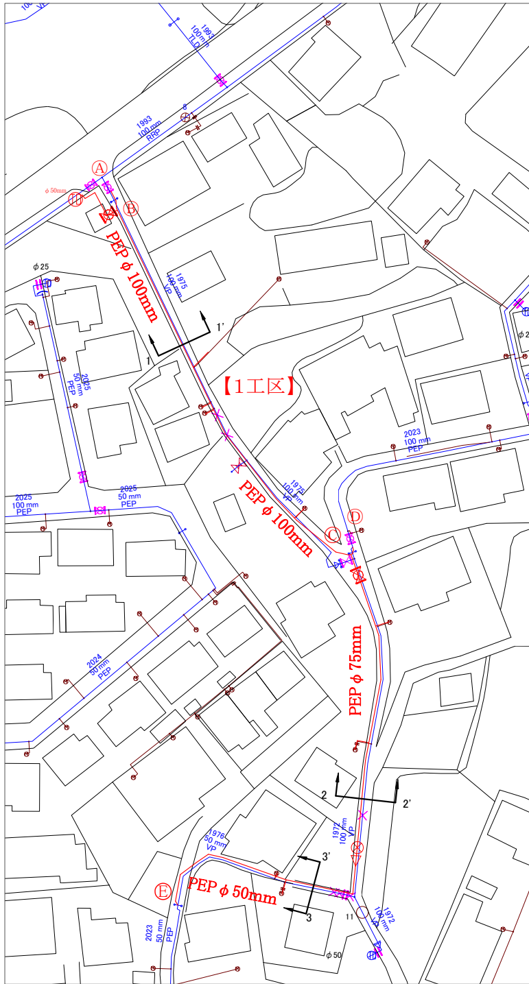
平面図 (1) S=1/500
