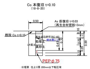
PEP φ 75土工図④
