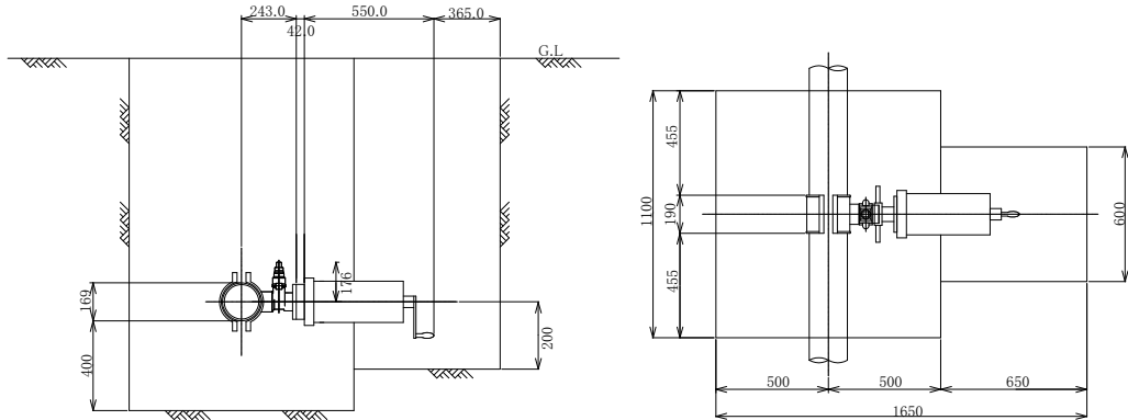
【参考】不断水分岐土工図150×50 S=Non
