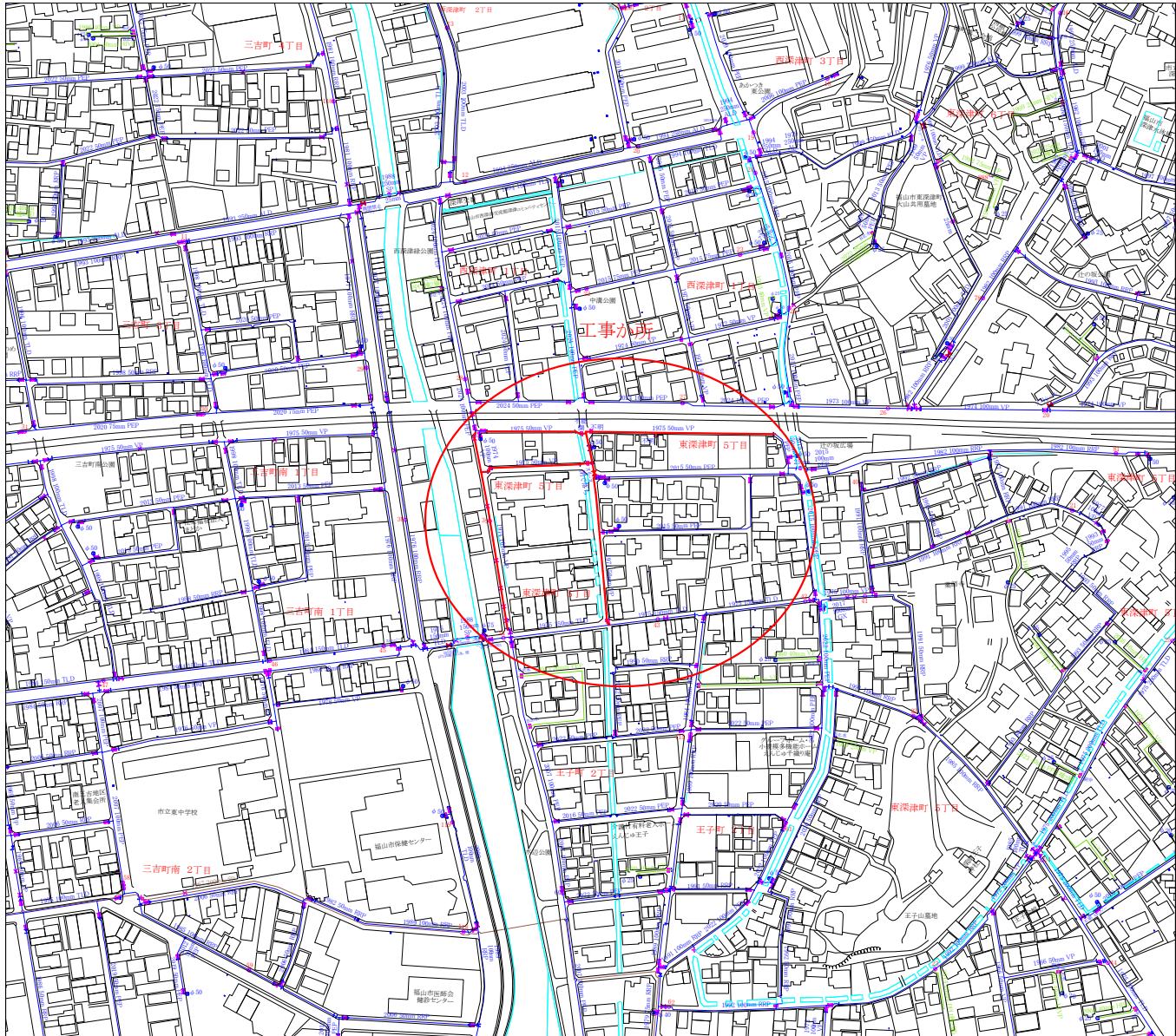
配管図 S=1/2,500
