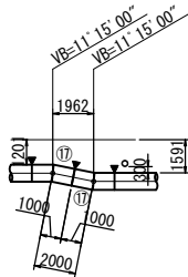
“o”部詳細図
