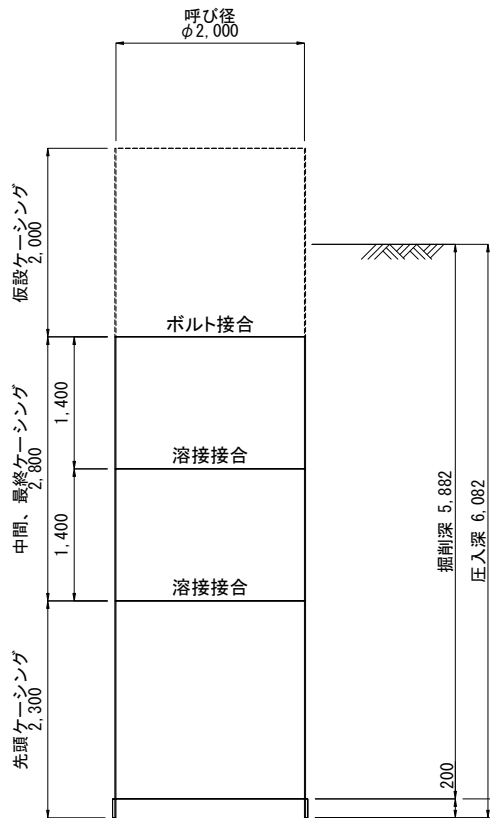
A-A断面 圧入掘削時
