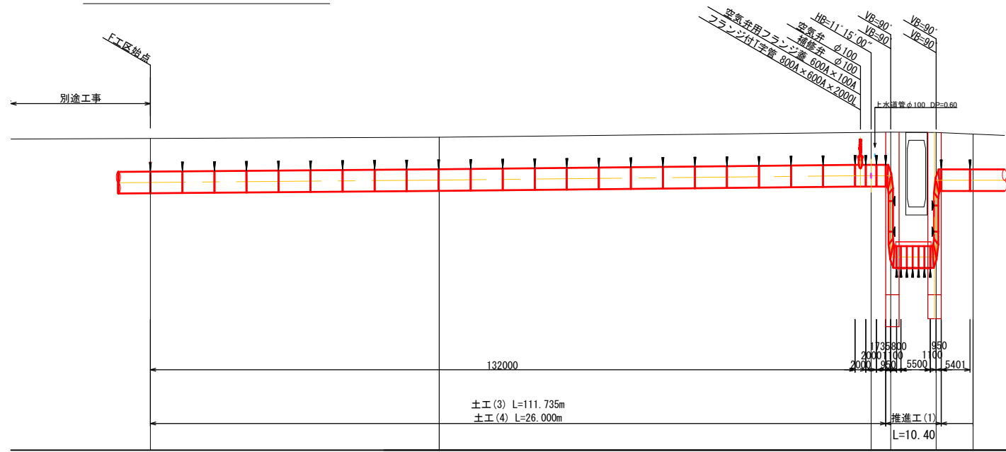
縦断図(1) / V=1:100 H=1:500
