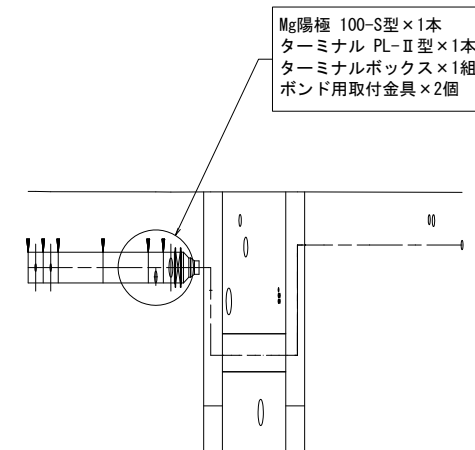
縦断図(3) V=1:100 H=1:500
