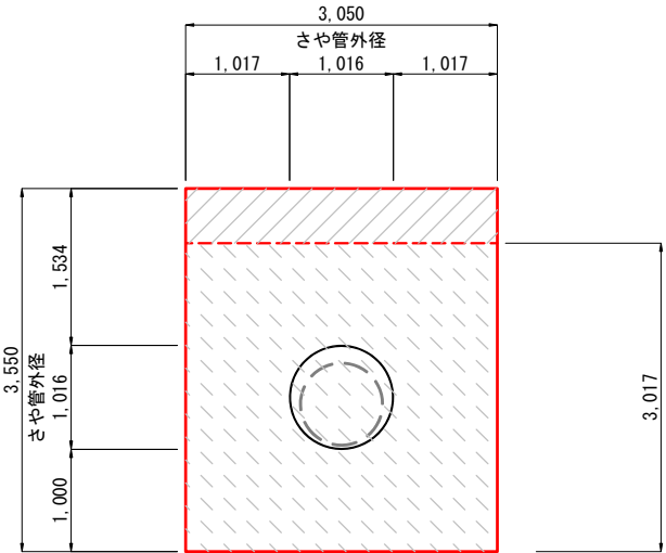
B-B断面図
