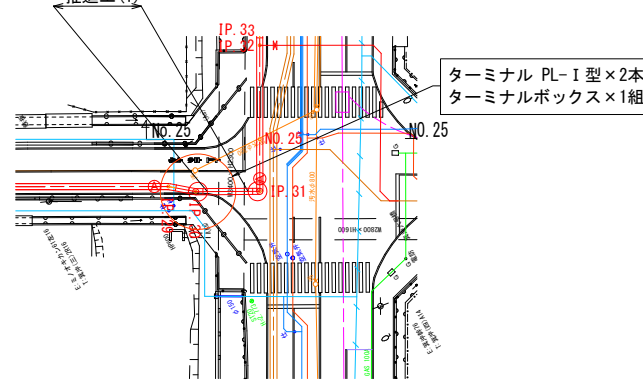
縦断図(2) V=1:100 H=1:500
