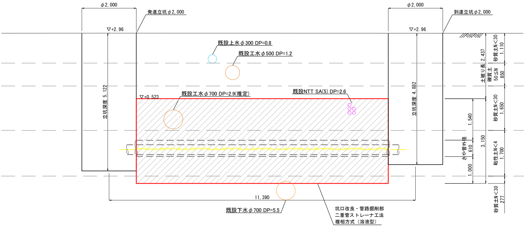
A-A断面図
