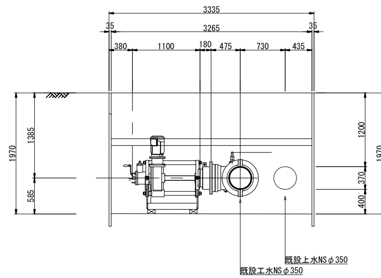
B-B 断面图
