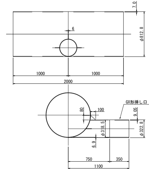
メカ挿し付排水T字管
