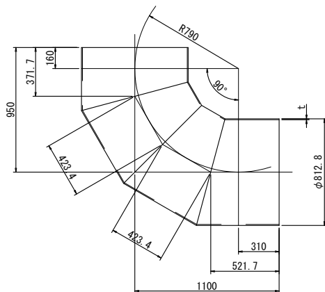
90° 曲管
