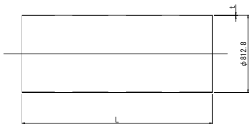
短管
