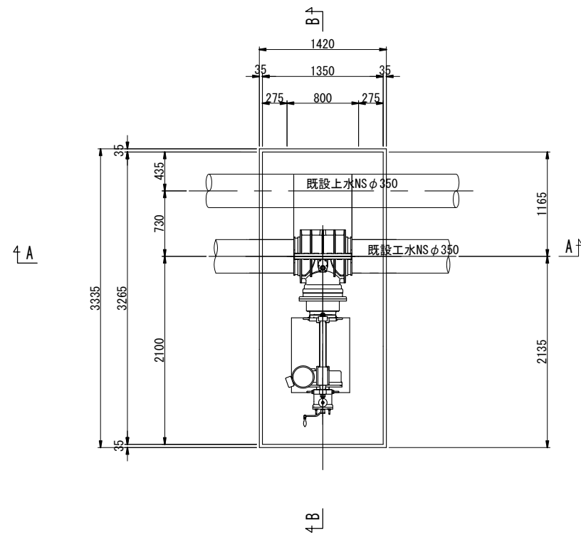
平面图
