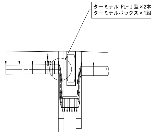
管割詳細図(2) S=1/200
