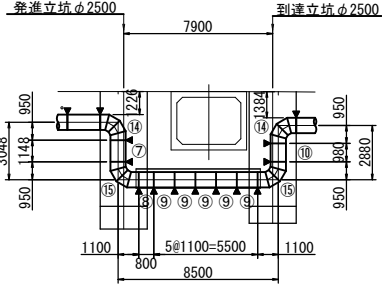
“n”部詳細図
