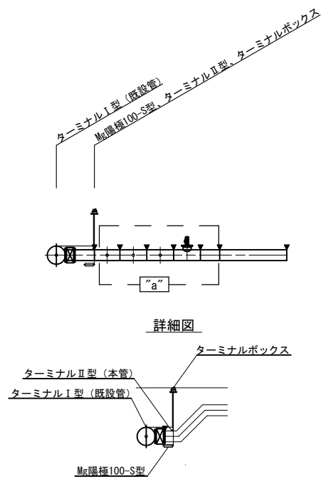
管割詳細図(1) S=1/200
