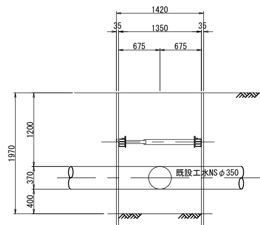
A-A 断面図
