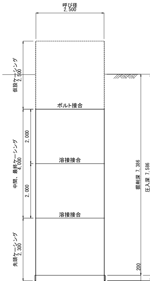
A-A断面 圧入掘削時
