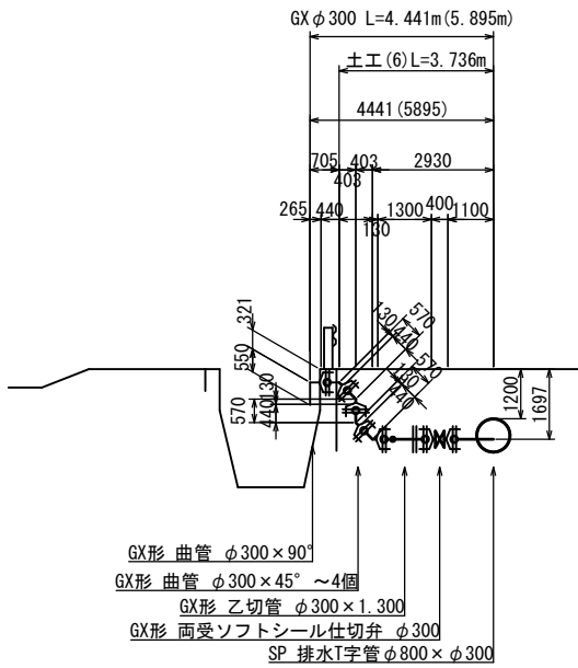
新設排泥管詳細図
