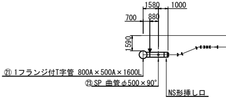
工業用水道連絡管②
