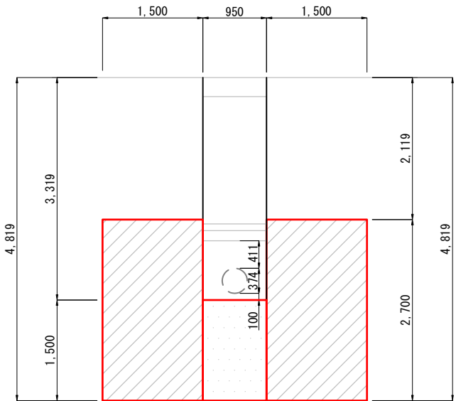
B-B断面図
