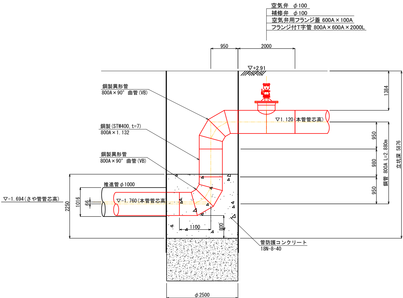
B-B断面図
