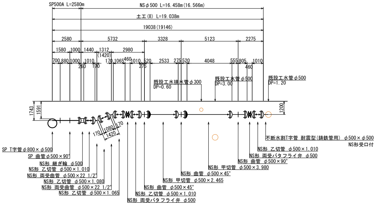
新設工業用水連絡管-2
