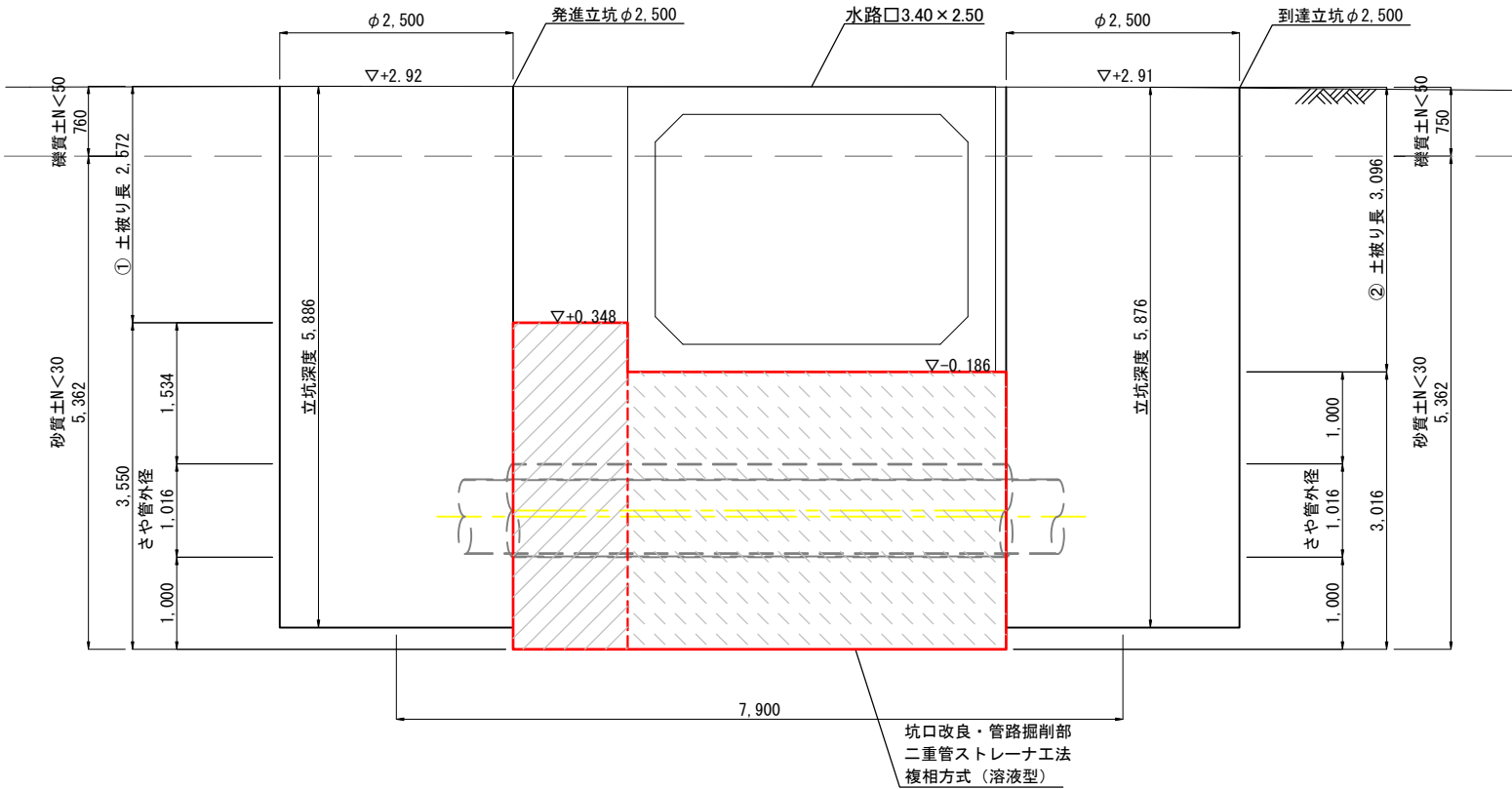
A-A断面図
