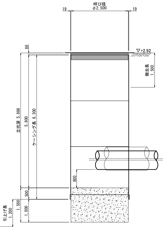
A-A断面 引上げ完了時
