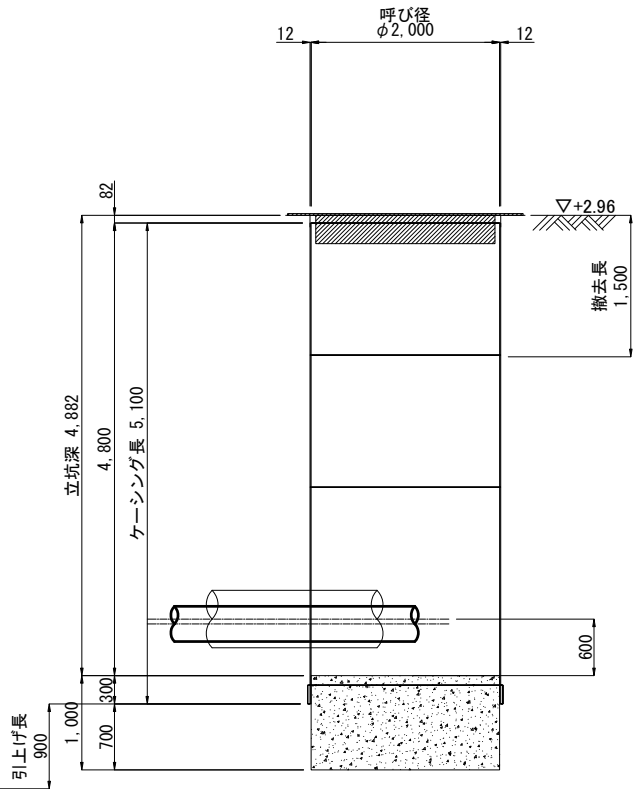
A-A断面 引上げ完了時
