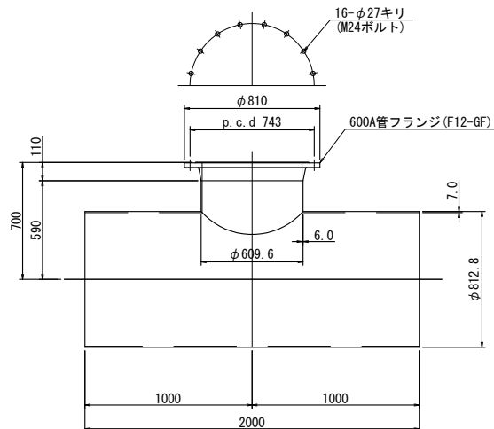
フランジ付T字管
