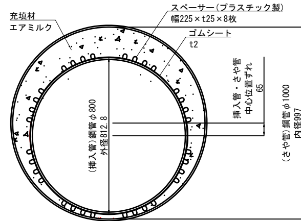
挿入管断面図 S=1/10
