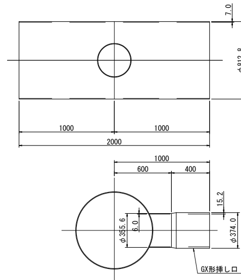
メカ挿し付T字管
