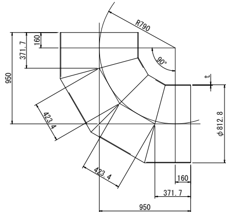
90° 曲管
