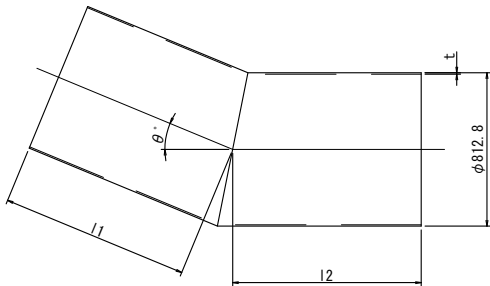
θ° 曲管
