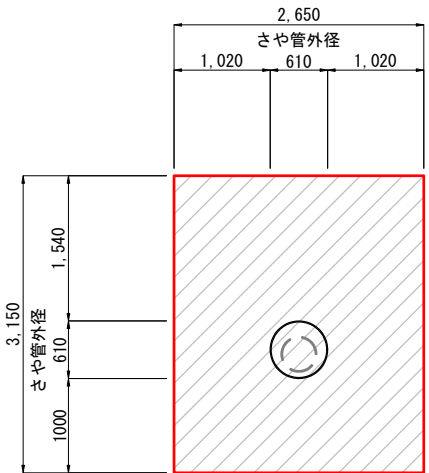
B-B断面図
