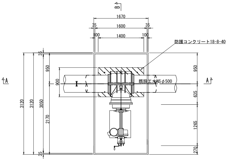
平面図
