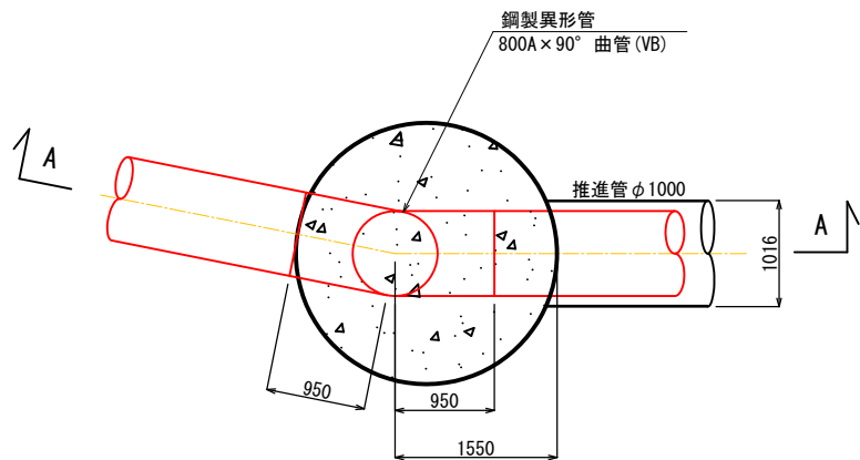
A-A断面図
