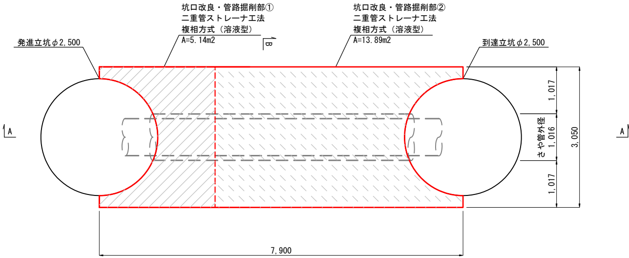
平面図
