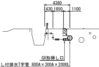
排泥管②配管図
