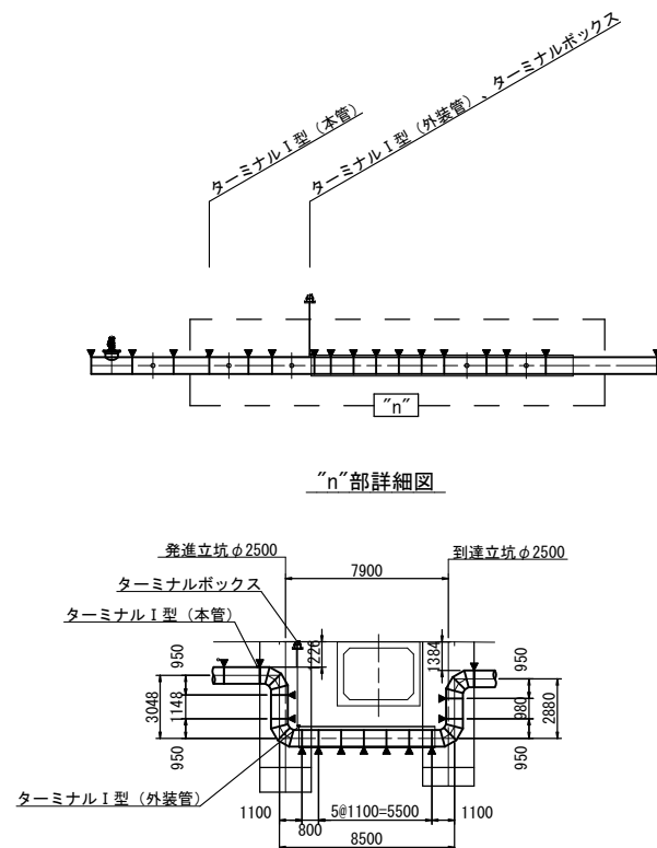
管割詳細図(2) S=1/200
