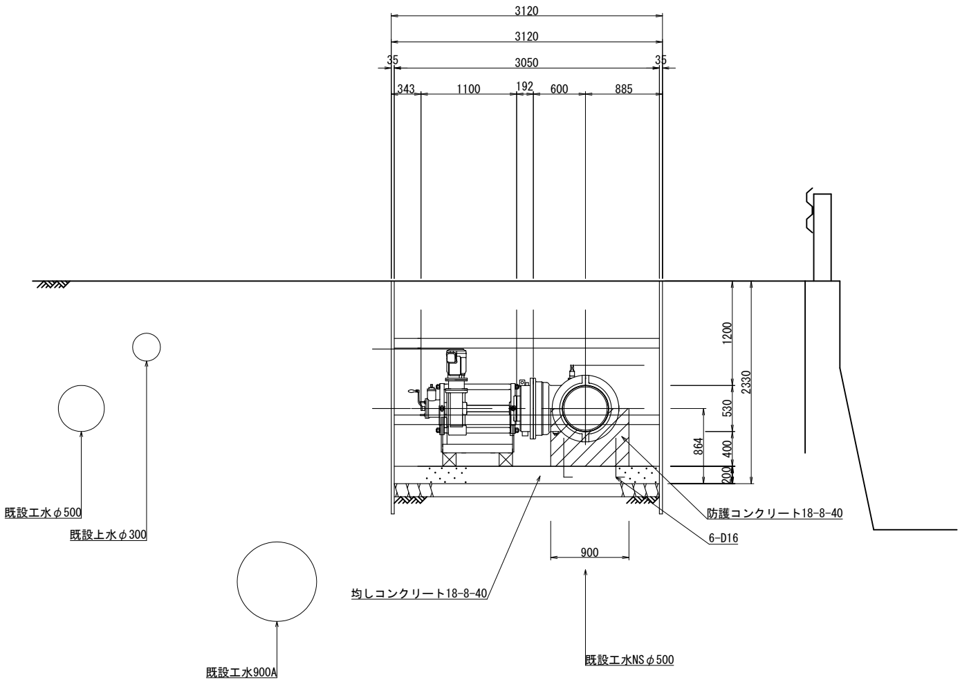
B-B 断面図
