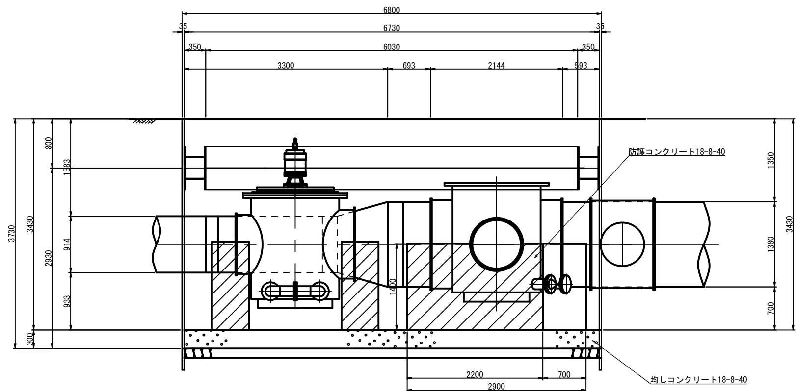
A-A 断面図
