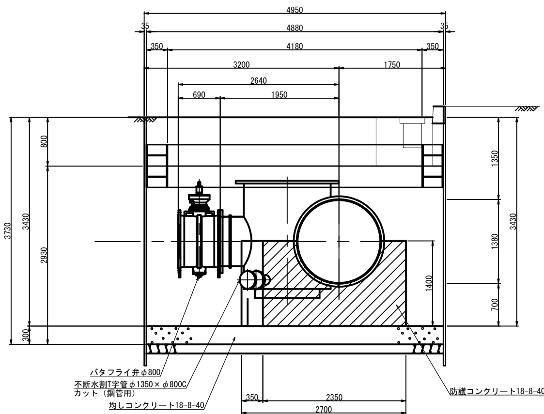
B-B 断面図
