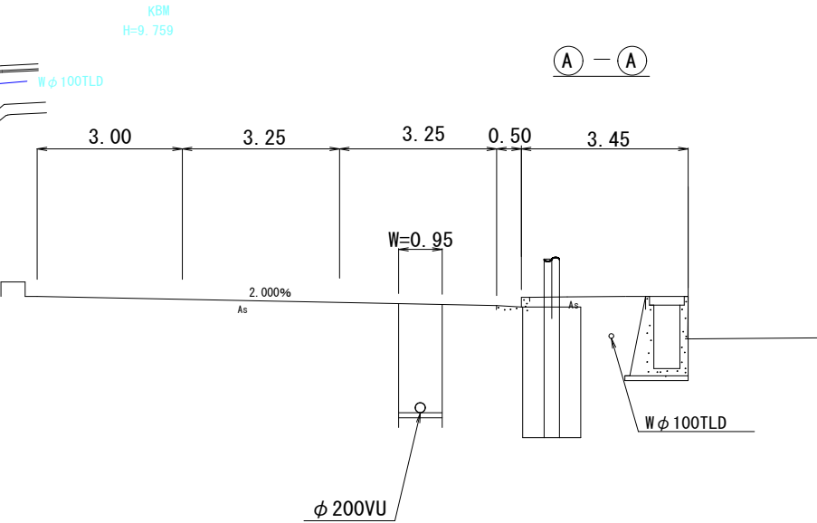
標準横断面図 S=1/100
