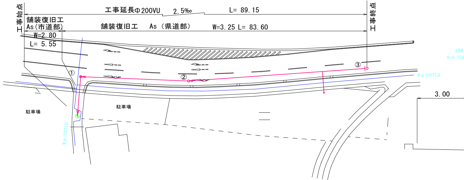
管渠埋設平面図 S=1/500
