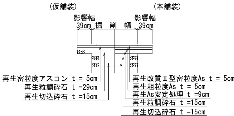
舗装断面図 S=1/10
