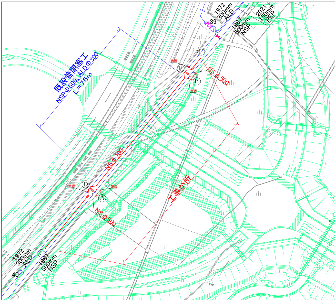
平面図 S=1/500
