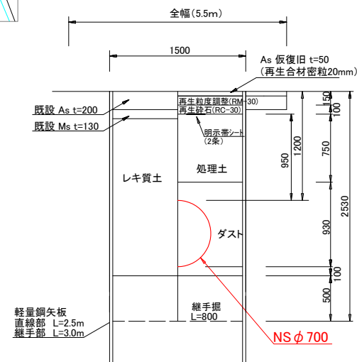
標準横断面図 S=1/100
