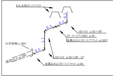
K形管帽部ドレン詳細図(D,E付近)
