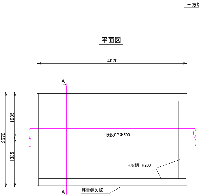
仮設工標準図 S=non (参考図)
