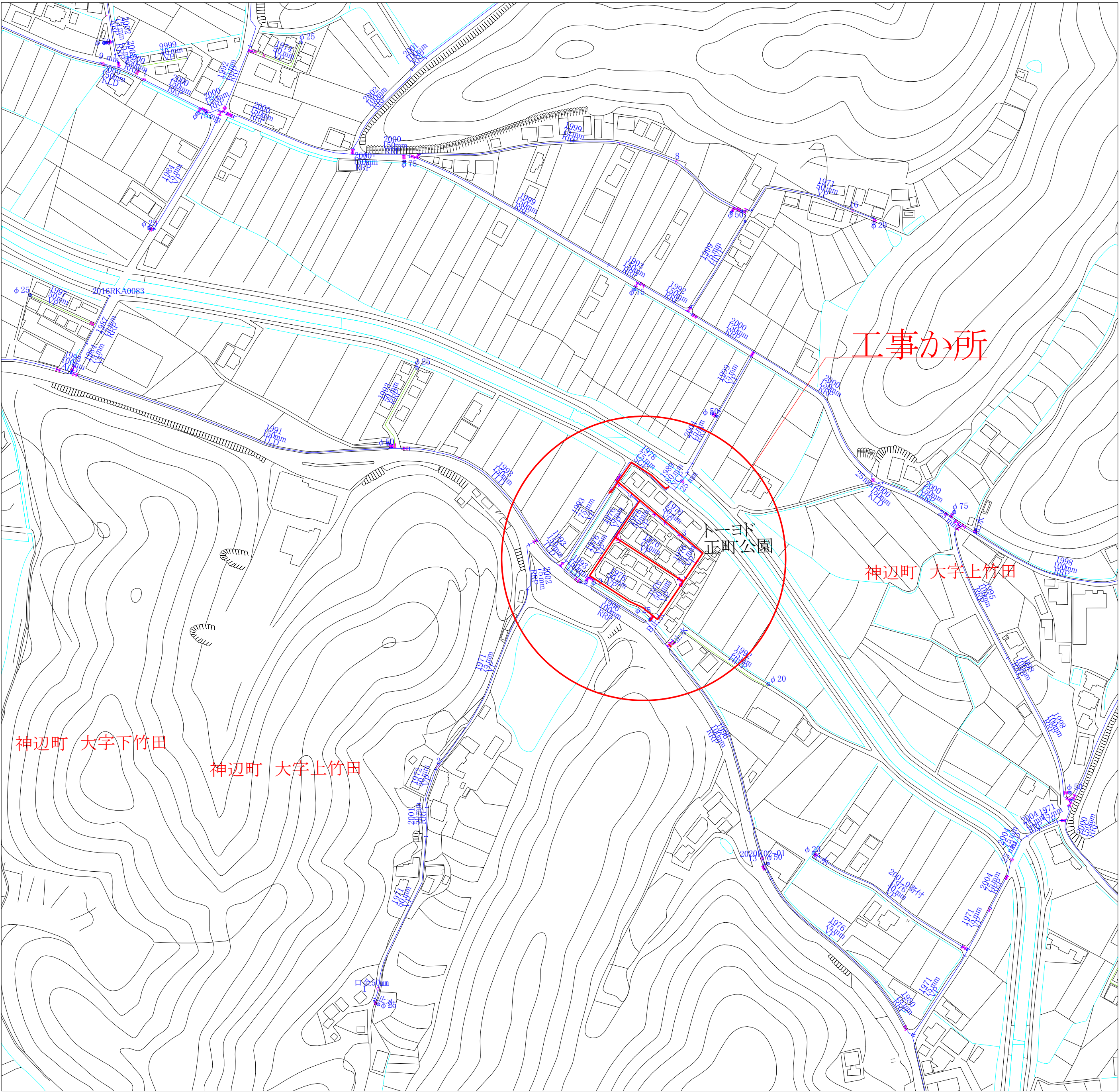
配管図 S=1/2,500
