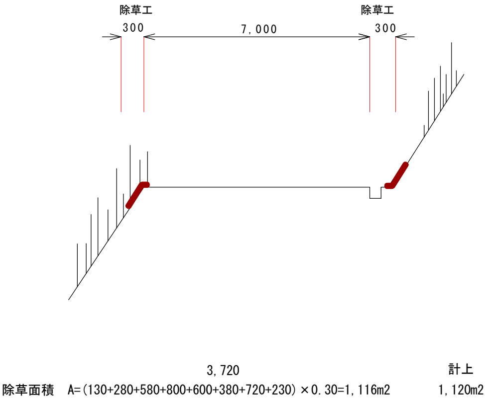
標準横断面図 S=1/100
