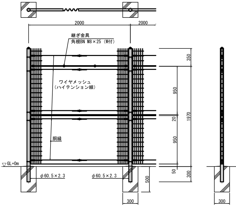
メッシュフェンス(H=2000)参考図 AT : S=1:20
