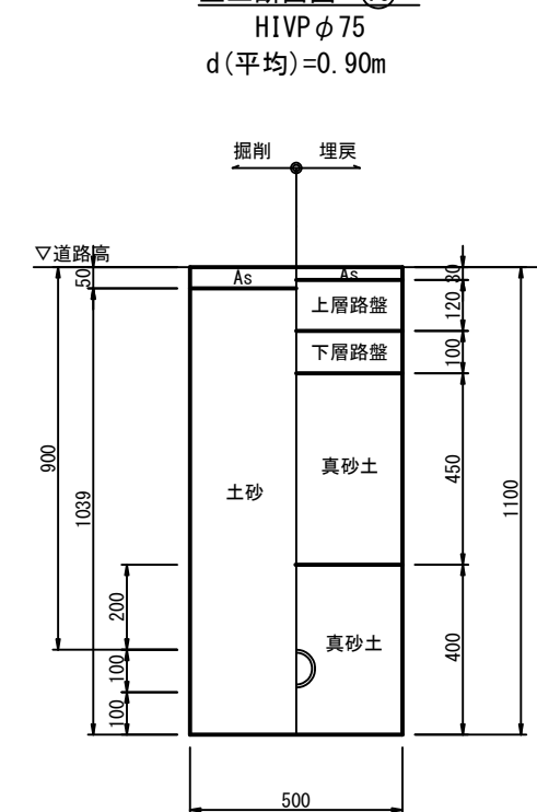
土工断面図 ⑩
