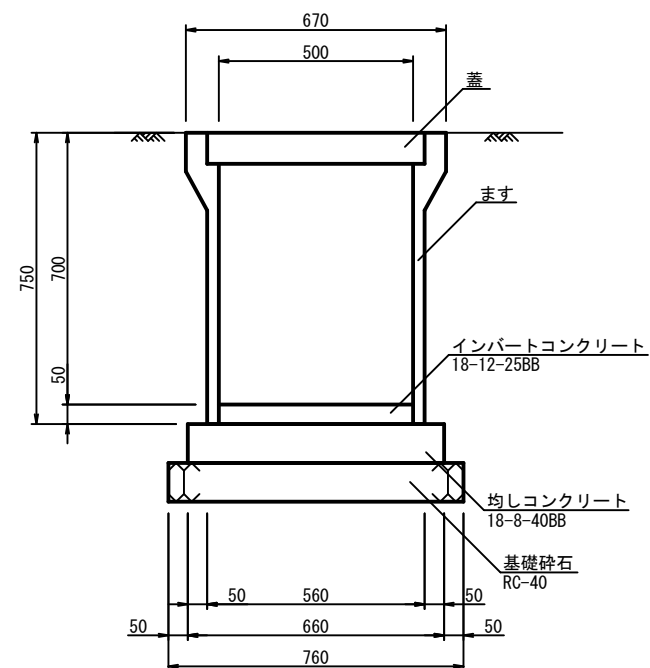
プレキャストます CB-S500
