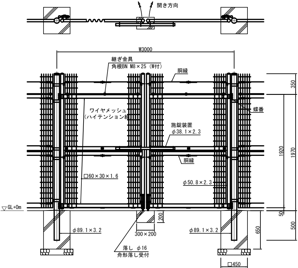
両開き門扉(W=3000 H=2000)参考図 AT : S=1:20
