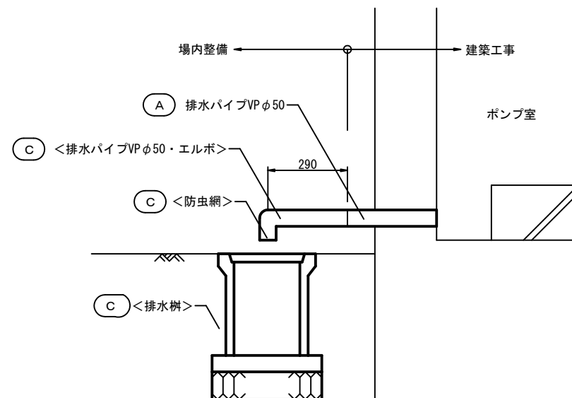
ポンプ所排水詳細図
