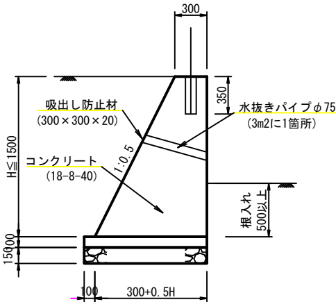
小型重力式擁壁 タイプⅡ-①
