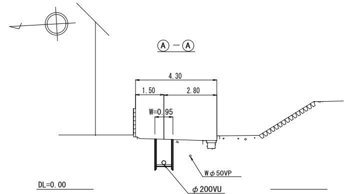
標準横断面図 S=1/100
