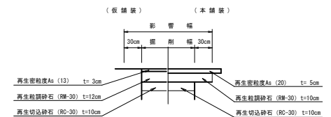
舗装復旧断面図 S=1/30
