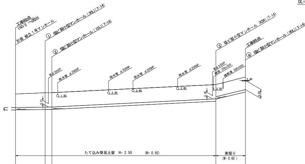
管渠埋設縦断面図 S = 縦1/100 横1/500
